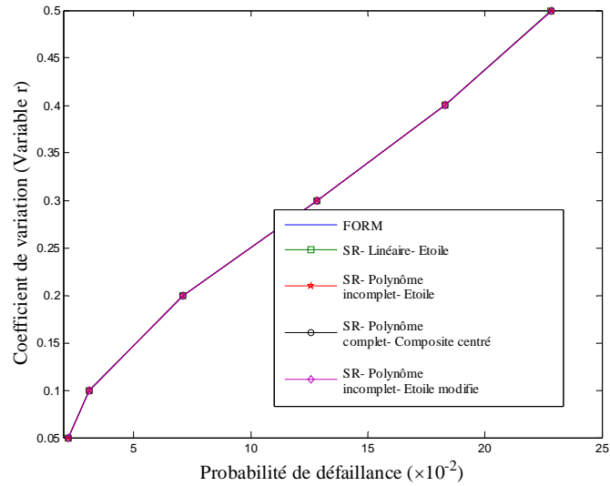
Figure A.7. Evolution de la probabilité de défaillance en fonction du coefficient de variation de variable n° 4 ( r )
