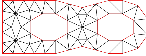
Fig. 1.8. Maillage initial.
