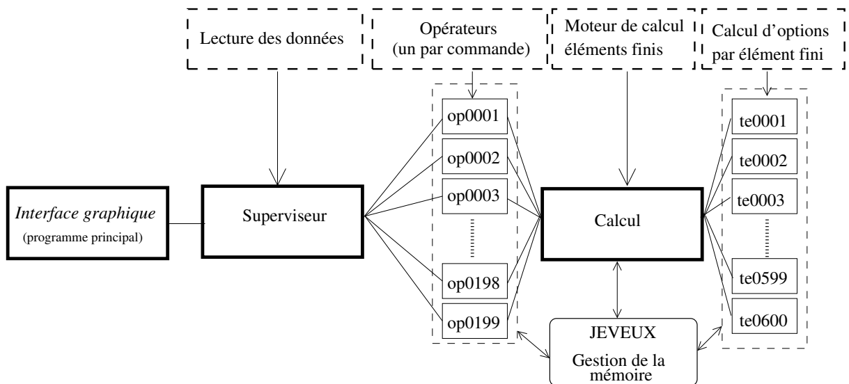
Fig. 1.5. Architecture informatique globale de Code_Aster .
