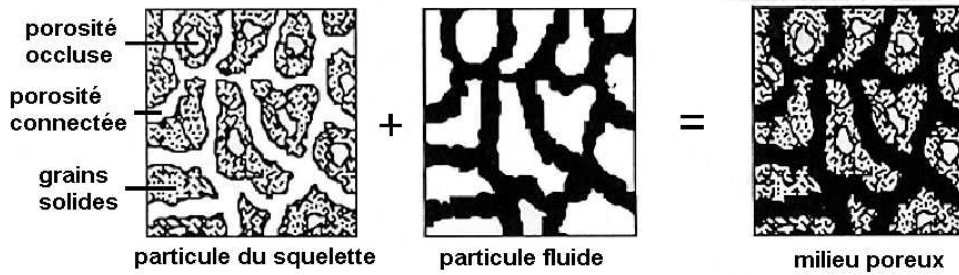
Fig. 1.1. Le milieu poreux vu comme une superposition de deux milieux continus : le squelette solide et la phase fluide.
