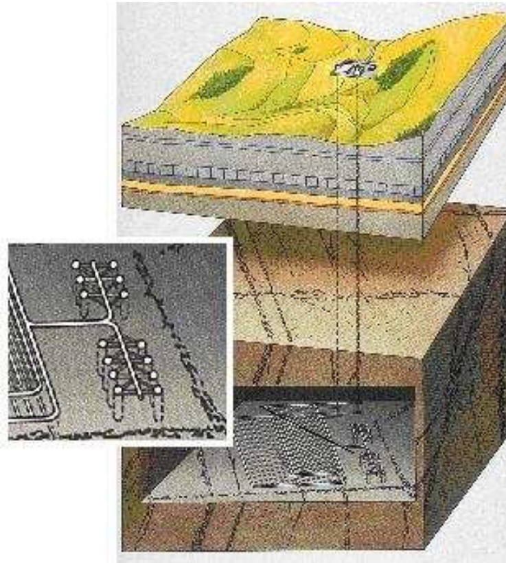
Fig. 1.2. Ouvrage de stockage souterrain dans son ensemble.
