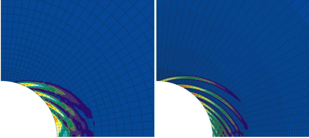
Fig. 1.7. Zones de fissuration dans un calcul d'excavation : à gauche, calcul sur un maillage grossier ; à droite, calcul sur un maillage raffiné autour de la zone d'excavation.
