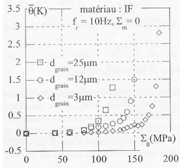
FIG. 5.20 – Courbes d'échauffement obtenues pour différents aciers ferritiques se différenciant de par la taille moyenne des grains [Dou04].
