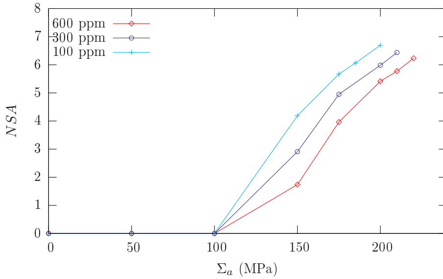
FIG. 5.49 – Evolution du nombre moyen de systèmes de glissement actifs par grain calculées pour différentes fractions volumiques de précipités non-cisillables de rayon constant.
