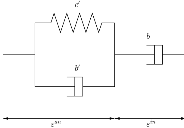
FIG. 4.13 – Schema d'un élément rhéologique de Kelvin-Voigt associé à un amortisseur visqueux.
