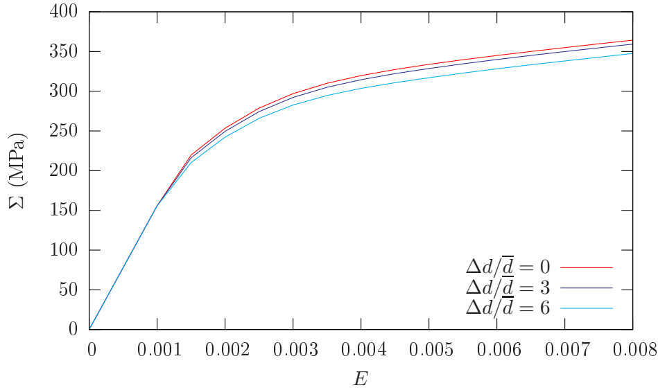
FIG. 5.27 – Courbes de comportement en traction uniaxiale obtenues par le modèle pour différentes distributions de la taille de grain ayant la même valeur moyenne.
