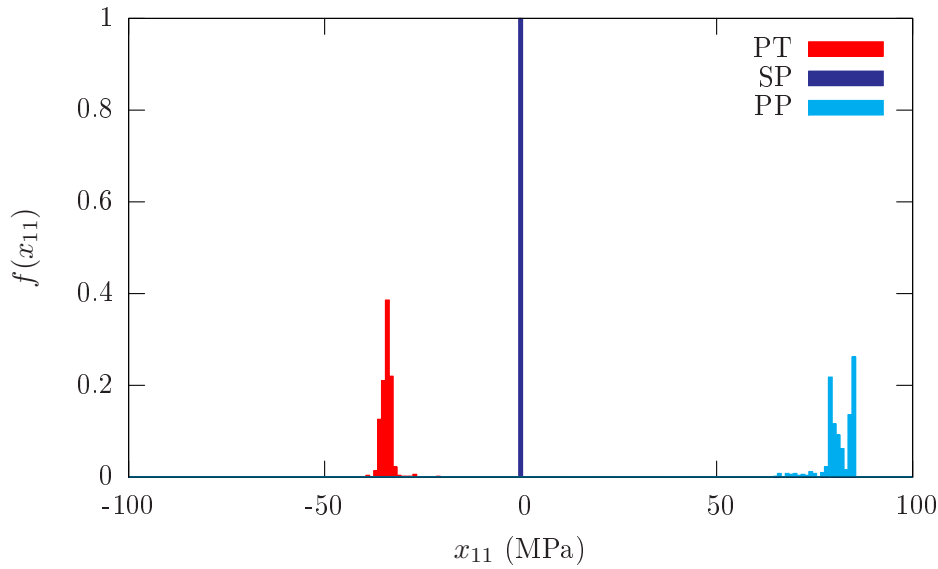
FIG. 5.45 – Fonctions de densités associées à la composante 11 de la variable d'écrouissage cinématique locale x calculées à l'aide du modèle après prédéformations de 10% transverse (PT) ou parallèle (PP) à la direction du chargement cyclique ou sans prédéformation (SP).
