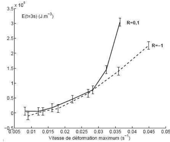
FIG. 3.12 – Energie dissipée en fonction de la vitesse de déformation maximale dans le cas d'un acier laminé pour deux rapports de charge différents [Maq06].
