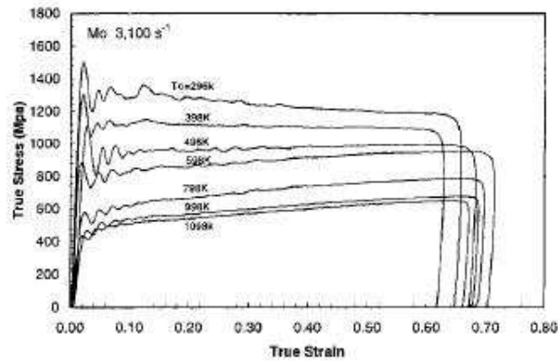
FIG. 3.2 – Courbes de comportement obtenues à différentes températures lors d'essais adiabatiques sur des polycristaux de molybdène [NNGL99].
