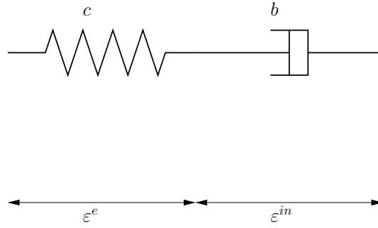
FIG. 4.8 – Schéma d'un élément rhéologique de Maxwell.
