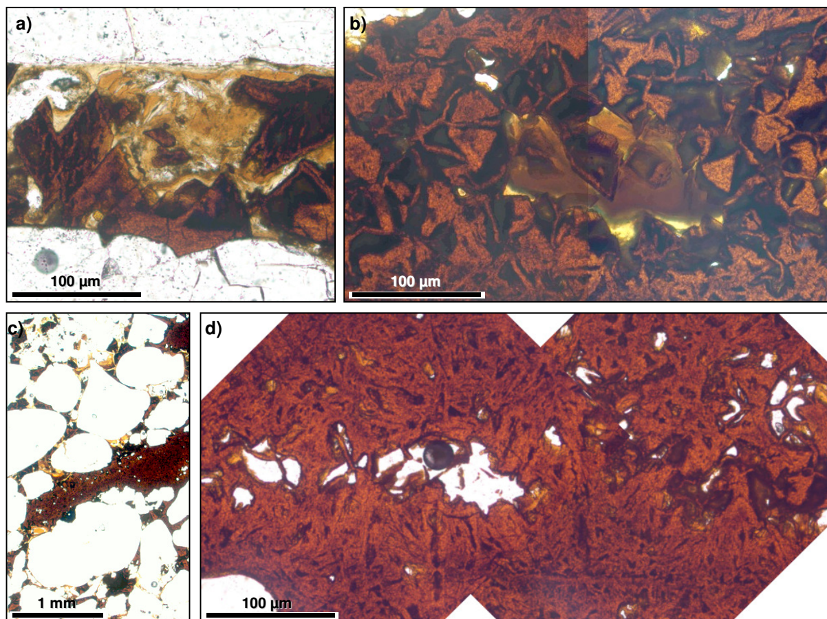
Figure 84 - Oxydes de fer (goethite) en pseudomorphose de rhomboédres (Les Chézeaux, Santranges, 18). Lumière polarisée. a) Dans l'espace poral entre les grains de quartz ; b) Enchevêtrement de rhomboédres dans un "filonet" d'oxydes dépourvu de grains détritiques. c) Grès grossier à grains ronds et passages (lentilles) d'oxydes fer dépourvus de grains de quartz, également illuviations argileuses (jaunes) dans les pores. d) Détail de c : ciment d'oxydes de fer dans des structures dépourvues de grains de quartz. La géométrie des cloisons ferrugineuses évoque des croissances cristallines sous forme de lattes (plaquettes), mais des géométries compatibles avec des rhomboédres sont également possibles. Il faut noter, la présence d'une morphologie arrondie qui est éventuellement d'origine biologique (fossile).
