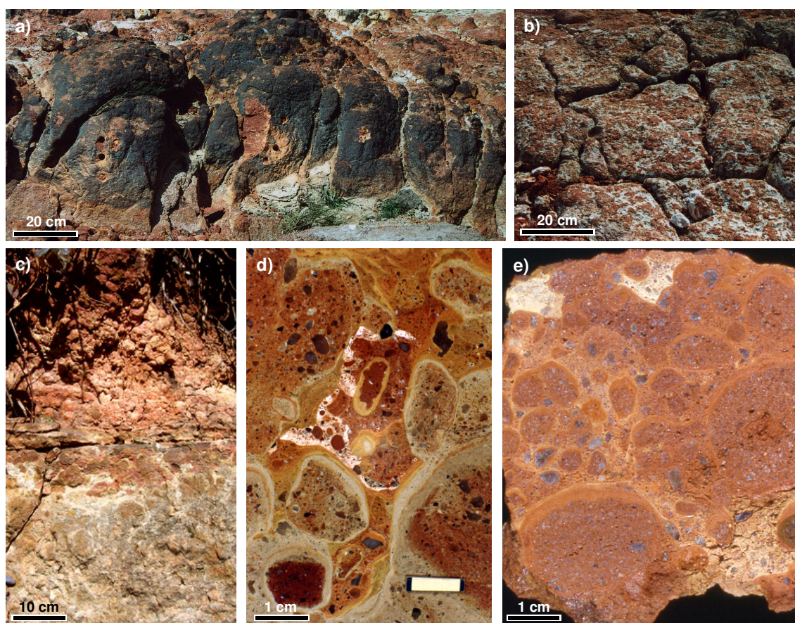
Figure 24 - Aspect colonnaire des niveaux gréseux. Les niveaux gréseux présentent souvent un débit colonnaire résultant des transformations au sein d'un sol avec fentes verticales plus pédoturées que le corps des colonnes et structures de coiffe au sommet des colonnes. a) Débit colonnaire du niveau de grès (Naussac, 48). Noter les points de prélèvement pour les mesures paléomagnétiques. La patine noire des grès est acquise en milieu immergé. b) Débit colonnaire vue par le dessus. Niveau gréseux fortement bioturbé par des terriers de termites et blanchi (Naussac, 48). c) Aspect nodulaire des faciès colonnaires sommitaux (Passat, Saint Victor, 03). d) Faciès nodulaire avec grandes illuviations de matériaux fins en base des vides et en coiffe dans les nodules (Le Bouchet, Olby, 63). e) Faciès nodulaires similaires avec extension des illuviations jusqu'à former des raies qui "enveloppent" plusieurs nodules (Naussac, 48).
