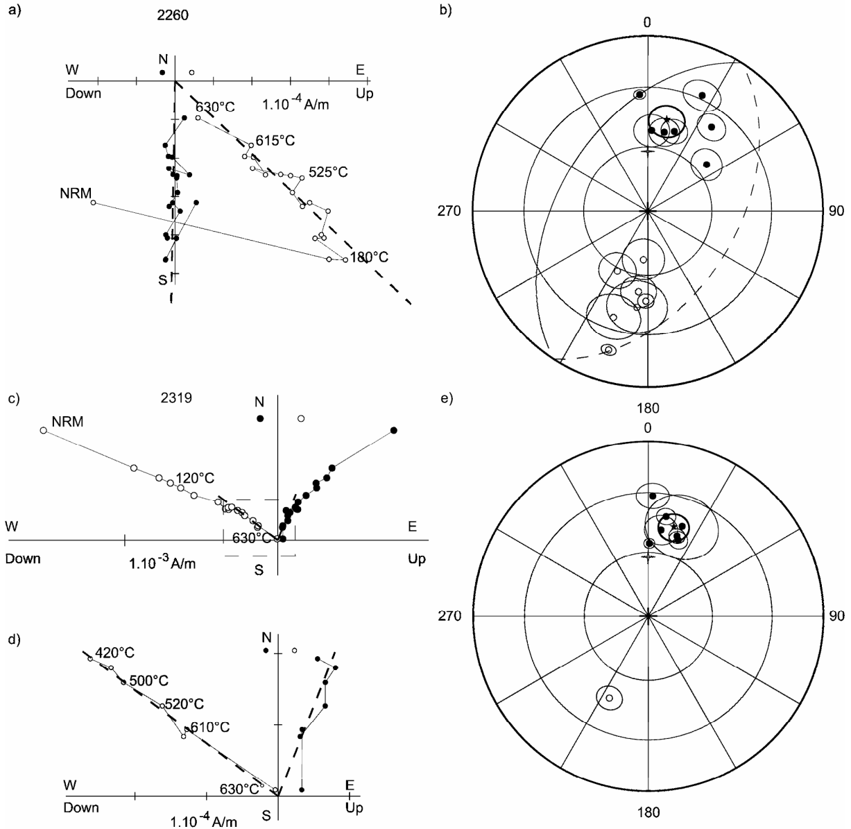
Figure 35 - Désaimantation de l'aimantation rémanente naturelle (ARN) et directions d'aimantation haute température (ARHt) pour les sites de Naussac-1 et de Naussac-2. a) Projection orthogonale du vecteur aimantation au cours de la désaimantation thermique pour un échantillon représentatif du site de Naussac-1. b) Projection à aires conservées des directions d'ARHt et de leur moyenne pour le site de Naussac-1. c) Projection orthogonale du vecteur aimantation au cours de la désaimantation thermique pour un échantillon représentatif du site de Naussac-2. d) Zoom sur la fin de la désaimantation ; e) Projection à aires conservées des directions d'ARHt et de leur moyenne pour le site de Naussac-2. Symboles noirs/ blancs : le vecteur aimantation pointe vers le bas/haut, les directions sont normales/ inverses. Etoile: moyenne des directions d'ARHt. Croix grise : direction du champ dipôle actuel.
