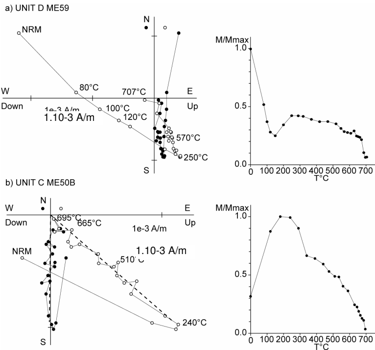
Figure 17 - Diagrammes de Zijderveld représentatifs pour deux échantillons représentatifs des Mottes. La plupart de l'aimantation est portée par l'hématite (désaimantation entre 580°C et 680°C). Il existe une aimantation détruite à basse température dont la direction est proche du champ dipôle actuel.
