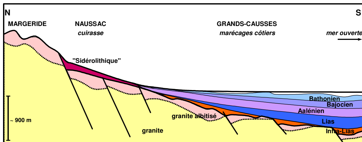
Figure 107 – Coupe schématique à travers le Ssud du Massif central au Dogger. La couverture sédimentaire se réduit sur le socle et se raccorde aux paléaltérations datées du Jurassique supérieur/Crétacé inférieur. Des reliefs de socle dominaient vraisemblablement les paléaltérations.
