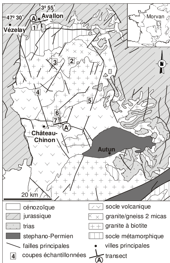
Figure 93 - Carte géologique simplifiée du Morvan et localisation des coupes échantillonnées pour le paléomagnétisme : 1-Avallon ; 2-Saint-Agnan ; 3-La Pérouse ; 4-Chapelle de Banquet ; 5-Moux-en-Morvan ; 6-Planchez ; 7-Château-Chinon. La coupe AA' est représentée sur la figure 95.
