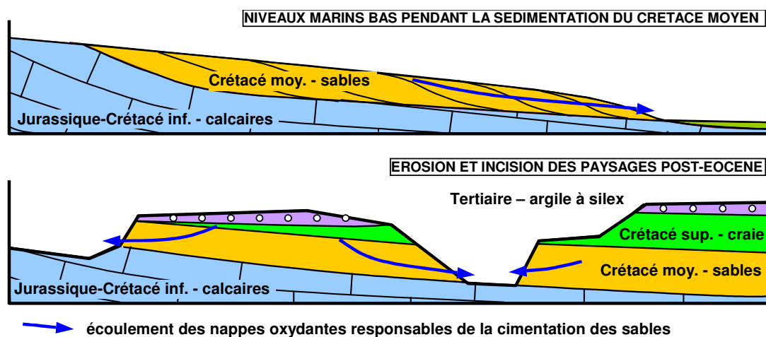
Figure 104– Schéma illustrant les deux hypothèses concernant la ferruginisation des sables du Crétacé inférieur de la bordure sud-est du bassin de Paris : altération précoce pendant le dépôt des sables lors de périodes d'abaissement du niveau eustatique ou altération tardive lors de l'évolution continentale cénozoïque et l'incision des paysages.
