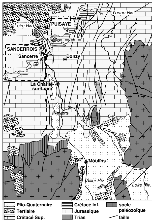
Figure 77 - Carte géologique de la bordure sud-est du bassin de Paris. Les formations étudiées se situent sur l'auréole de Crétacé inférieur du Sud du bassin de Paris. Les zones encadrées correspondent à la localisation des zones étudiées en Puisaye et en Sancerrois.
