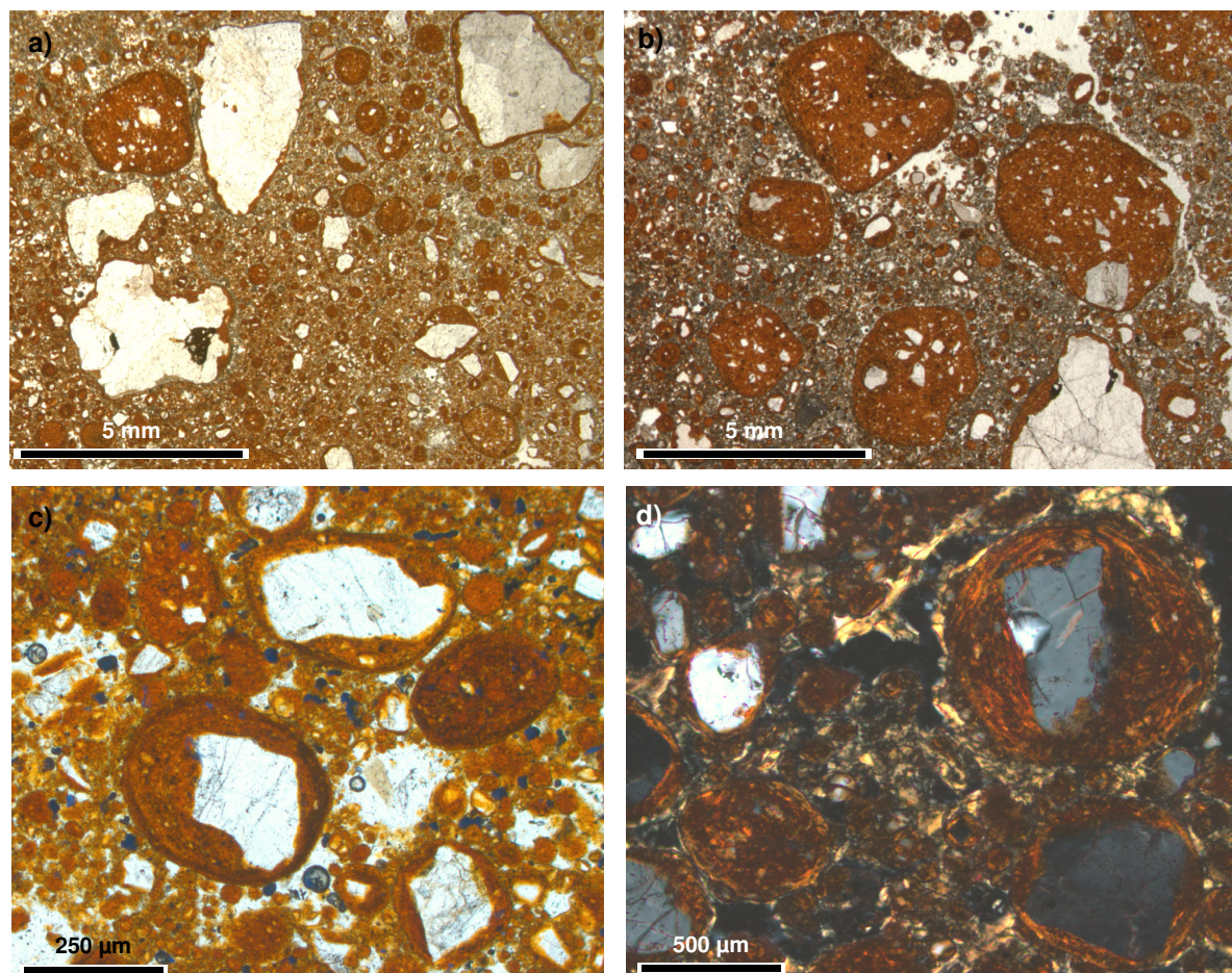
Figure 27 – Gravelles des grès rouges "sidérolithiques". a, b) Ces éléments ronds, relativement bien calibrés, de 100 à 500 \mu\text{m} de diamètre forment des assemblages granulaires, mêlés à des éléments plus grossiers comme des quartz et des nodules de grès à matrice argilo-ferrugineuse rouge (Naussac, 48) ; lumière polarisée. c) Le cœur des gravelles est soit formé d'un grain de quartz relativement gros, soit de matrice argilo-ferrugineuse. L'enveloppe des gravelles est d'épaisseur variable. Souvent elles possèdent un cortex plus ferrugineux (Naussac, 48) ; lumière polarisée. d) Les enveloppes de gravelles sont formées d'argiles orientées (Naussac, 48) ; lumière analysée.
