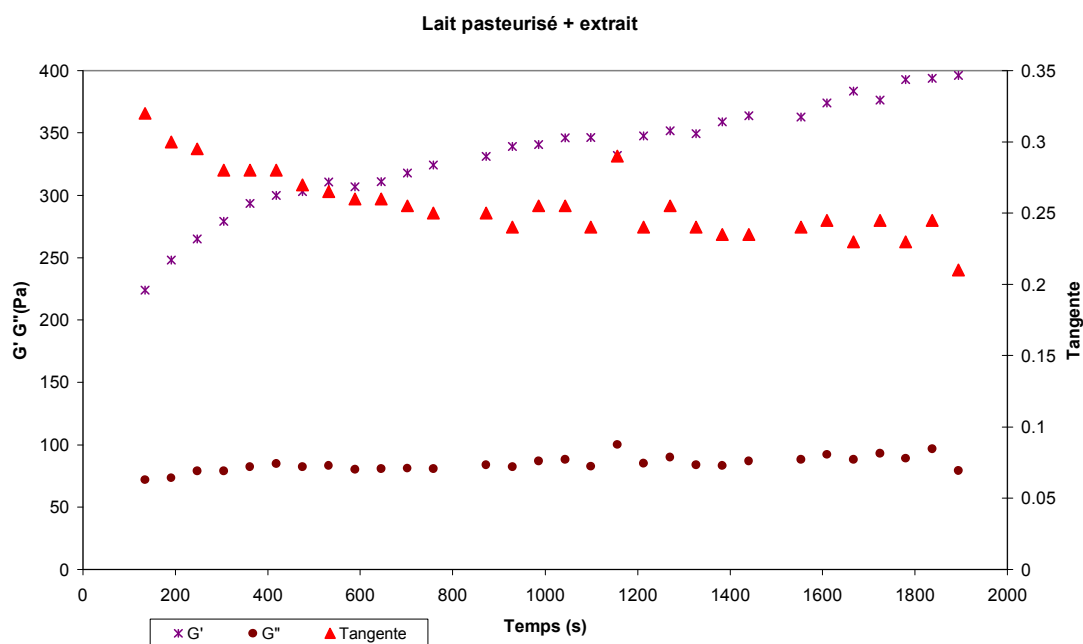
Figure 4.10 : Evolution du module conservatif G' , du module dissipatif G'' et du déphasage (tangente \delta ) au cours du temps lors de la coagulation du lait pasteurisé avec la présure.
