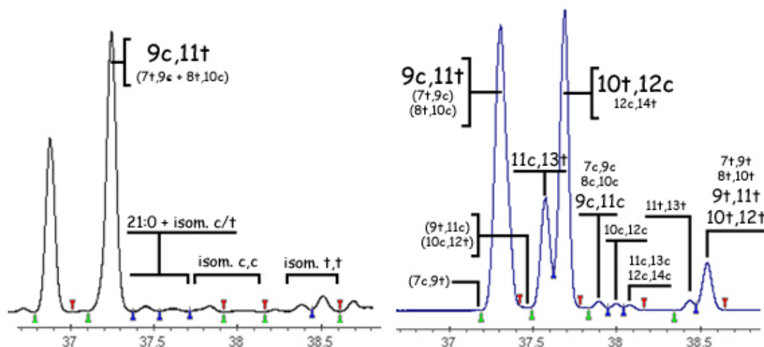
Figure 13 : Chromatogrammes partiels montrant la région d'éluion des isomères ALC d'un beurre (gauche) et d'un étalon commercial obtenu par synthèse chimique (droite) (cond. chromatogr. cf. § 3.2.1.5).
