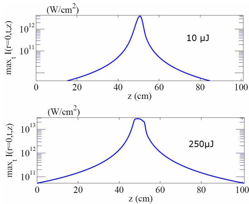
Figure 3.3. Profils d'intensité en fonction de la distance de propagation pour deux énergies différentes, 10 \mu J (en haut) et 250 \mu J (en bas).
