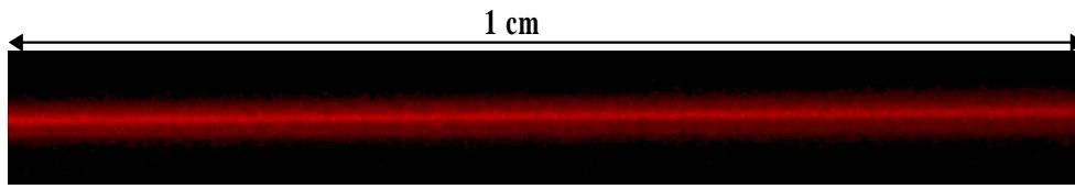
Figure 5.3. Image latérale de la trace de luminescence (sur 1 cm) laissée par un filament qui se propage dans le colorant non inversé. On peut observer un canal de lumière intense qui se propage entouré par son réservoir d'énergie. Energie initiale, 20 \mu J, diamètre du faisceau sur la lentille, 3.5 mm, focale de la lentille, 10 cm.
