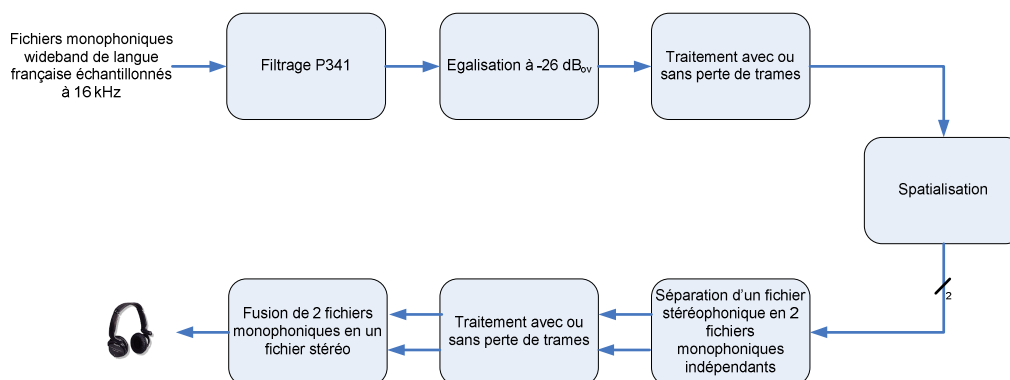
Figure 4.25 Traitement appliqué aux fichiers pour le test wideband pour la conférence centralisée
