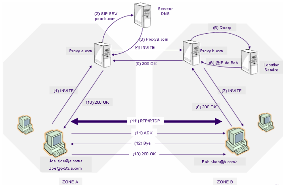
Figure 1.21 Exemple d'appel VoIP SIP
