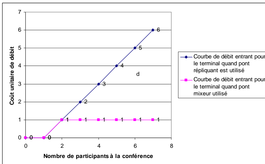
Figure 2.20 Comparaison en termes de bande passante entrante pour un terminal de chaque architecture
