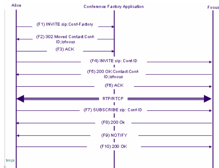
Figure 1.22 Création puis entrée en conférence
