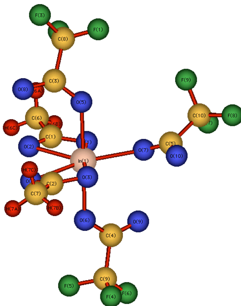
figure II-7 : représentation du complexe de l'indium dans le cristal \text{K}_2\text{InC}_{10}\text{O}_{10}\text{H}_6\text{F}_9 .
