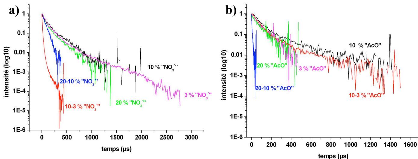
Figure IV-3 : déclins de luminescence du niveau ^4S_{3/2} pour les nanoparticules de CaF_2 synthétisées par la voie a) « nitrate » et b) « acétate ».
