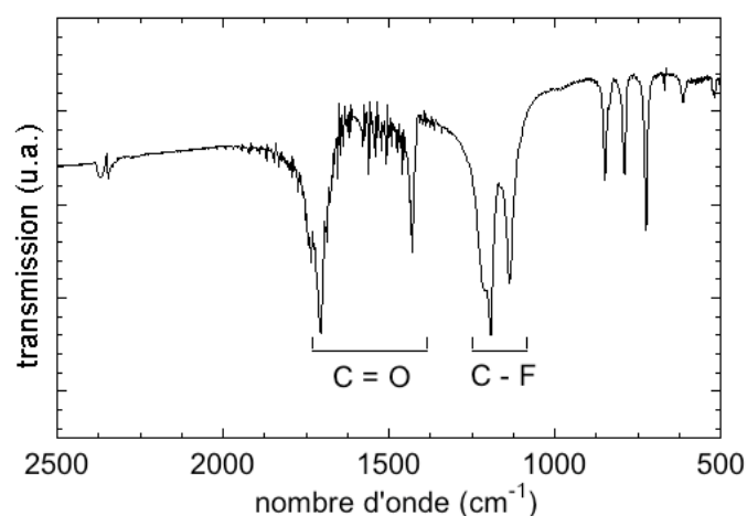
Figure II-10 : spectre FT-IR des cristaux broyés de \text{K}_3\text{InC}_{12}\text{O}_{12}\text{F}_{18} .
