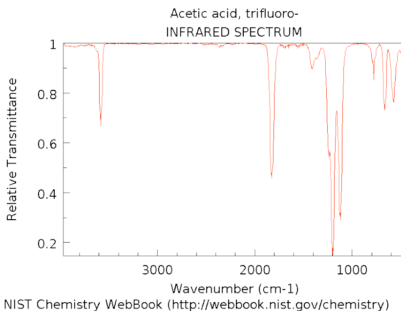
Figure II-11 : spectre FT-IR de la molécule d'acide trifluoroacétique obtenu en phase gazeuse.
