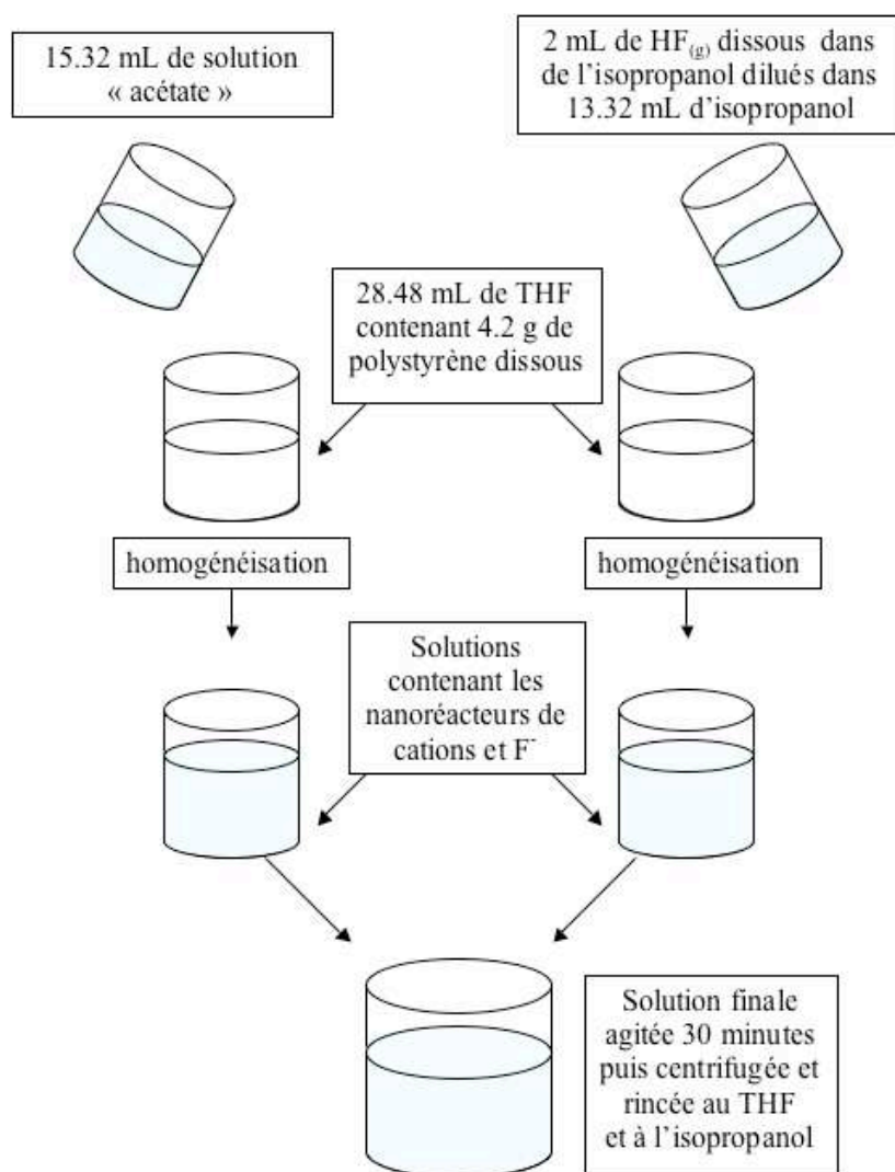
Figure III-9 : schéma de synthèse de nanoparticules de \text{CaF}_2 ou \text{PbF}_2 à partir de solutions « acétates » dans un système de nanoréacteurs non-aqueux pour un pourcentage volumique isopropanol / THF de 54 %.
