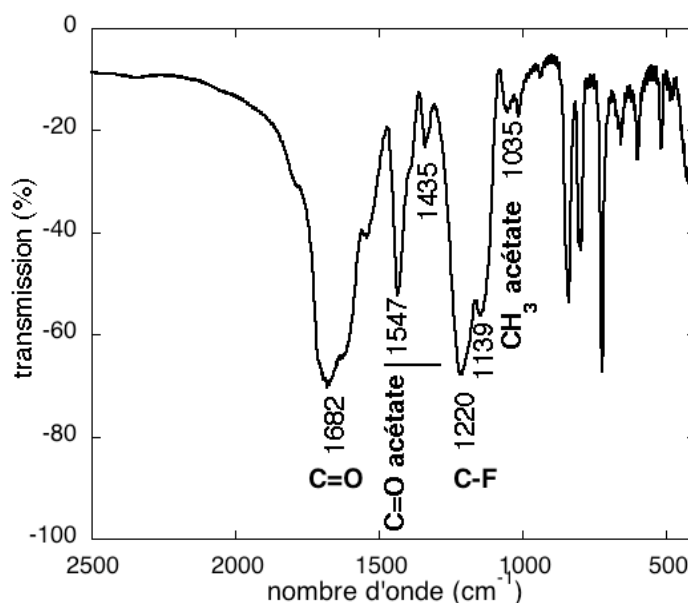
Figure II-12 : spectre FT-IR du précurseur de \text{PbF}_2 .
