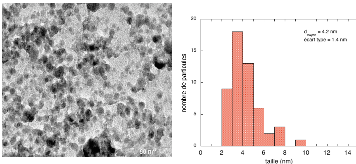
Figure III-27 : photographie MET des nanoparticules obtenues à température ambiante et leur histogramme de dispersion de taille à droite.
