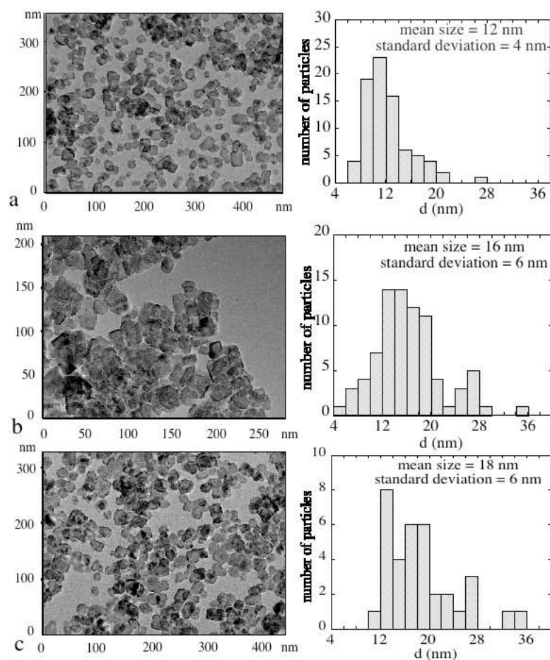
Figure III-13 : nanoparticules de \text{CaF}_2 obtenues à partir de précurseurs nitrates pour différents temps d'agitation, a) 10 minutes, b) 30 minutes et c) 120 minutes, pour un rapport isopropanol / THF = 54 %.
