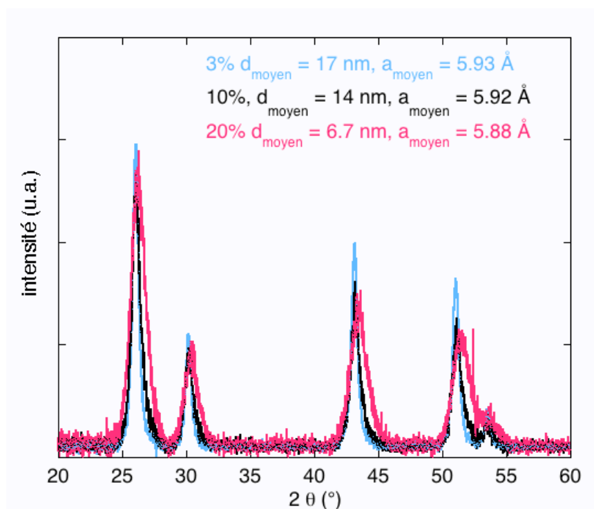
Figure III-23 : diffractogrammes X des nanoparticules de \text{PbF}_2 dopées ytterbium à différents pourcentages : 3, 10 et 20 % théoriques.
