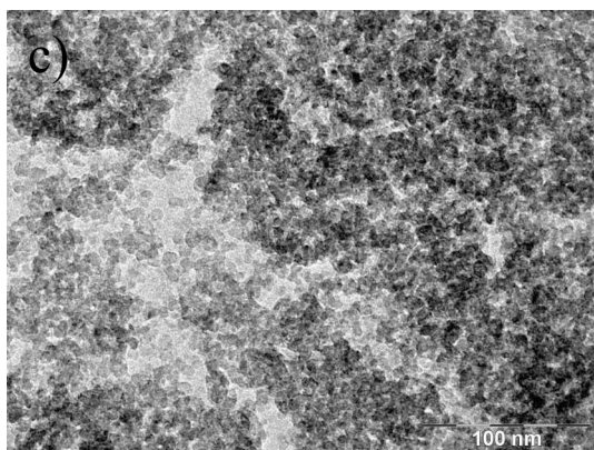
Figure III-15 : nanoparticules de \text{CaF}_2:\text{Er} dopées à a) 3 %, b) 10 % et c) 20 % obtenues à partir de précurseurs « acétates ».
