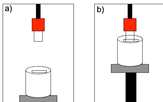
Figure II-15 : sch ma de dip-coating, a) avant et apr s que le film ait  t  d pos  ; b) pendant le d p t du film.
