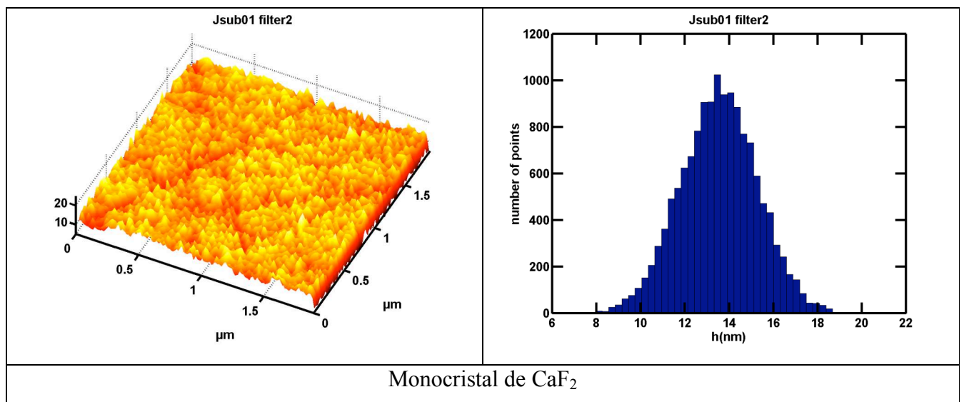
Figure II-23 : AFM d'un monocristal de \text{CaF}_2 utilisé comme substrat de couche mince
