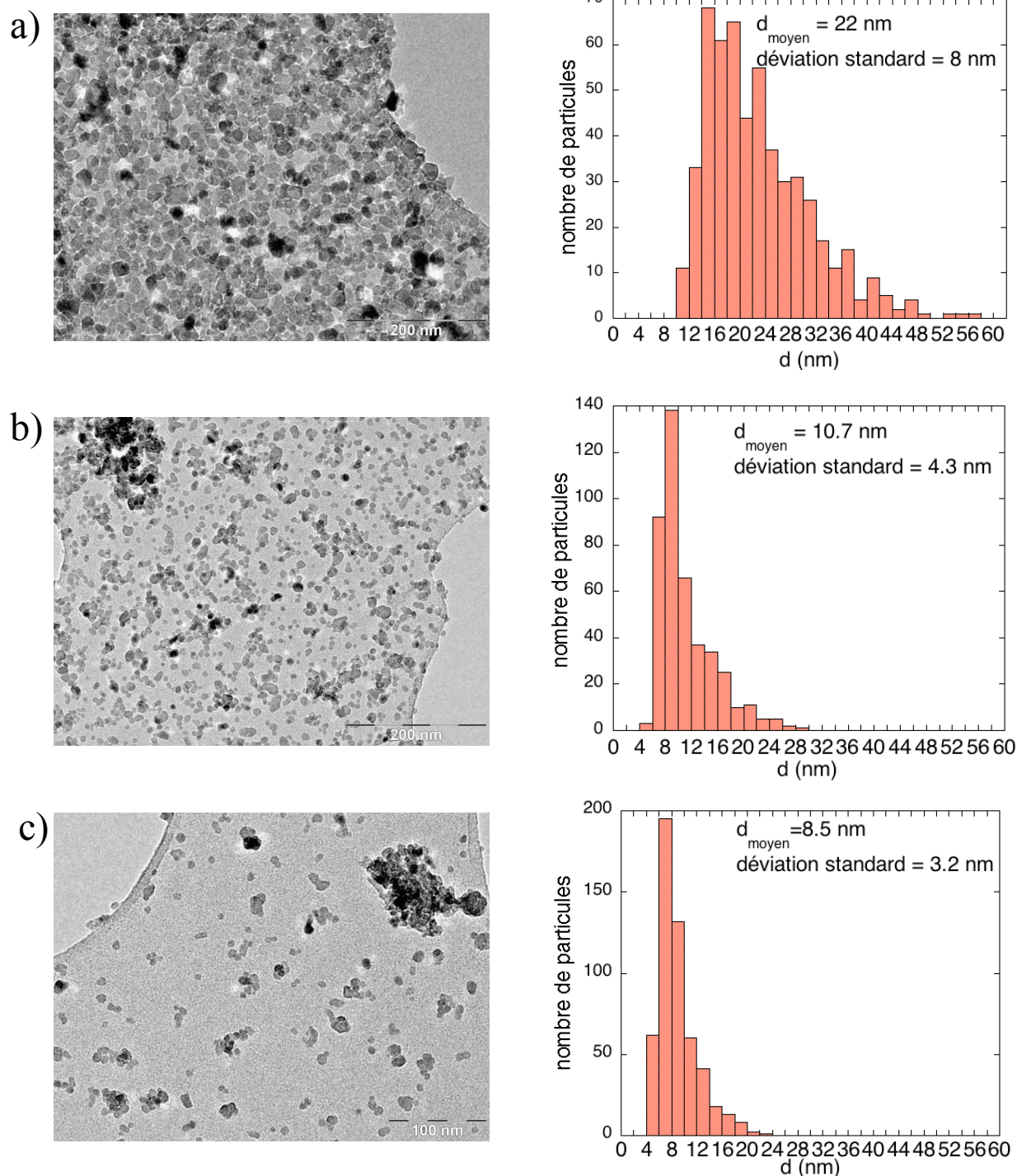
Figure III-16 : nanoparticules de \text{CaF}_2:\text{Er} dopées à a) 3 %, b) 10 % et c) 20 % obtenues à partir de précurseurs « nitrates ».
