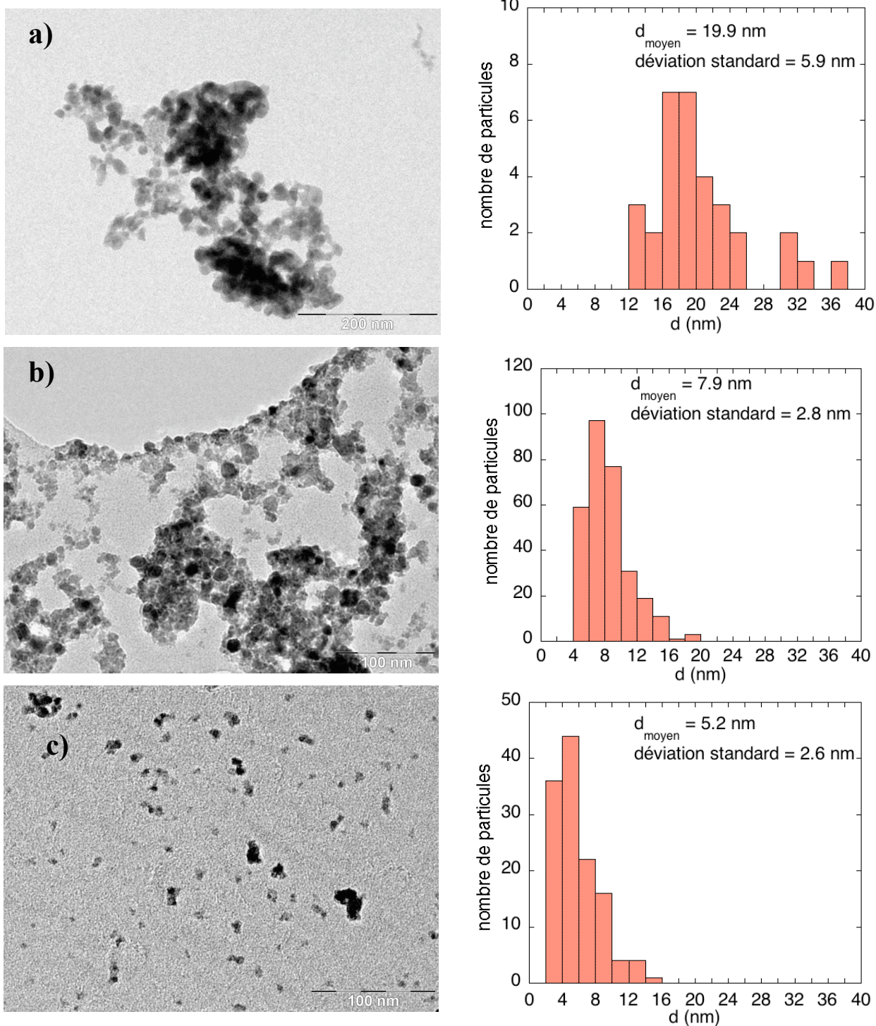
Figure III-24 : photographies MET des nanoparticules de \text{PbF}_2:\text{Yb} dopées à a) 3 %, b) 10 % et c) 20 % .
