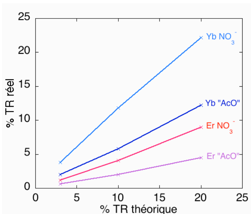
Figure III-14 : représentation des pourcentages réels de TR dans \text{CaF}_2 en fonction du pourcentage initialement prévu et des précurseurs cationiques (cf tableau III-10).
