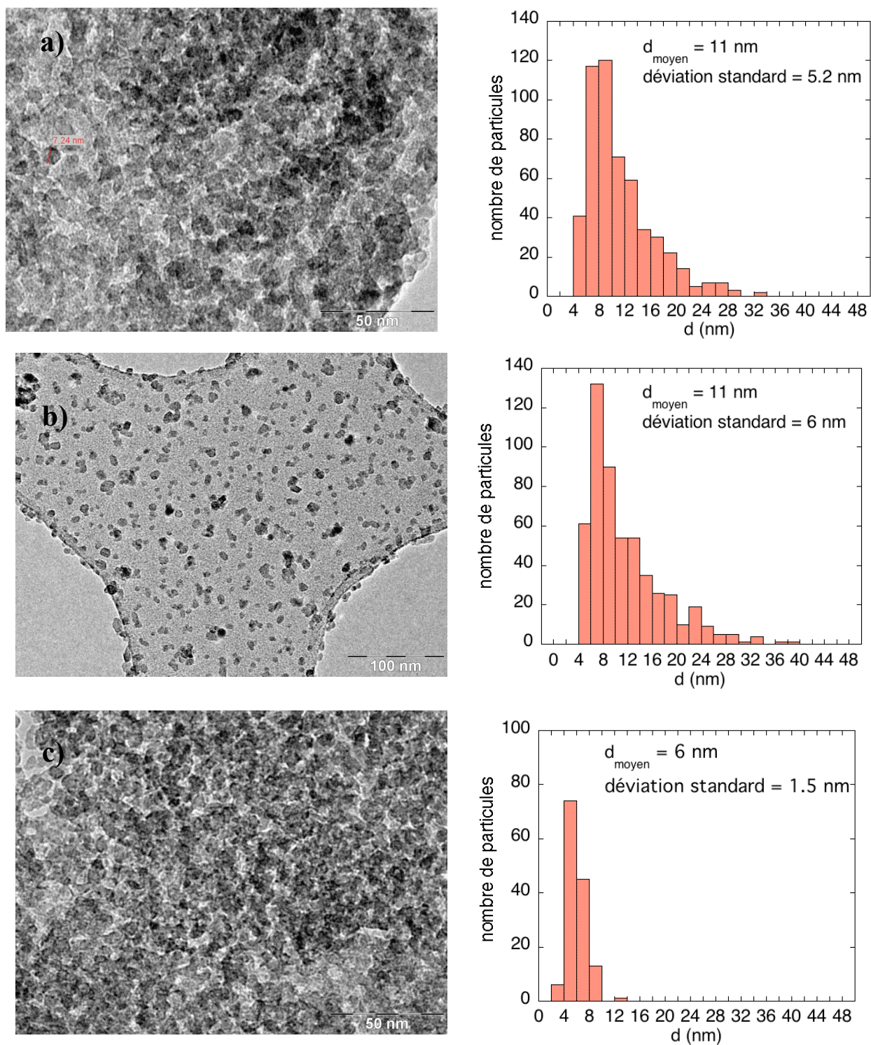
Figure III-17 : nanoparticules de \text{CaF}_2:\text{Yb} dopées à a) 3 %, b) 10 % et c) 20 % obtenues à partir de précurseurs « acétates ».
