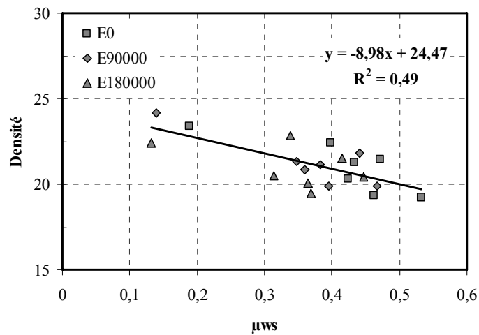
Figure V.38 : Évolution du paramètre Densité en fonction du frottement dans le cas de l'ensemble des enrobés (Profil seillé, Échelle de rugosité)
