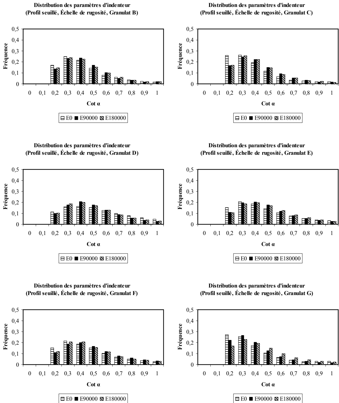
Figure VIII.29 : Distribution du paramètre « cot \alpha » (Profil seillé, Échelle de rugosité, Granulat B - G)
