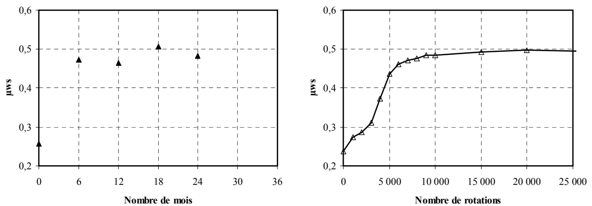
(c) Site de Coëx (BBTM 0/6)
