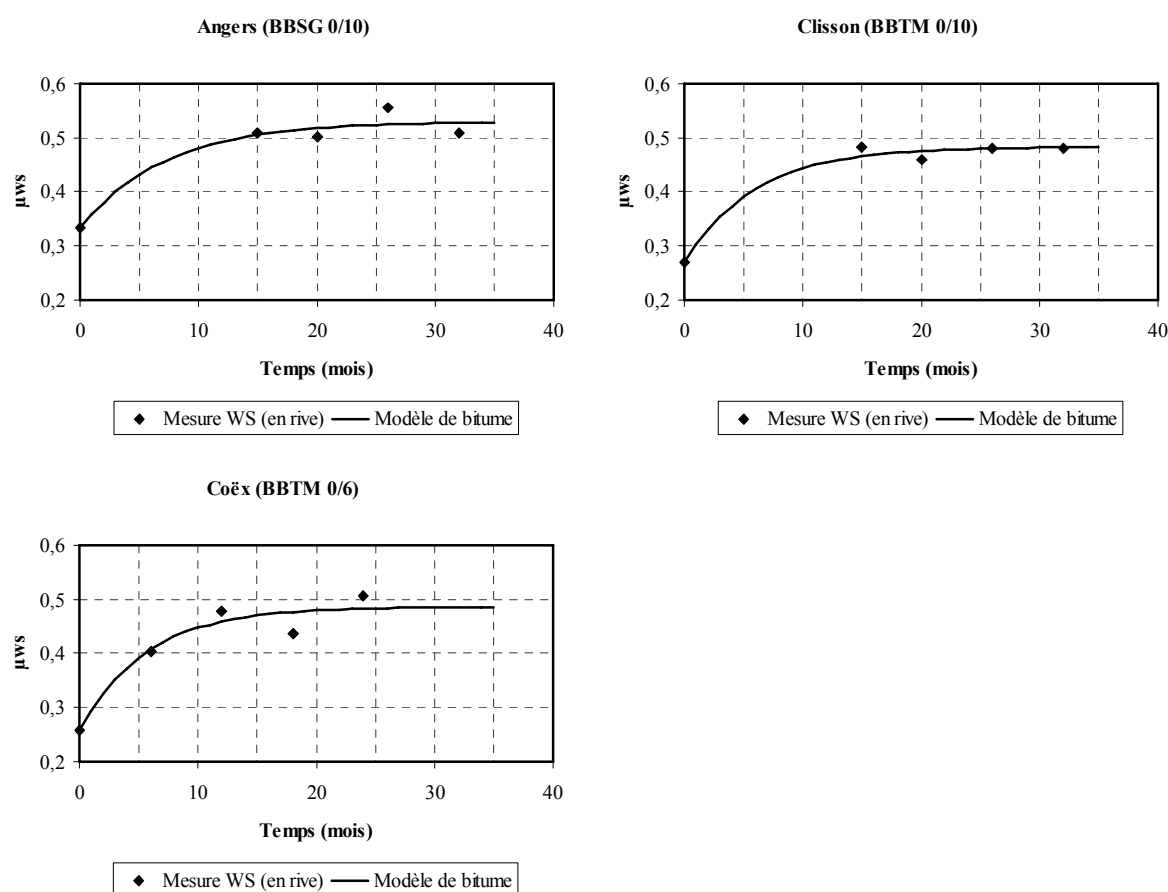
Figure VI.8 : Expression de la fonction du bitume \mu_B tenant compte du vieillissement
