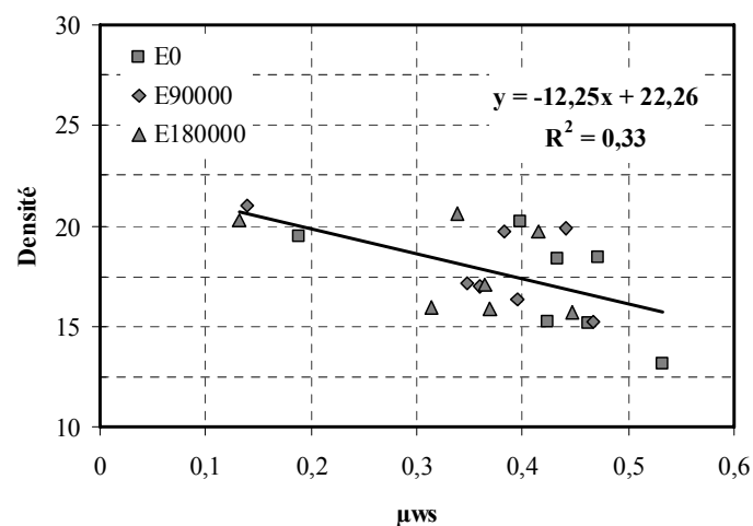
Figure V.30 : Évolution du paramètre \text{Densité} en fonction du frottement dans le cas de l'ensemble des enrobés (Profil entier, Échelle de rugosité)
