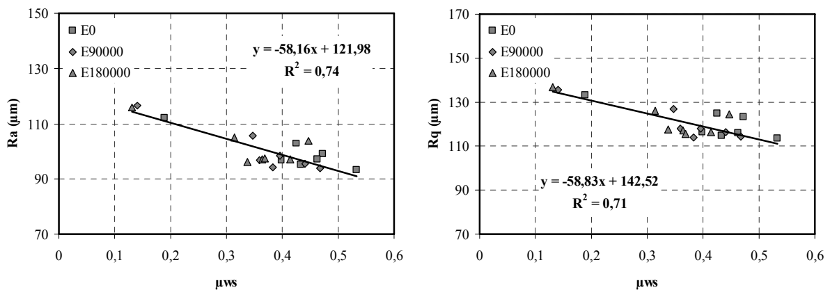
Figure V.39 : Évolutions des paramètres R_a et R_q en fonction du frottement dans le cas de l'ensemble des enrobés (Profil seillé, Échelle de rugosité)
