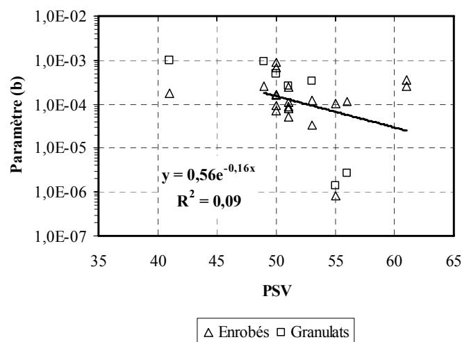
Figure VIII.83 : Relation entre le paramètre (b) et PSV
