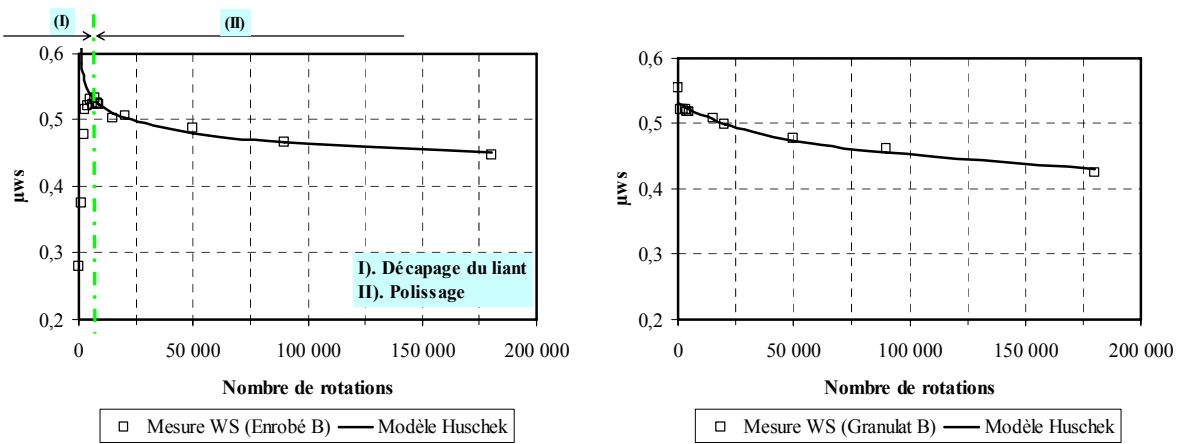
(a) Cas d'un BBTM 0/6, fabrication en laboratoire
