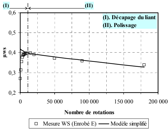
(a) Cas d'un BBTM 0/10, fabrication en laboratoire
