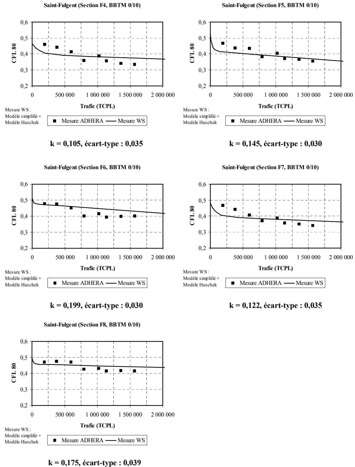
Figure VI.14 : Comparaisons entre les évolutions réelles et simulées du site de Saint-Fulgent avec les paramètres « k » variables
