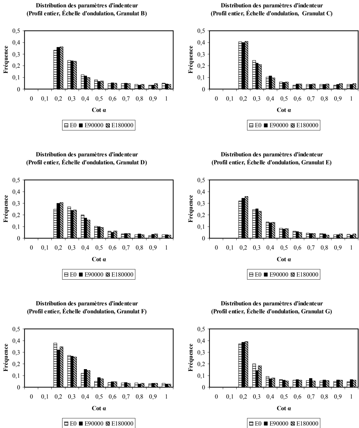
Figure VIII.26 : Distribution du paramètre « cot \alpha » (Profil entier, Échelle d'ondulation, Granulat B - G)
