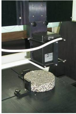
(a) Système de mesure LCPC en laboratoire (b) Principe du capteur (émission et diffusion) [145]
