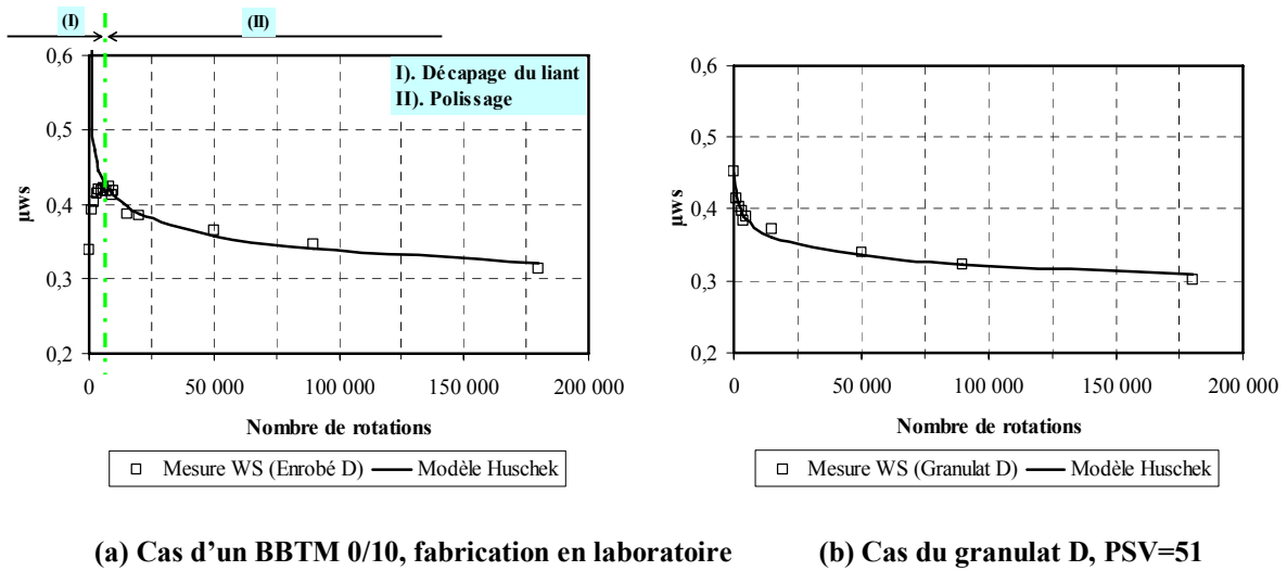
Figure VIII.51 : Courbes d'évolution comparées : mesures et modèle Huschek
