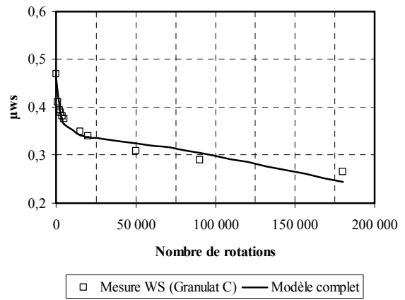
(b) Cas du granulat C, PSV=53
