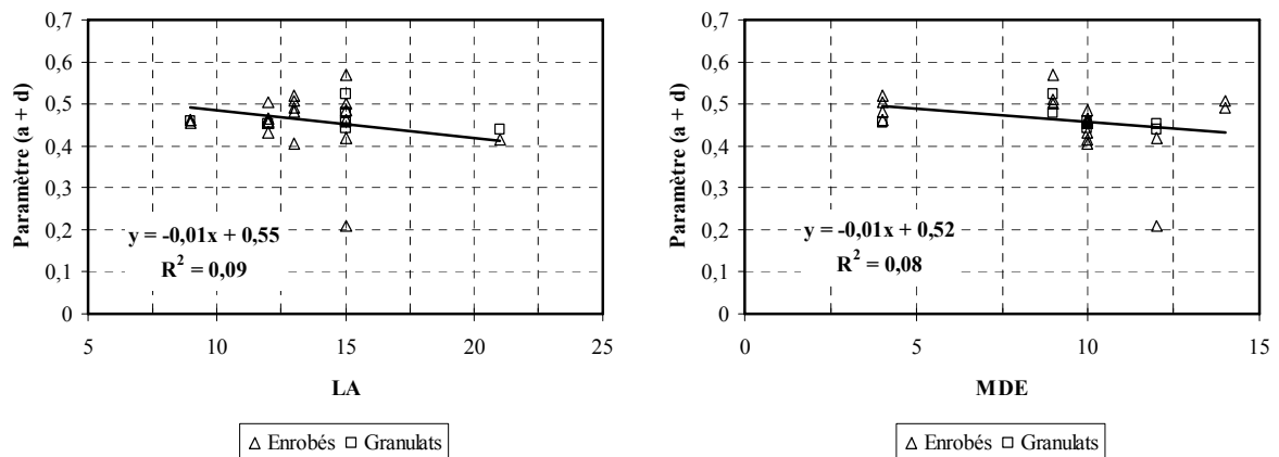
Figure VIII.76 : Relations entre le coefficient de frottement maximal et les valeurs LA et MDE
