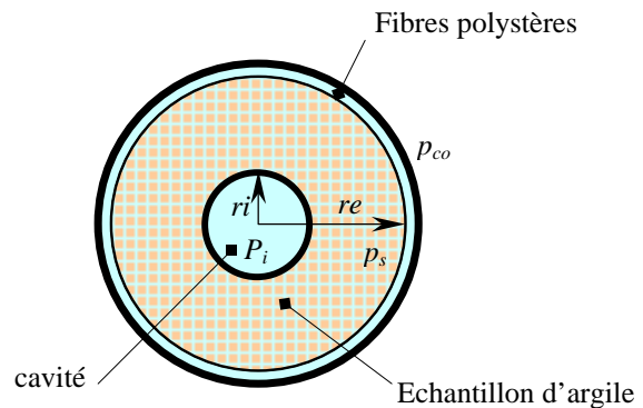
Figure III.41- Coupe transversale de l'échantillon d'argile.
