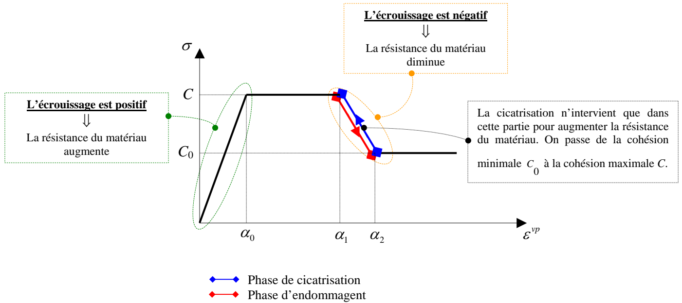
Figure IV.10 - Représentation de la phase d'endommagement et de cicatrisation dans la courbe de variation de la cohésion en fonction du paramètre d'écrouissage.
