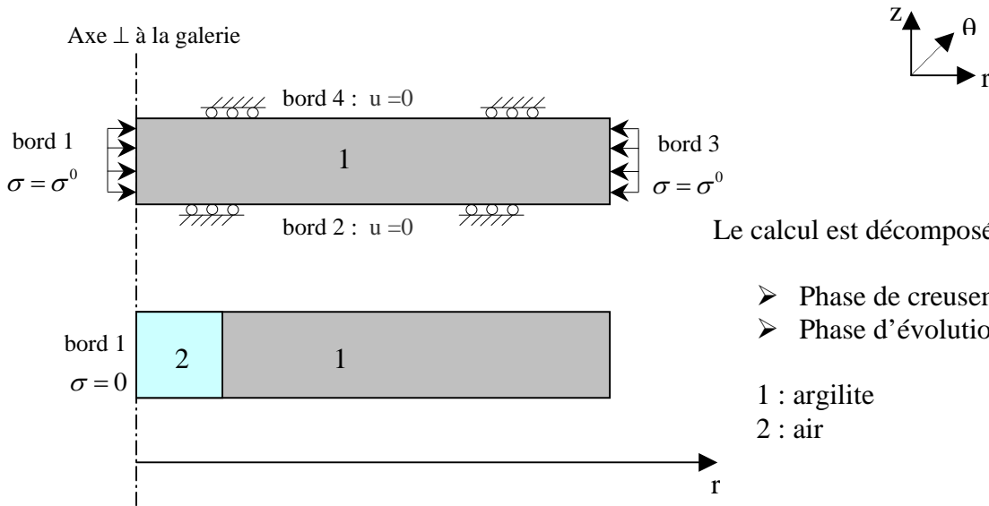
Figure V.18 - Modèle 2D axisymétrique pour un tunnel sans soutènement Pour le cas d'un tunnel avec soutènement :
