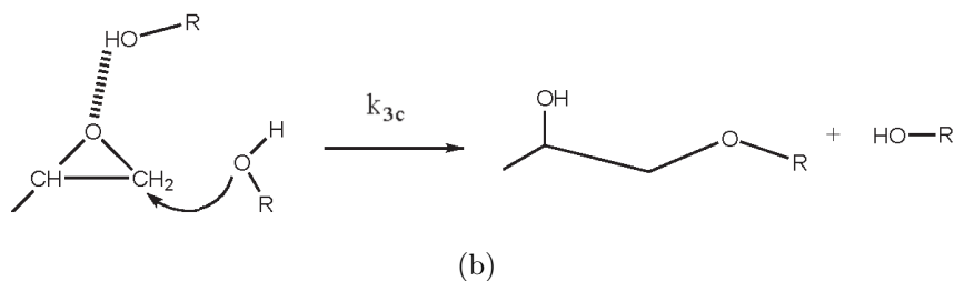
FIG. 2.11 – Étapes mettant en jeu la réaction des groupes hydroxyles par un mécanisme non catalytique (a) et auto-catalytique (b)
