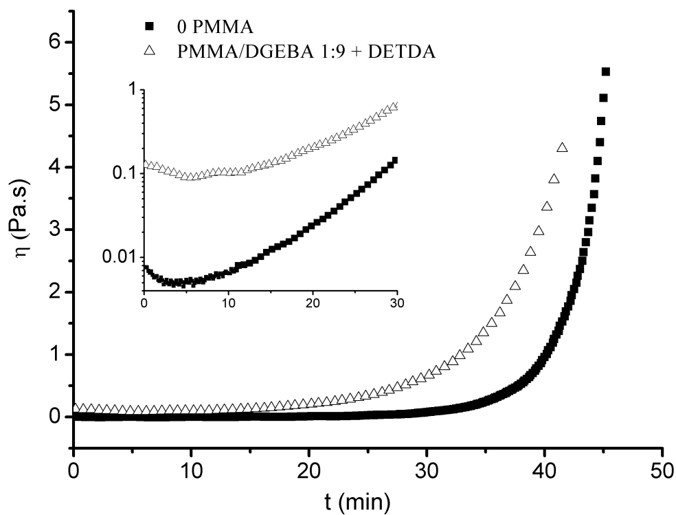
FIG. 4.27 – Variation de la viscosité à cisaillement nul pour le système DGEBA/DETDA modifié par 10% en PMMA ( en masse par rapport à DGEBA) comparé à celle du système non modifié à 140°C
