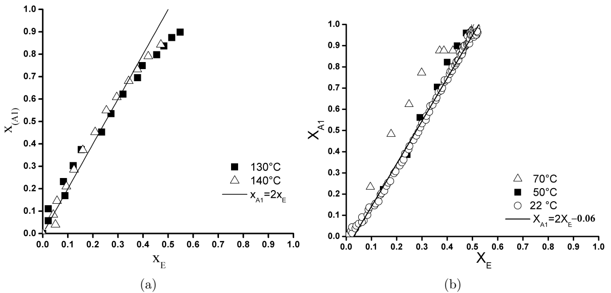
FIG. 4.7 – Taux de conversion des groupes amine primaire en fonction de celui des groupes époxy dans le cas des systèmes DGEBA/DETDA (a) DGEBA/IPD (b)
