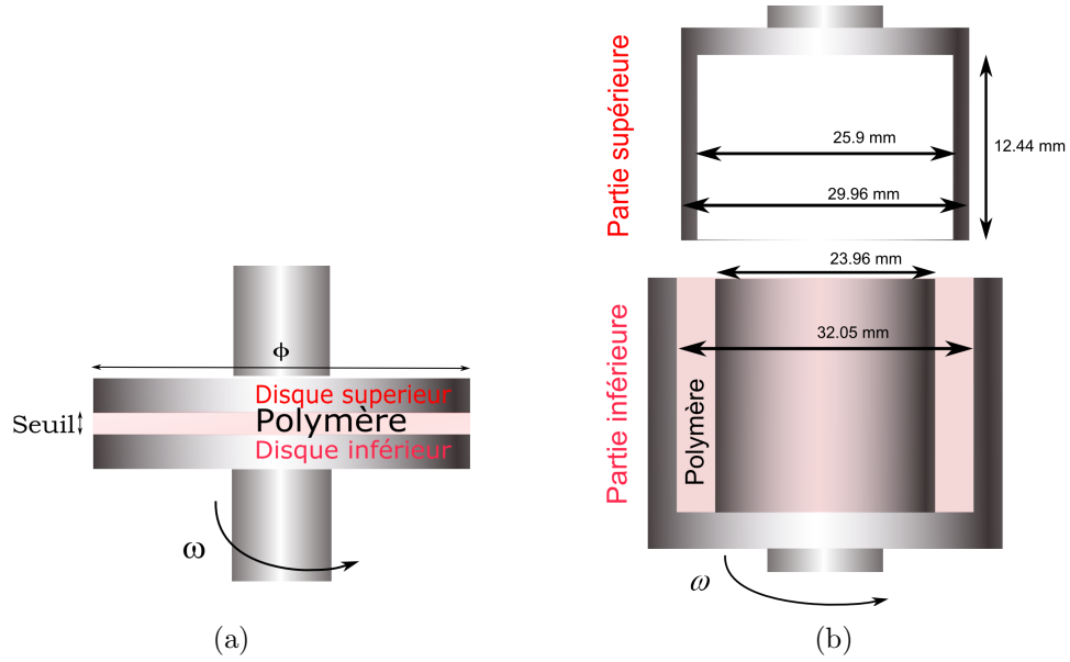
FIG. 3.8 – Mesure de la viscosité : Géométrie plan-plan (a), Géométrie double couette (b)
