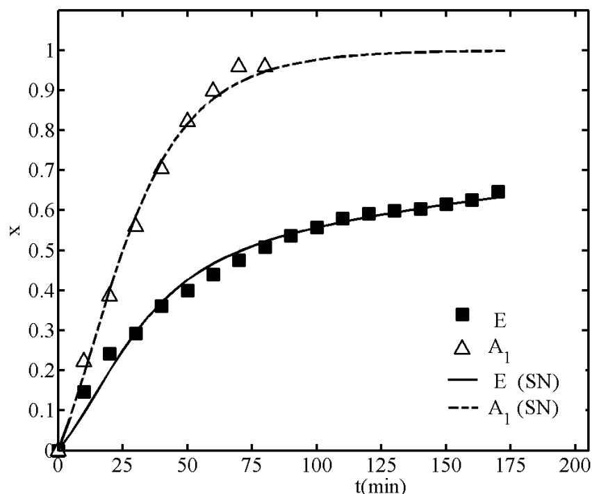
FIG. 4.14 – Taux de conversion (DGEBA/IPD) T_c = 50^\circ\text{C}
