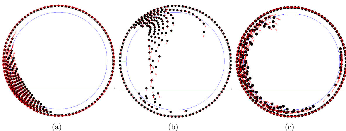
FIG. 5.15 – Évolution de l'écoulement pour une viscosité de 1 Pa.s après 1 (a), 3 (b), et 5 (c) secondes.
