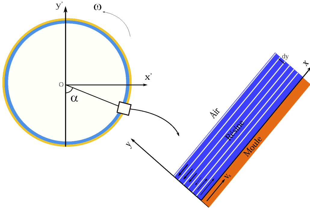
FIG. 2 – Couches d'écoulement
