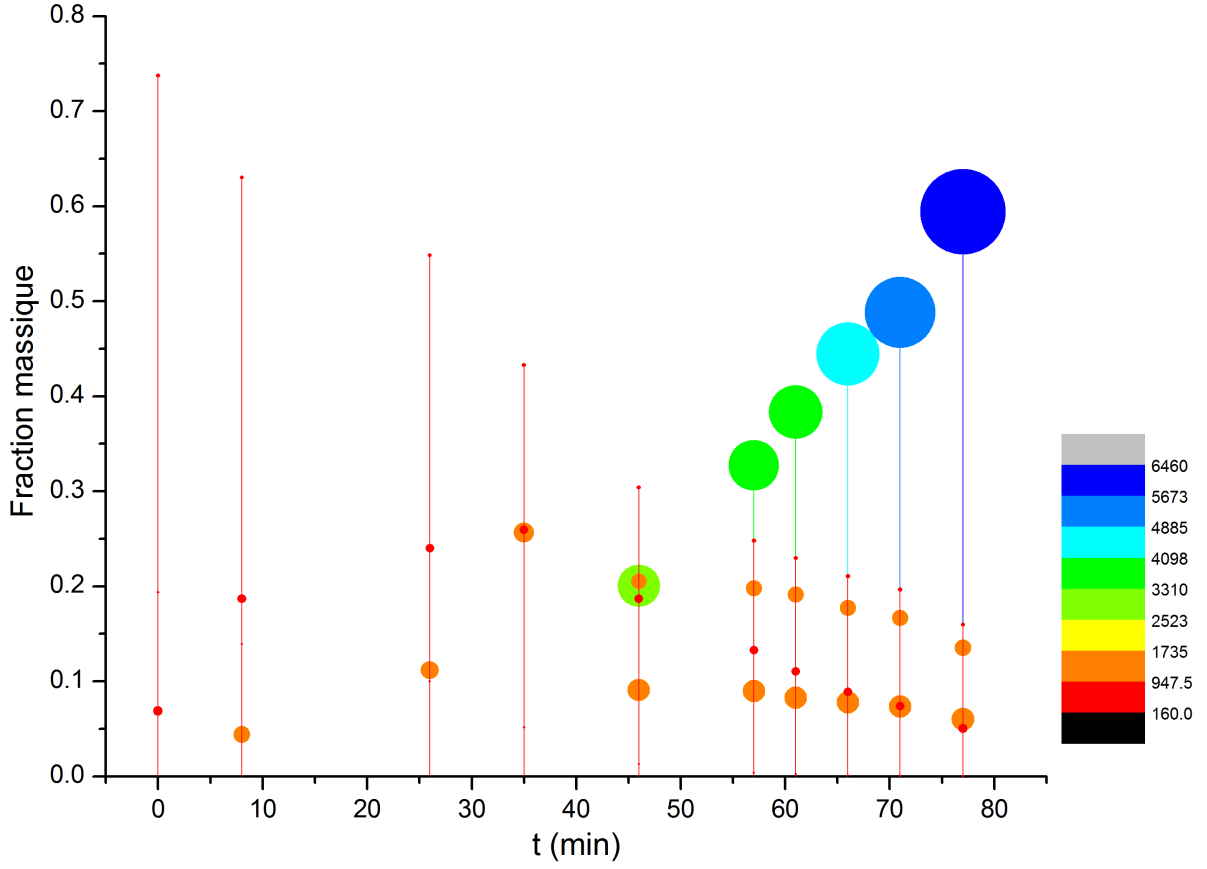
FIG. 4.16 – Dispersion des masses molaires au cours de la réticulation du système DGEBA/DETDA en bain d'huile thermostaté à 130°C.
