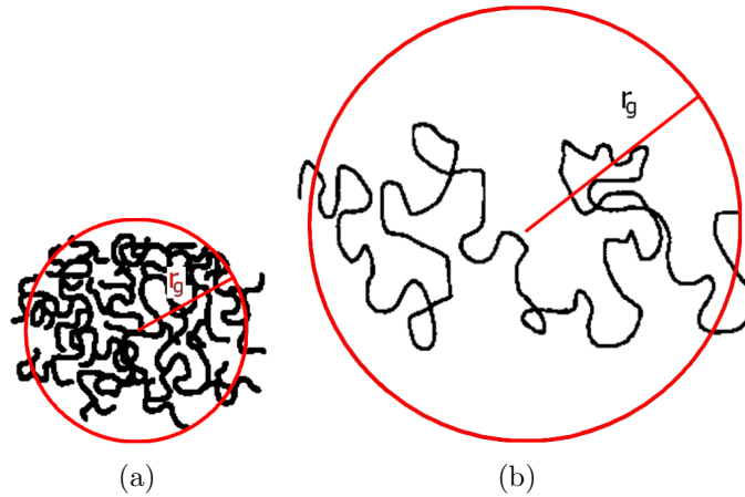
FIG. 2.18 – Rayons de gyration r_g des polymères ramifiés et linéaires de même degré de polymérisation N : (a) r_g \propto N^{\frac{1}{4}} , (b) r_g \propto N^{\frac{1}{2}}
