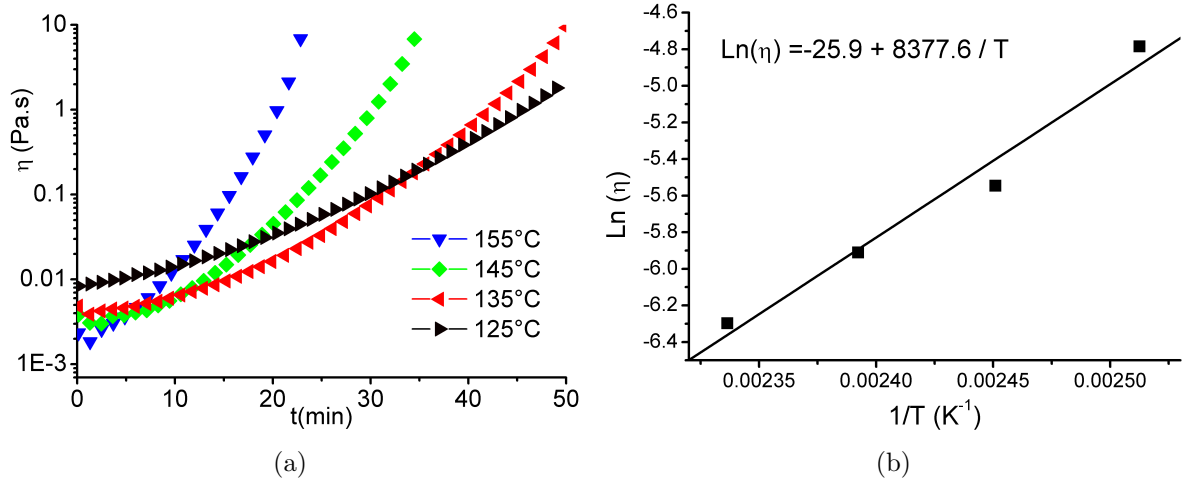
FIG. 4.21 – Variation de la viscosité dynamique mesurée à 1Hz en fonction du temps pour différentes températures de réticulation (a) ; Graphe d'Arrhenius pour la viscosité initiale ( \eta' ) dans le cas du système DGEBA/DETDA (b).
