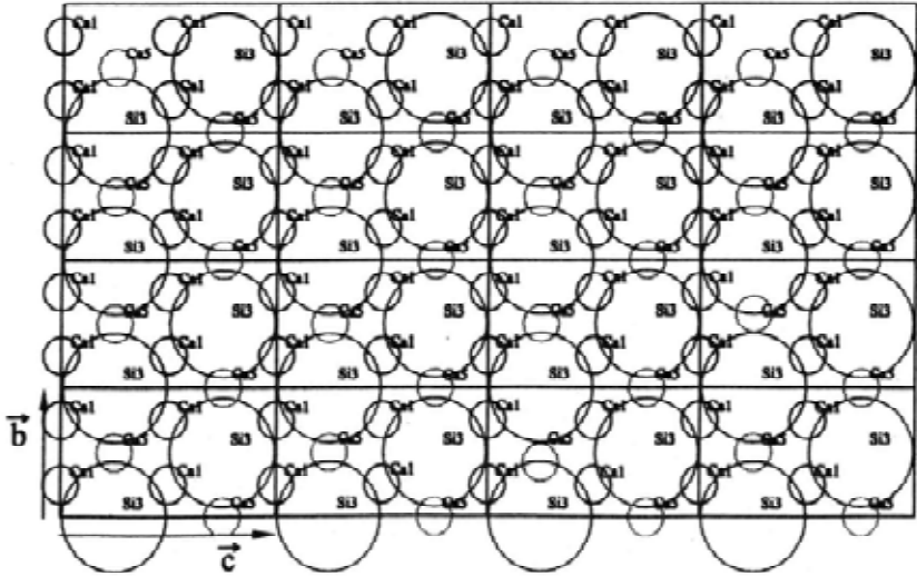
Figure III-14 : Plans hexagonaux dans la structure de Mumme x = 1/3 (bas), x = 0 (centre), x = 2/3 (haut)
