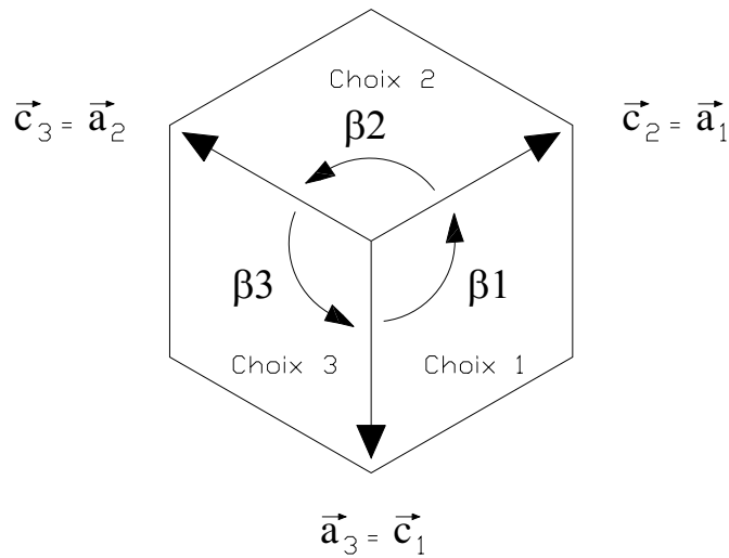
Figure A1-6 : Les trois choix (\vec{a}_1, \vec{c}_1) , (\vec{a}_2, \vec{c}_2) , (\vec{a}_3, \vec{c}_3) associés à un axe unique \vec{b}
