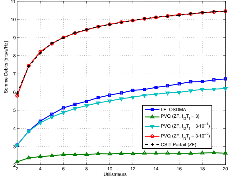
Figure 7: Somme des débits en fonction du nombre d'utilisateurs avec un canal corrélé temporellement, M = 2 antennes et \text{SNR} = 10 dB.
