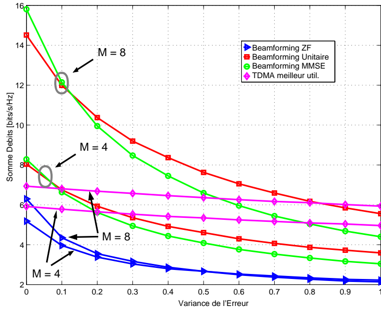
Figure 10: Somme des débits en fonction de la variance de l'erreur d'estimation du canal pour M = 4, 8 antennes, K = M utilisateurs et \text{SNR} = 10 dB.
