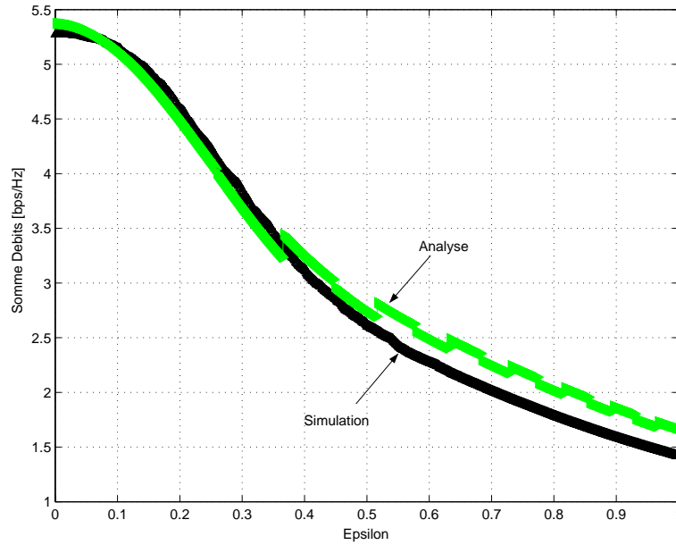
Figure 2: Comparaison des résultats analyse-simulation de la borne inférieure sur la somme des débits en utilisant la métrique III, pour M = 2 antennes, K = 15 utilisateurs, \text{SNR} = 10 dB et B = 1 bit.
