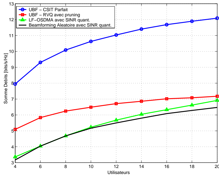
Figure 11: Somme des débits en fonction du nombre d'utilisateurs dans un système avec beamforming linéaire et sélection d'utilisateurs, M = 4 antennes, \text{SNR} = 10 dB, et B = 10 bits sur la voie de retour.
