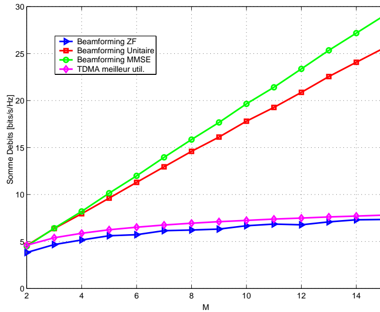
Figure 9: Somme des débits en fonction du nombre d'antennes M pour K = M utilisateurs et SNR = 10 dB.
