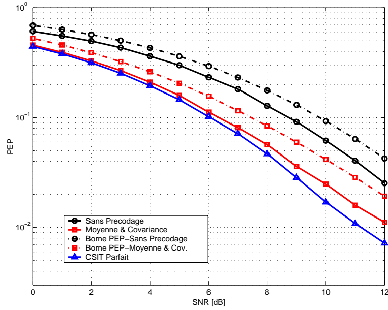
Figure 1: PEP en fonction du SNR pour différents niveaux de CSIT, \rho = 0.9 and \gamma = 40\%
