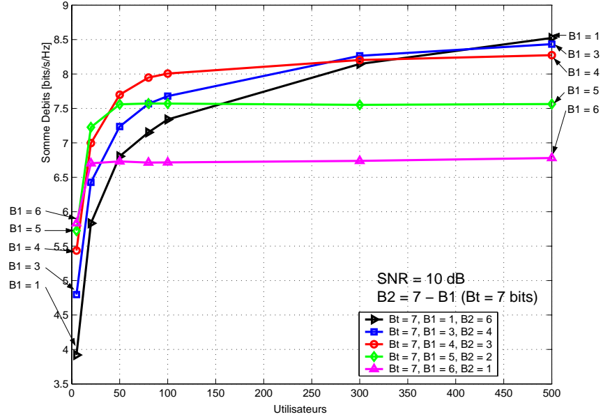
Figure 5: Somme des débits en fonction du nombre d'utilisateurs pour M = 2 et \text{SNR} = 10 dB.
