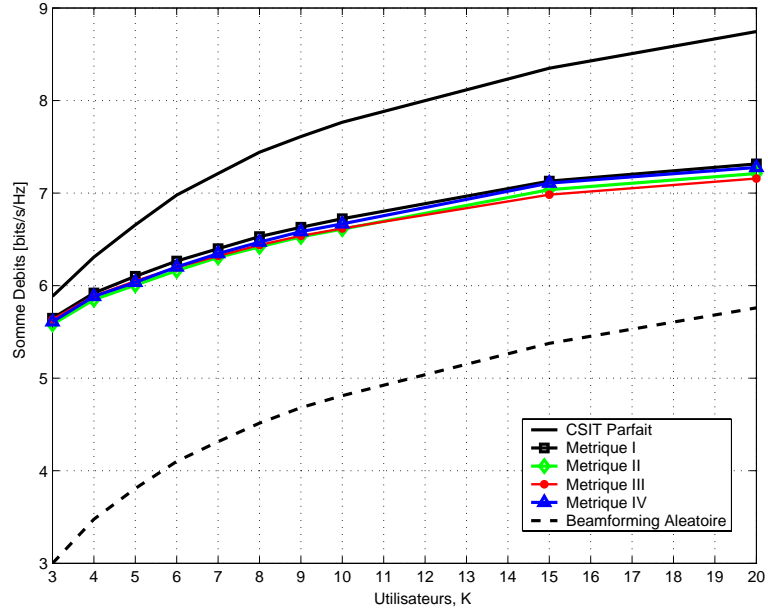
Figure 3: Somme des débits obtenue par différentes approches de feedback en fonction du nombre d'utilisateurs, pour B = 9 bits, M = 3 antennes au transmetteur et \text{SNR} = 10 dB.
