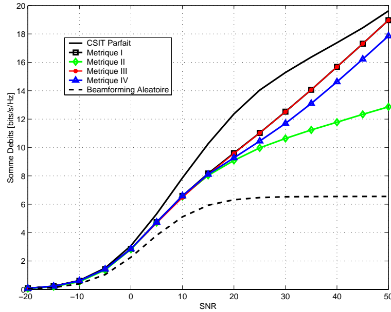
Figure 4: Somme des débits obtenue par différentes approches de feedback en fonction de SNR moyen, pour B = 9 bits, M = 3 antennes et K = 10 utilisateurs.
