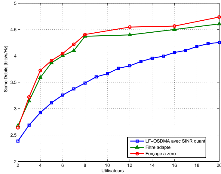
Figure 6: Somme des débits en fonction du nombre d'utilisateurs dans un canal corrélé spatialement, M = 2 antennes et \text{SNR} = 10 dB.
