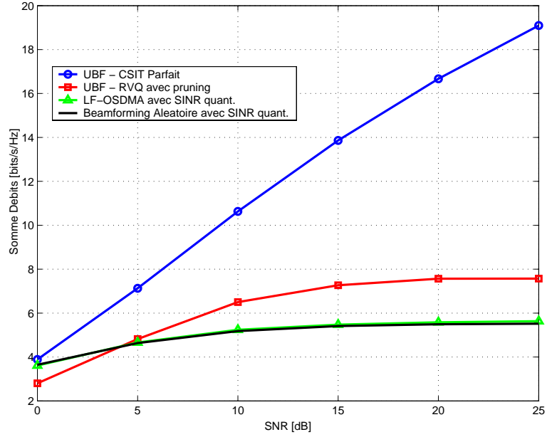
Figure 12: Somme des débits en fonction de SNR moyen dans un système avec beamforming linéaire et sélection d'utilisateurs, M = 4 antennes, K = 10 utilisateurs, et B = 10 bits sur la voie de retour.
