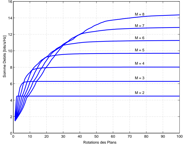
Figure 8: Somme des débits en fonction du nombre de rotations de plans (itérations de l'algorithme) pour différents nombres d'antennes au transmetteur, K = M utilisateurs et \text{SNR} = 10 dB.
