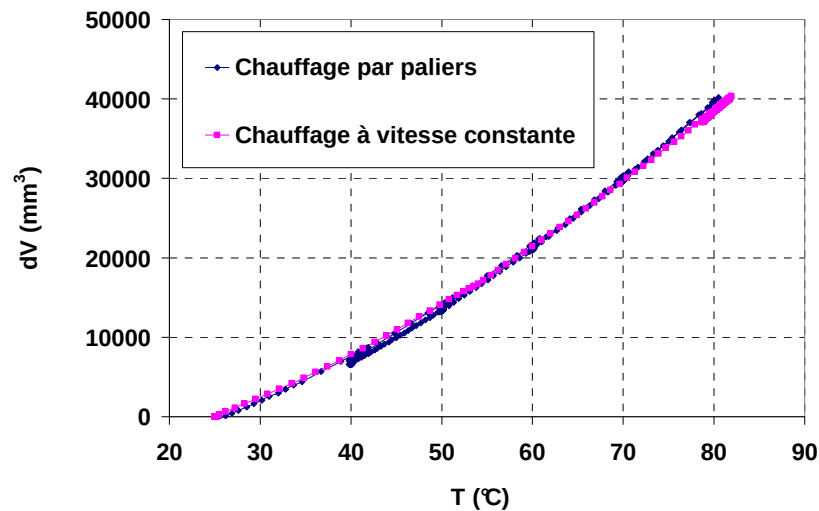
Figure 2- 36. Comparaison entre les résultats d'étalonnage du chauffage par palier et par rampe de 25 à 80 ^{\circ}\text{C} (pression de confinement = 3,5 MPa, contre pression = 1 MPa)
