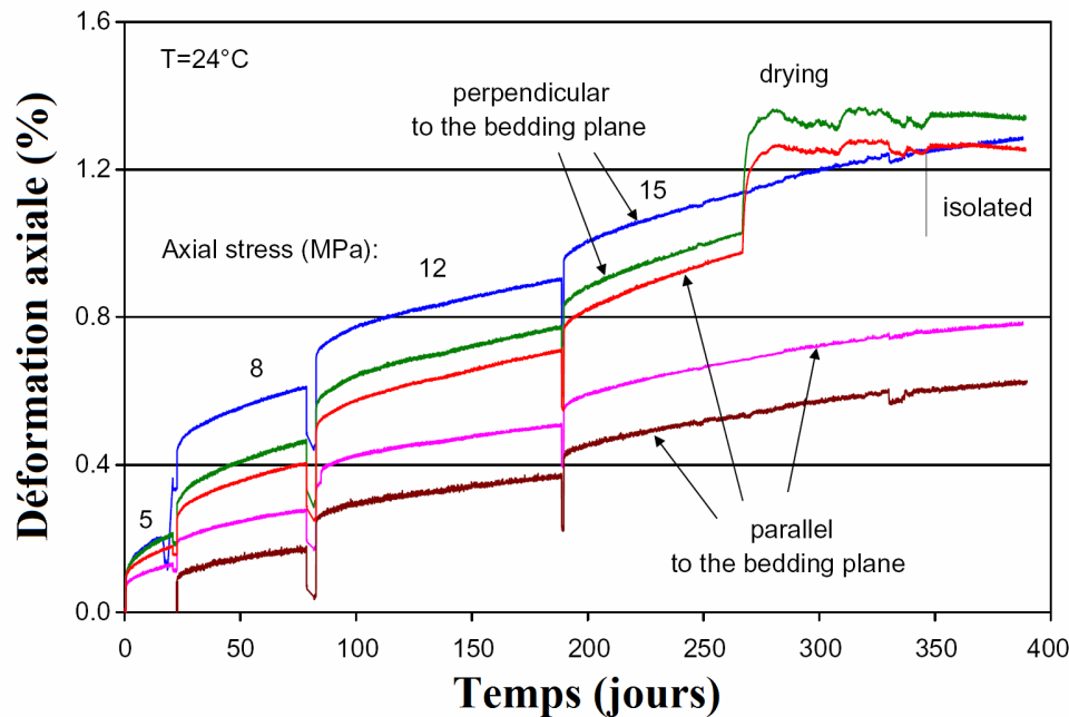
Figure 1- 15. Comportement différé de l'argile du Callovo-Oxfordien (Zhang et Rothfuchs, 2004)
