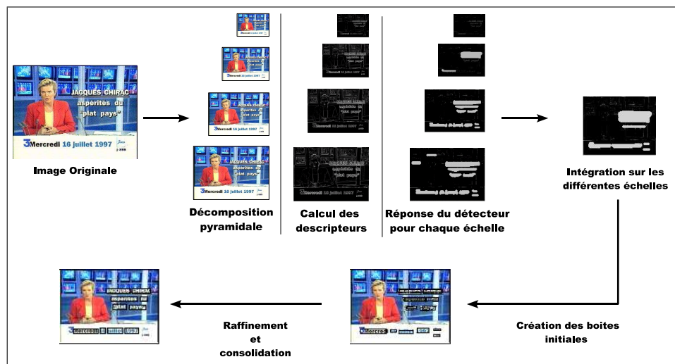
FIG. 4.1: Exemple didactique. Schéma algorithmique type d'un système de localisation de texte utilisant l'apprentissage
