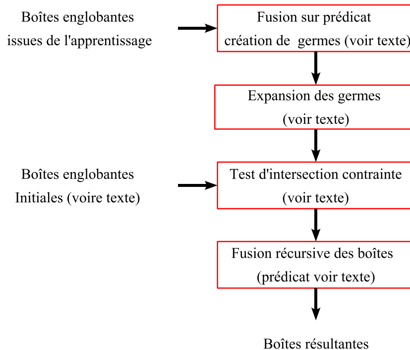
FIG. 9.28: Schéma récapitulatif du module itératif de regroupement des composantes connexes.
