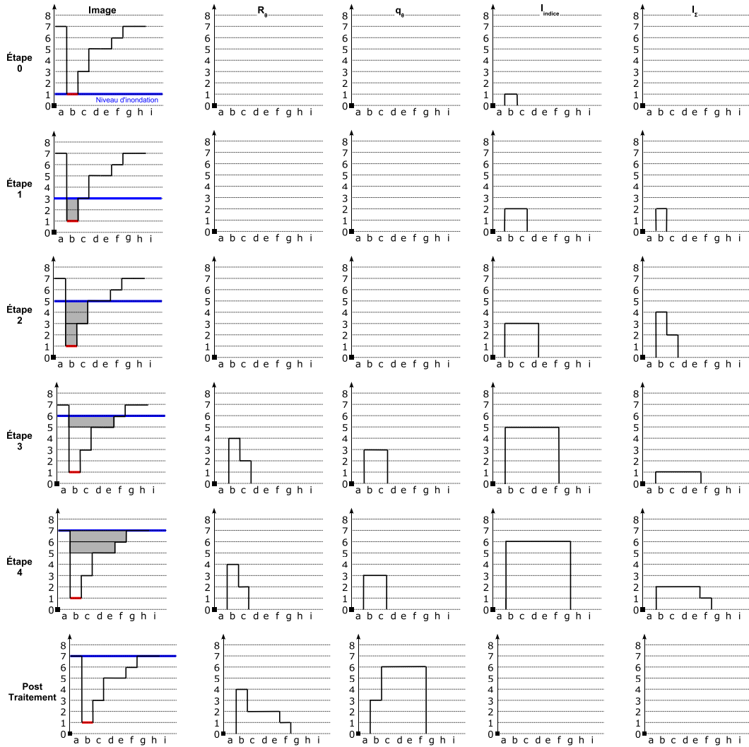
FIG. 8.10: Fermeture ultime surfacique (avec un pas d'ouverture unitaire) par inondation prenant en compte l'accumulation. De gauche à droite l'image inondée, R_\theta , q_\theta et les deux images auxiliaires permettant la prise en compte de l'accumulation I_\Sigma , I_{indice} . De haut en bas les différentes étapes de l'inondation (avec sur la première colonne : en trait gras le niveau d'inondation, et en grisé les structures de l'image pouvant participer à l'accumulation).
