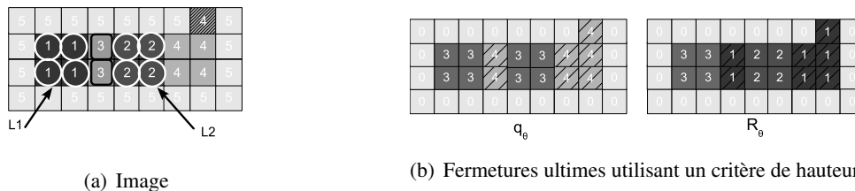
FIG. 8.8: Exemple de problèmes lors de la fusion de lacs pour le critère de hauteur
