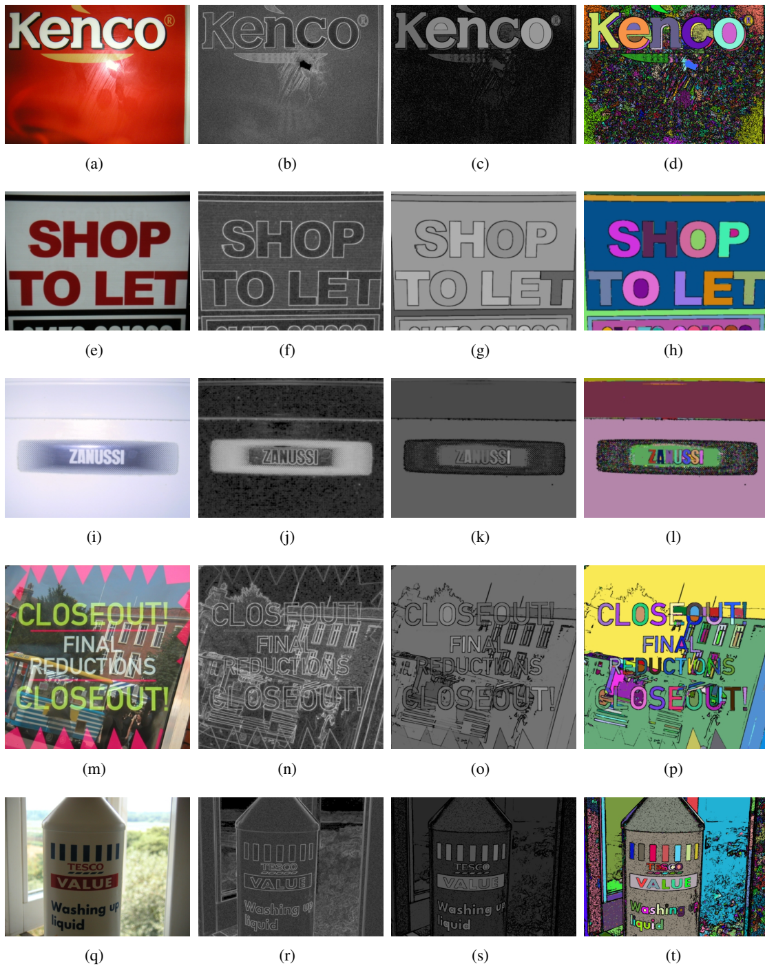
FIG. 7.20: Approche Gradient :utilisation de l'opérateur de fermeture ultime par hauteur. Présentation de segmentation satisfaisante en l'absence de tout autre traitement . De gauche à droite : image originale, gradient morphologique sur le canal luminance (Correction \gamma = 3 ), R_\theta (Correction \gamma = 3 ), q_\theta labellisée .Base ICDAR [53]
