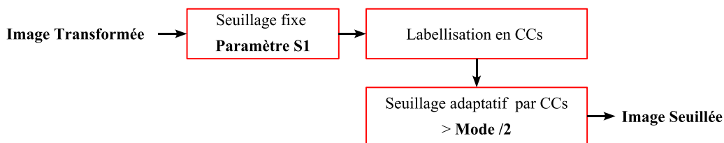
FIG. 9.3: Module de seuillage de l'image transformée R_\theta
