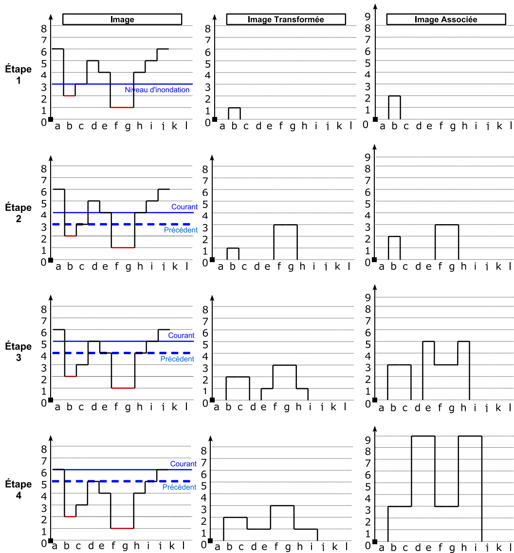
FIG. 8.2: Étapes de l'implémentation par inondation de la fermeture ultime par critère surfacique
