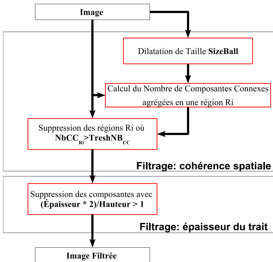
FIG. 9.6: Architecture du module de filtrage grossier.
