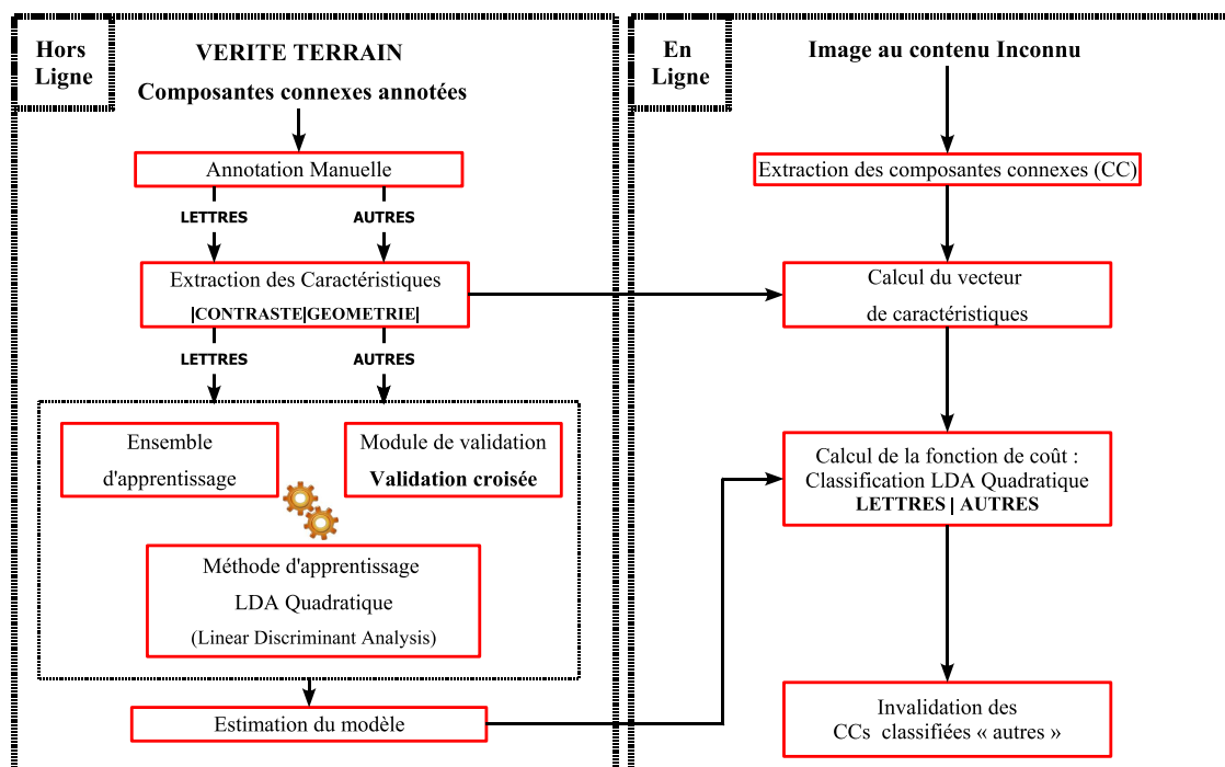
FIG. 9.12: Architecture du module de sélection des composantes par apprentissage.
