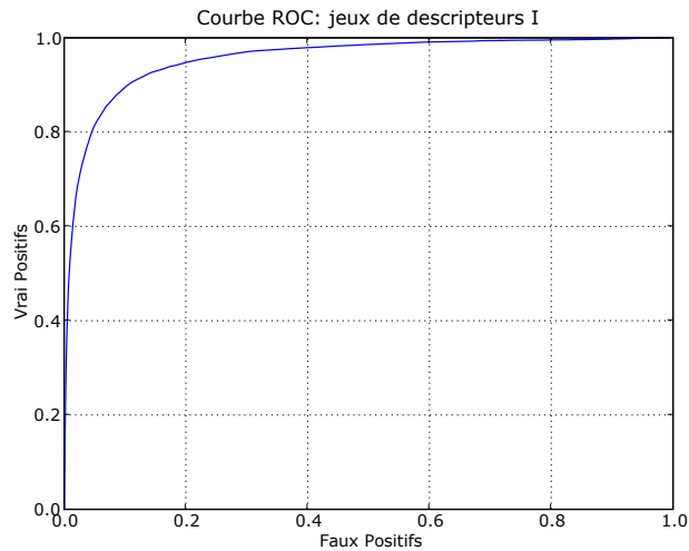
FIG. 9.26: Score du meilleur classifieur. Jeux de paramètres I avec expansion quadratique .
