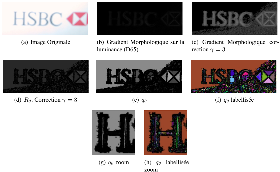
FIG. 7.17: En présence transition (i.e. frontière floue), l'application d'un gradient morphologique de taille unitaire suivi de l'utilisation de l'opérateur de fermeture ultime (ici utilisant un critère de hauteur) n'est pas appropriée.
