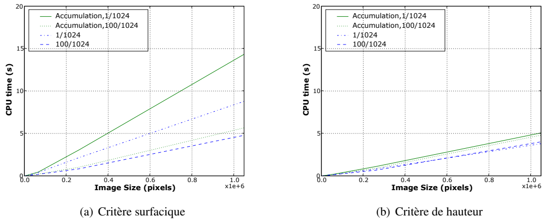
FIG. 8.13: Temps de calcul des algorithmes en fonction de la taille des images pour une même densité de minima. Le seuil d'arrêt de l'algorithme est toujours fixé à sa valeur maximale.
