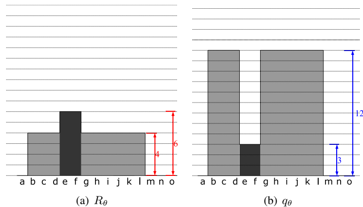
FIG. 7.12: Seconde stratégie de correction de la myopie de l'ouvert ultime pour des transitions graduelles : on propage l'accumulation à l'ensemble de la zone de transition
