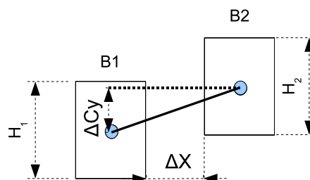
FIG. 9.29: Caractéristiques géométriques utilisées pour la fusion de boîtes
