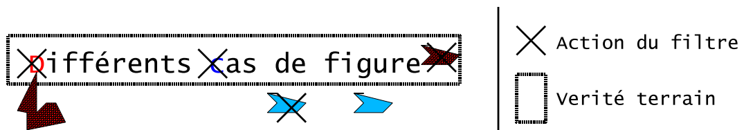
FIG. 9.9: Métrique pour le filtrage grossier : En noir les composantes lettres qui ne sont pas détruites. En bleu les cas correctement traités : la lettre supprimée est comptée comme un faux positif, la composante non lettre et non supprimée est comptée comme un faux négatif. En rouge les biais de la métrique : la composante non lettre est comptée comme un faux positif, la lettre agrégée avec une autre composante n'est pas comptabilisée.
