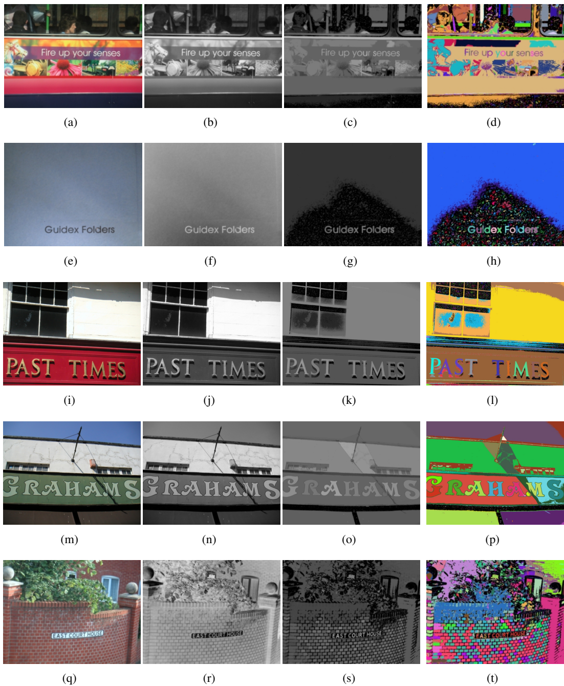
FIG. 7.14: Approche Directe :Utilisation de l'opérateur de fermeture ultime par hauteur. Présentation de segmentation satisfaisante en l'absence de tout autre traitement. De gauche à droite : image originale, canal de luminance pour une polarité du texte, R_\theta (Correction \gamma = 3 ), q_\theta labellisée. Base ICDAR [53]
