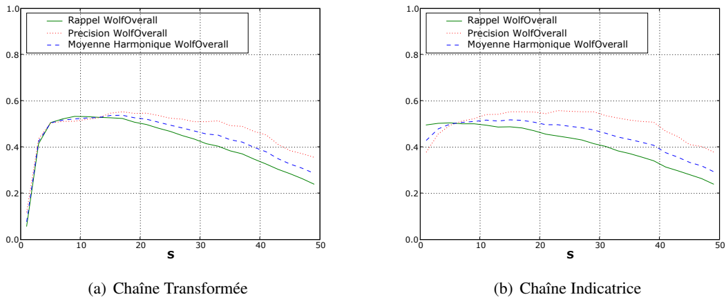
FIG. 10.6: Influence du paramètre S , Seuil bas de la transformée. Pour la chaîne "Transformée" et la chaîne "Indicatrice". Métrique utilisé WolfOverall tr = 0.6 tp = 0.4 (cf. 190).
