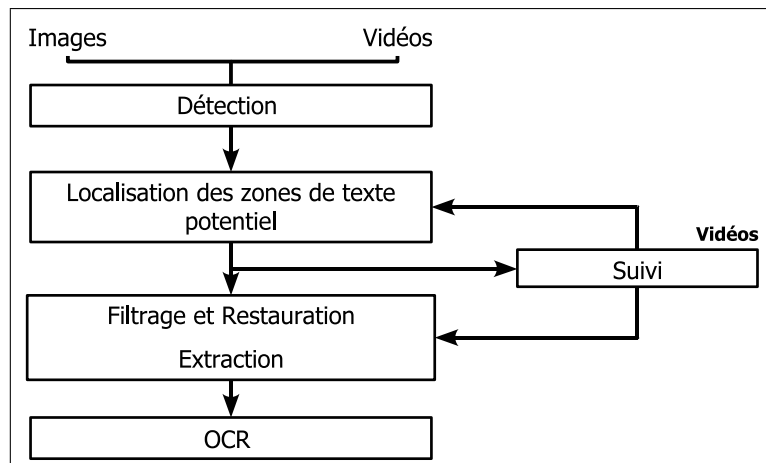
FIG. 2.5: Architecture d'un système d'extraction de texte.
