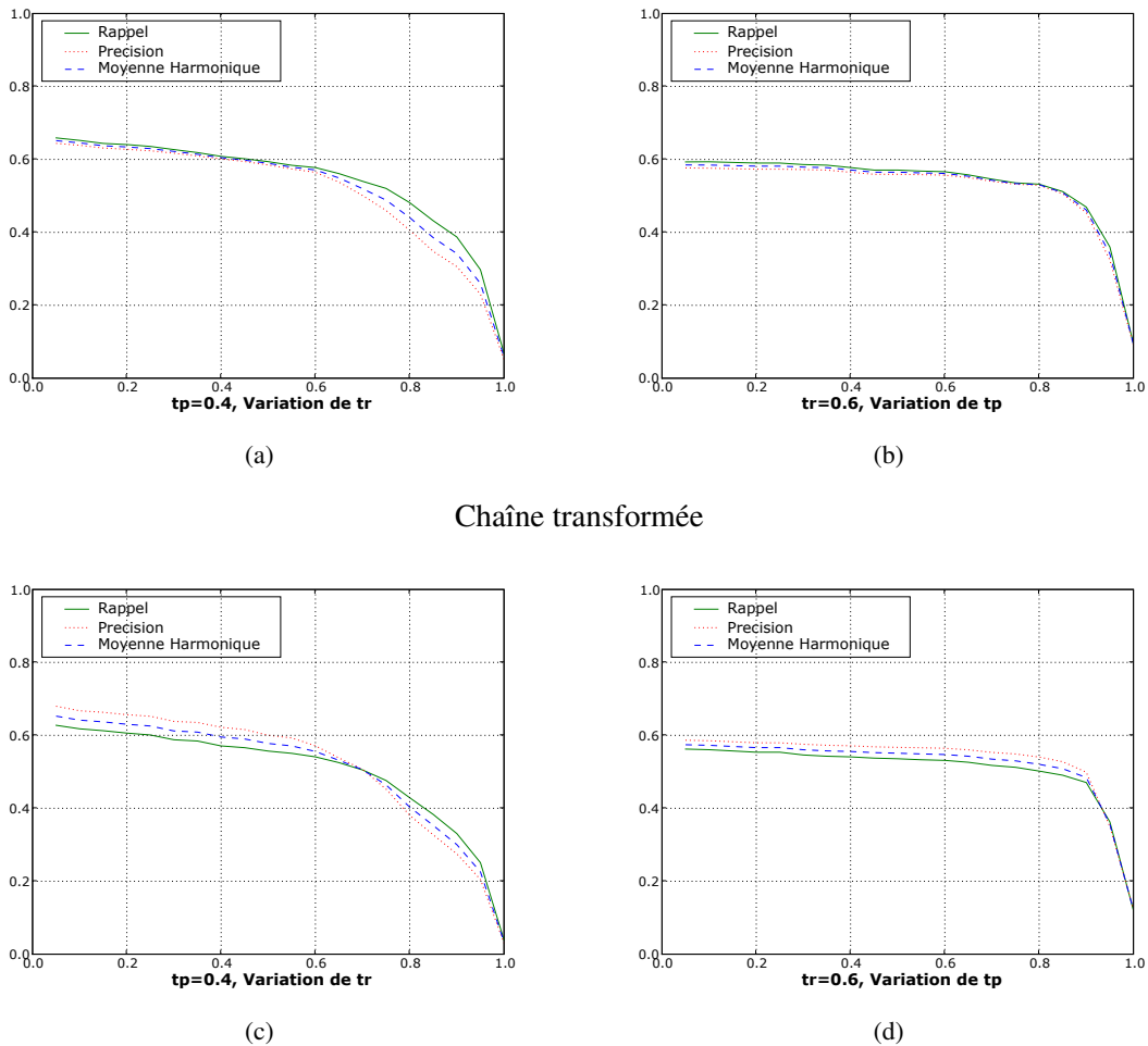
FIG. 10.5: Diagramme de performance sur la base officielle d'ImagEval. Colonne de gauche : variation de la contrainte de rappel tr (avec tp constant et égal à 0.4) ; Colonne de droite : variation de la contrainte de précision tp (avec tr constant et égal à 0.6).
