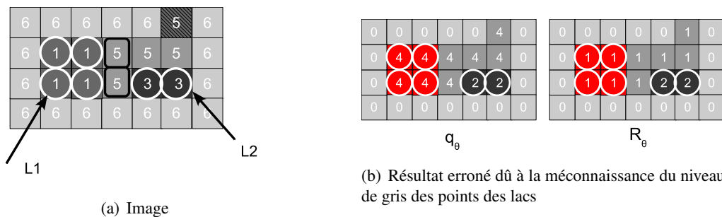
FIG. 8.5: Premier cas de figure : résultat erroné
