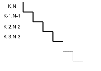
FIG. 8.14: Configuration pour laquelle les algorithmes 8.3.2 et 8.5.1 sont quadratiques
