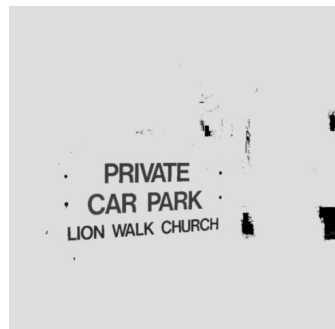
(g) q_\theta
