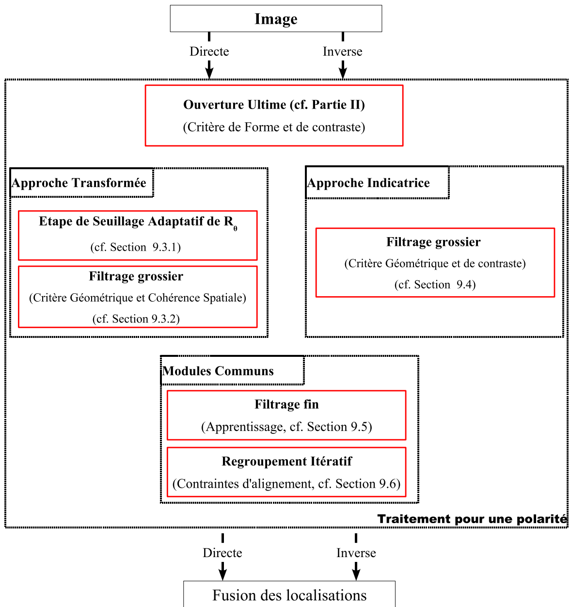
FIG. 9.2: Présentation des chaînes de traitement Transformée et Indicatrice
