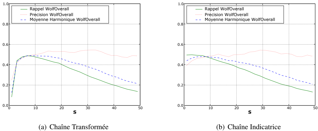
FIG. 10.12: Base ICDAR : Influence du paramètre S , Seuil bas de la transformée. Pour la chaîne Transformée et la chaîne Indicatrice. Métrique utilisée WolfOverall tr = 0.8 tp = 0.4 (cf Section 10.1.2.4).
