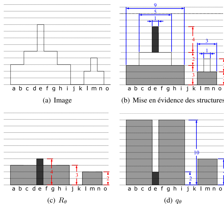
FIG. 6.1: Ouverture Ultime par des segments sur un profil de ligne
