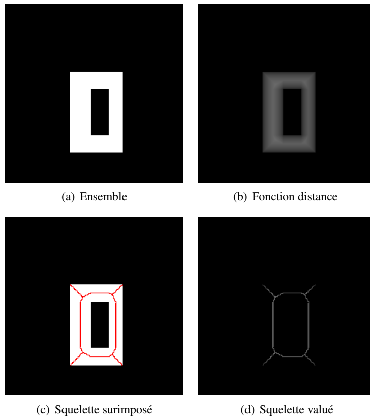
FIG. 9.15: Utilisation du squelette par points d'ancrage (4-connexte) pour la détermination de l'épaisseur et de la consistance de l'épaisseur d'un ensemble.
