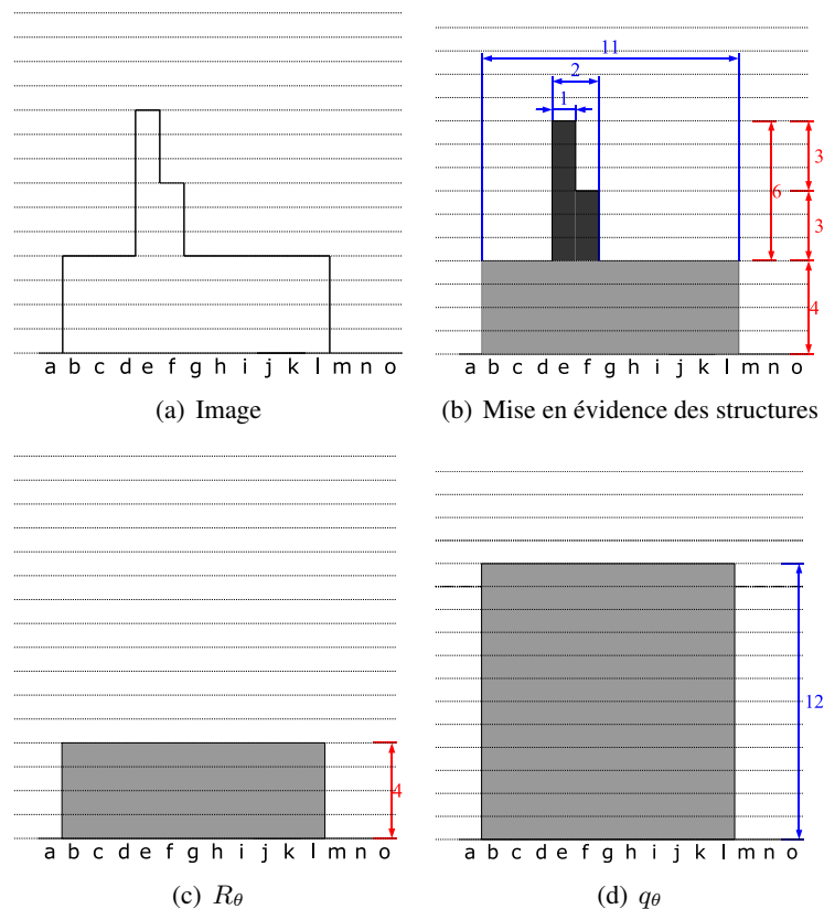
FIG. 7.8: Myopie de l'ouvert ultime pour des transitions graduelles
