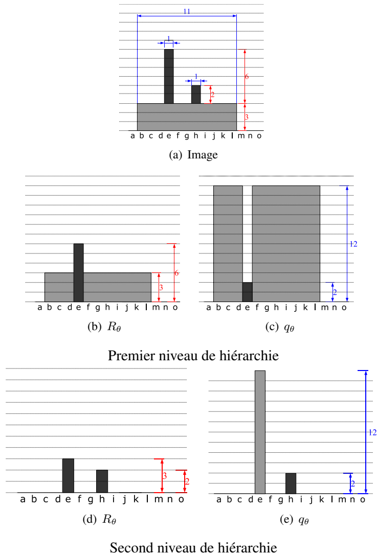
FIG. 7.7: Illustration des deux premiers niveaux d'une hiérarchie de résidus utilisant des ouvertures ultimes surfaciques.
