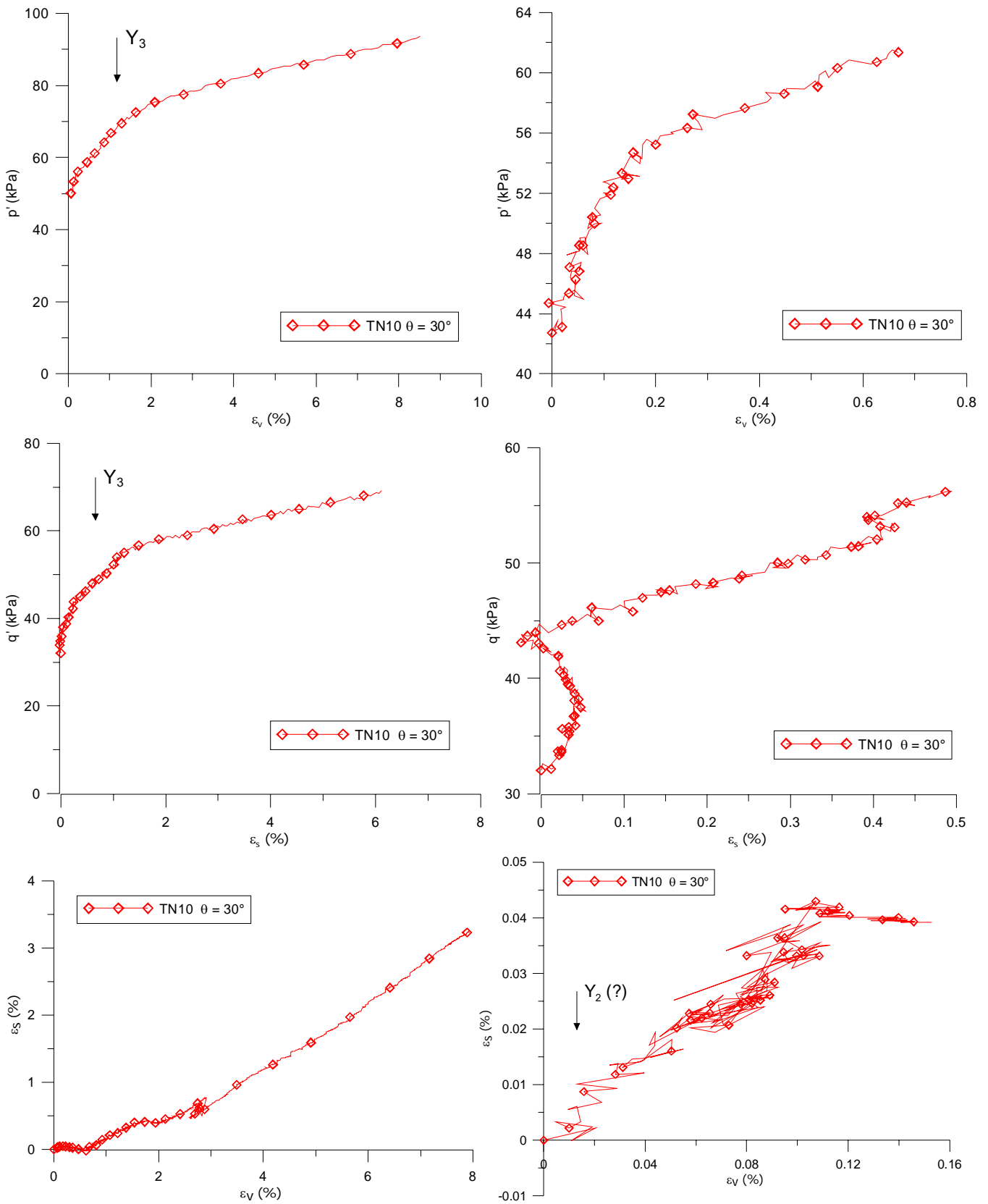
Figure 2 Essai TN10 ( \theta = 30^\circ ) : diagrammes en q - \varepsilon_s ; p' - \varepsilon_v et \varepsilon_s - \varepsilon_v .
