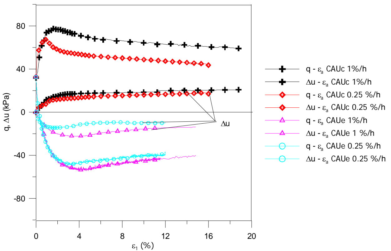
Figure V-41 Effet de la vitesse de cisaillement sur le comportement non-drainé du sol en compression et en extension
