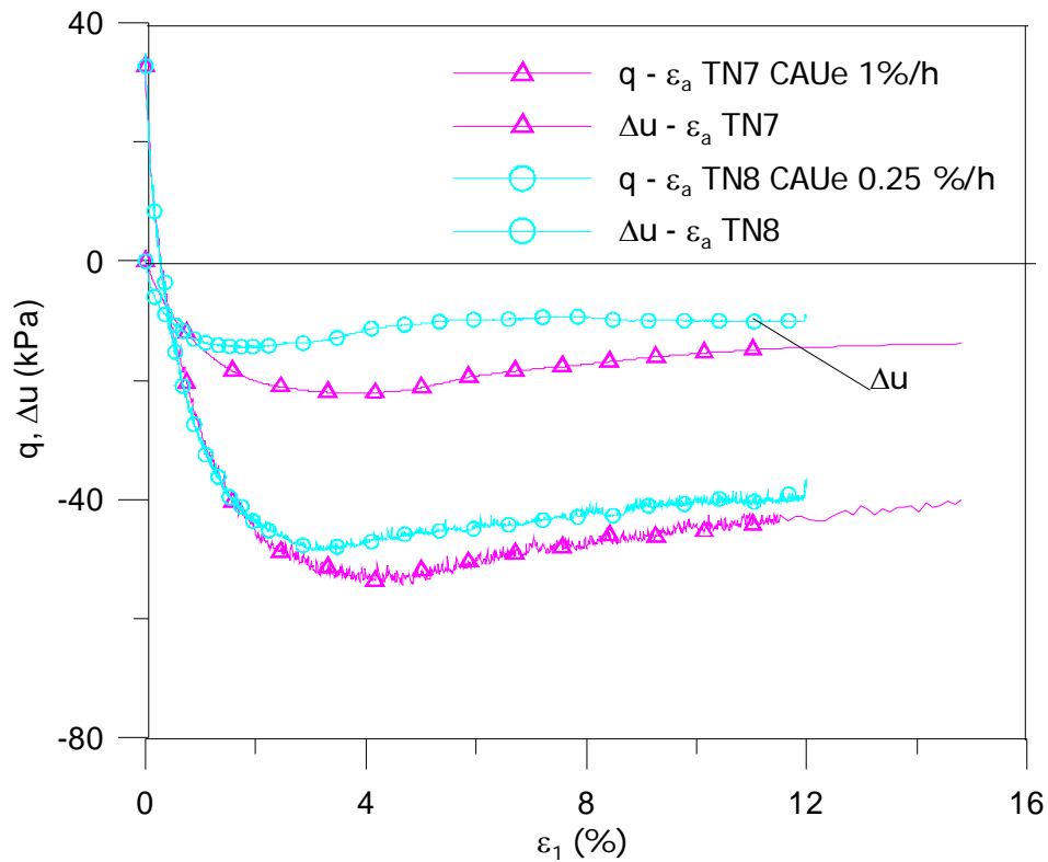
Figure V-40 Effet de la vitesse de cisaillement sur le comportement non-drainé du sol en extension
