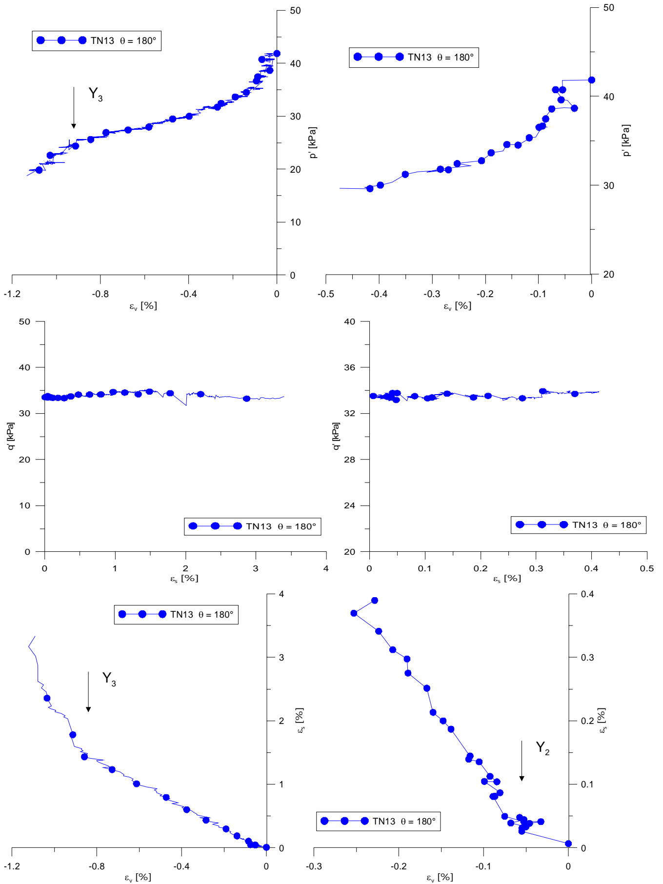
Figure 5 Essai TN13 ( \theta = 180^\circ ) : diagrammes en q - \varepsilon_s ; p' - \varepsilon_v et \varepsilon_s - \varepsilon_v .
