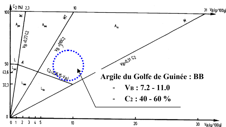
Figure II-31 Classification du LCPC pour les sols fins selon la valeur de bleu et la fraction argileuse (% < 2 \mu m) (Magnan et al., 1989)
