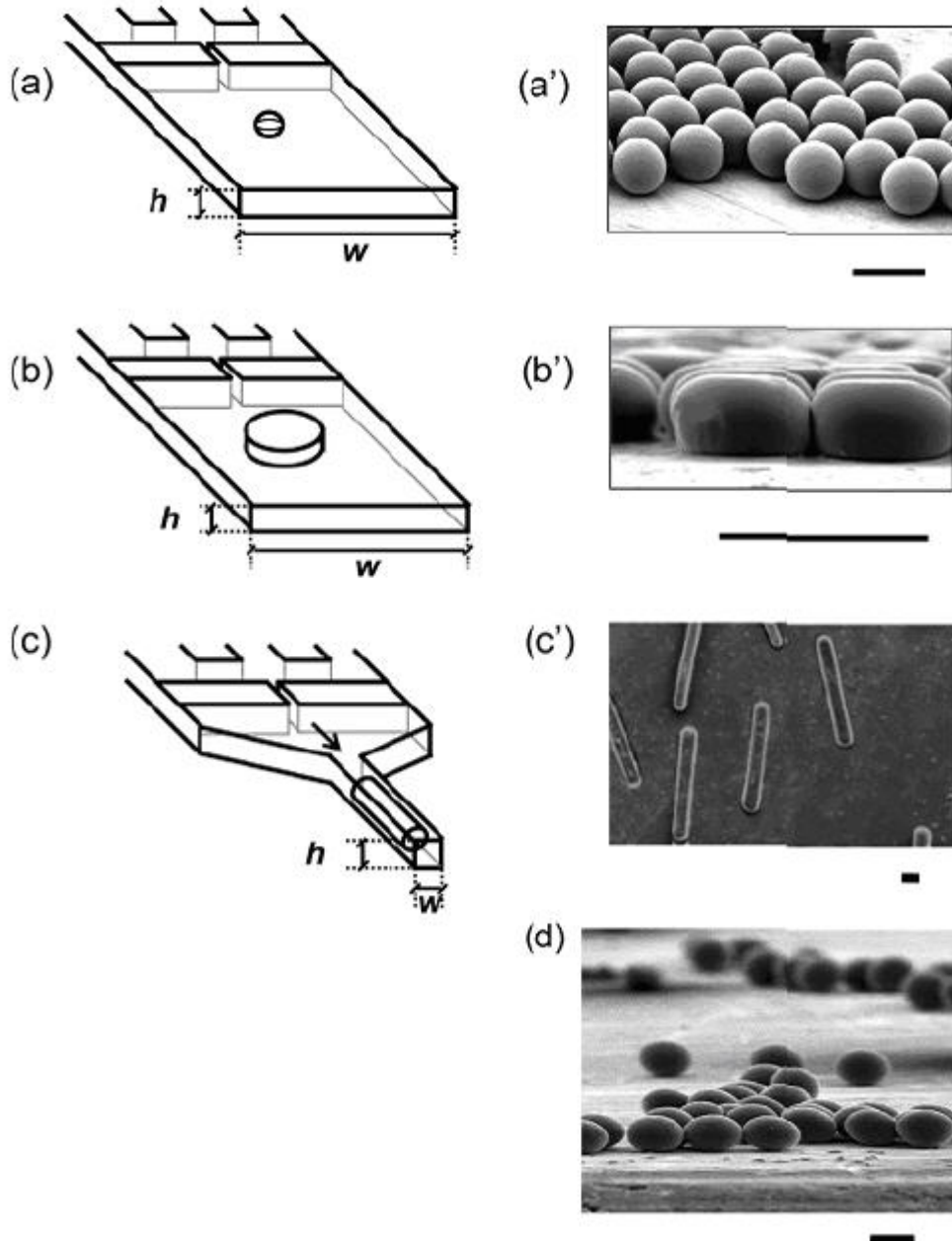
FIG. II.17 – (a, b, c) Schémas des circuits microfluidiques fabriqués avec du poly-(dimethylsiloxane) (PDMS), (a'-c', d) images en microscopie optique montrant différentes formes de particules de poly tri(propylene glycol)diacrylate) obtenues via photopolymérisation de gouttes d'émulsion préparées en microfluidique (échelle 100\mu\text{m} ).
