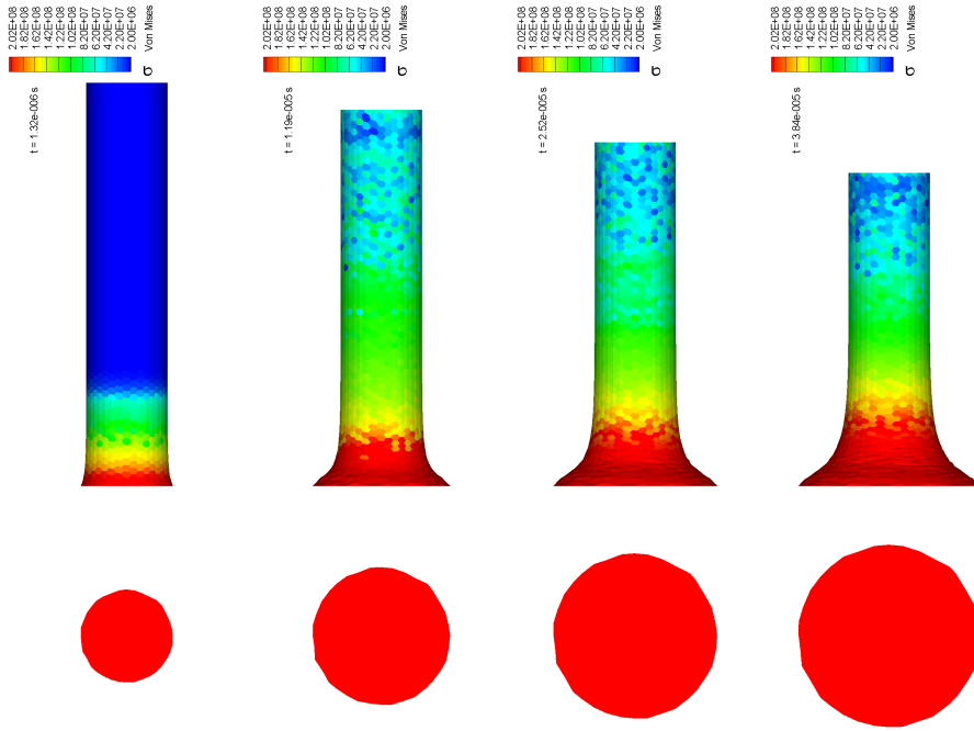
FIG. 5.4 – Barre de Taylor - \sigma Von-Mises - 0s < t < 3,84.10^{-5}s
