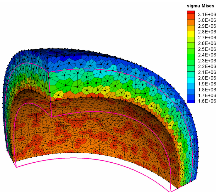
FIG. 4.2 – Contrainte équivalente de Von Mises - \approx 3.500 nœuds ( integration stabilisée - FF Sibson )
