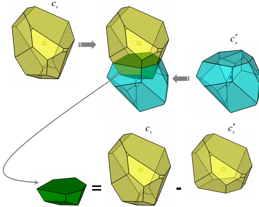
FIG. 3.11 – Etape-2 : Calcul de la mesure de volume du polyèdre P^{int} par le biais du volume complémentaire
