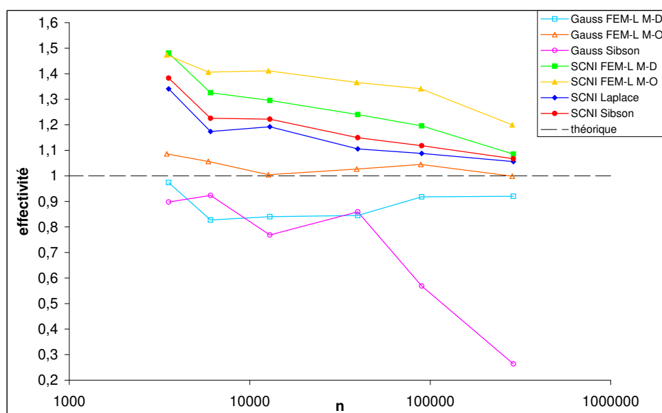
FIG. 4.5 – Courbes d'effectivité ( degré de convergence ) - échelle logarithmique pour le nombre de nœuds
