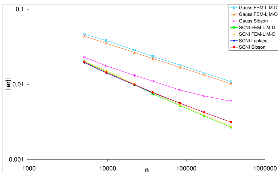
FIG. 4.10 – Courbes de convergence \|e\| = f(nb \text{ nœud}) - double échelle logarithmique
