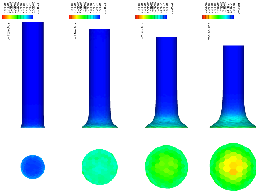
FIG. 5.5 – Barre de Taylor - p - 0s < t < 3,84.10^{-5}s
