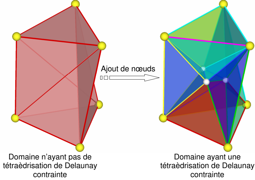
FIG. 2.6 – Tétraèdrisation contrainte de Delaunay du polyèdre de Schönhardt par ajout de nœuds
