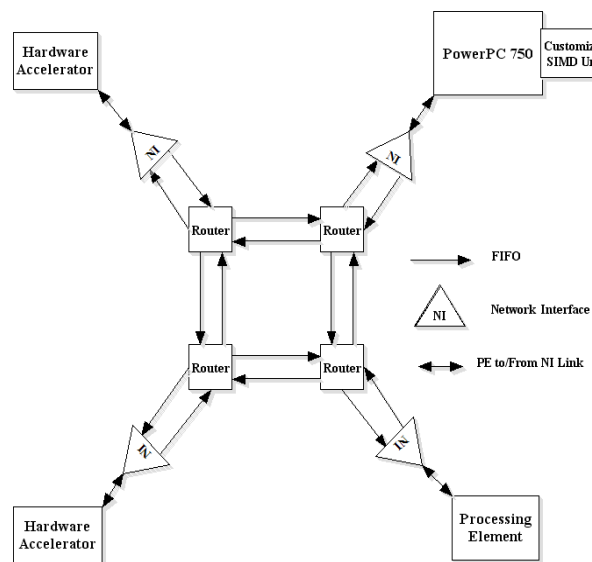
Figure 1-10 Un Réseau sur Puce typique modélisé en utilisant notre système.
