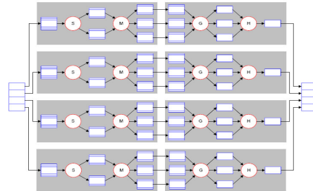
Image 1-11(c) Graphique de Tâches mises à jour d'un Modèle de Half Pipeline
