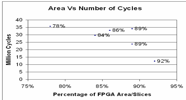
Figure 1-6 Compromis entre Espace et Accélération pour des filtres moyens
