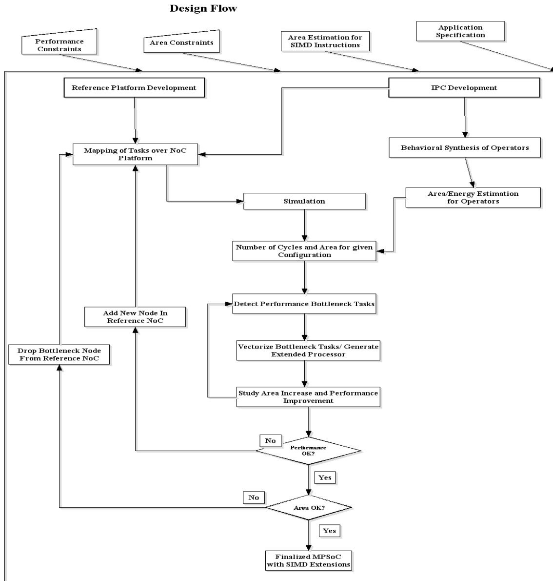
Figure 1-8 Méthodologie de Conception MPSoc pour un Processeur SIMD étendu avec un NoC sous-jacent
