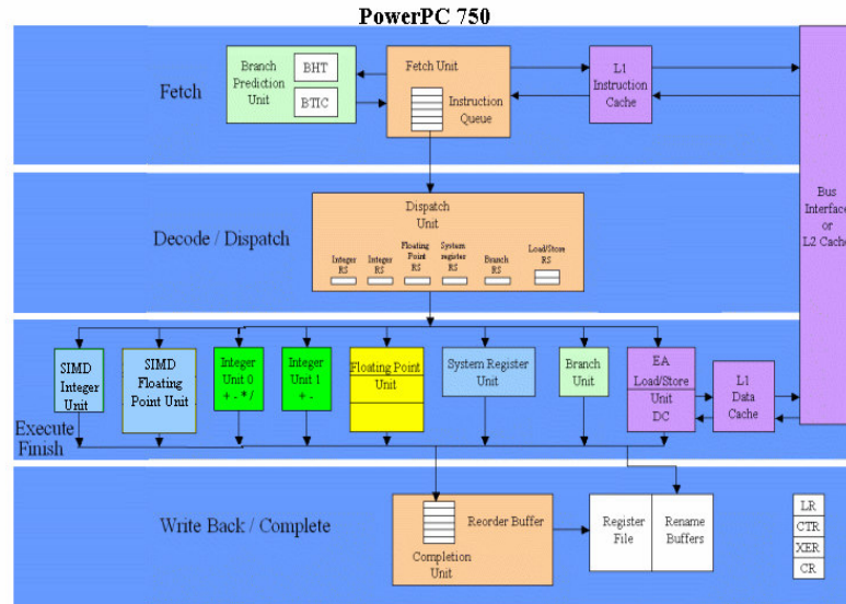
Figure 1-9 PowerPC 750 étendu avec un jeu d'Instruction AltiVec
