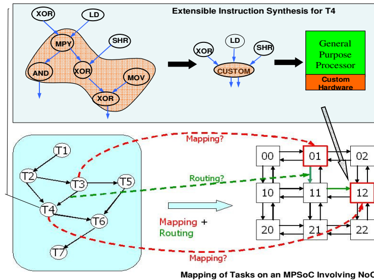
Figure 1-2 Intégration d'Instructions Étendues avec la Synthèse MPSoC en utilisant des Flux de Conception Traditionnels
