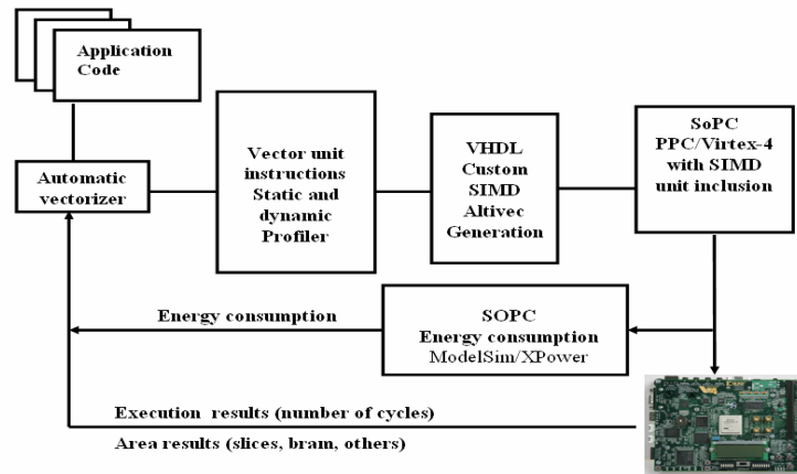
Figure 1-3 Flux de Conception de Système
