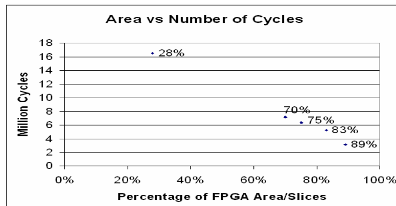
Figure 1-5 Compromis entre Espace et Accélération pour un Programme de Matrice Transposée
