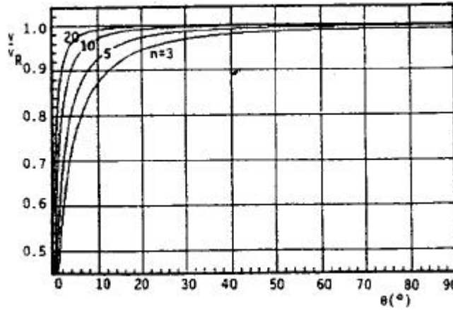
Figure 21 : Vitesse de phase de l'onde de Rayleigh en fonction de l'angle ( q ) pour différents modes( n ) [44].
