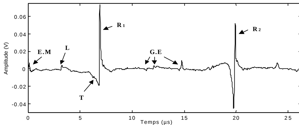
Figure 4 : Agrandissement du premier tour de propagation et identification des ondes engendrées: E.M: onde électromagnétique, L: onde longitudinale, T: onde transversale, R: ondes de Rayleigh, G.E: ondes de galerie à échos.
