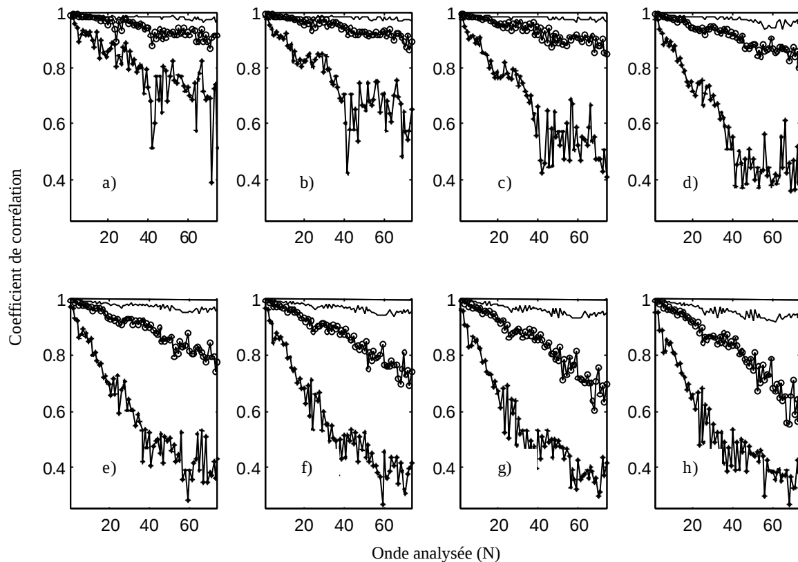
Figure 26 : Evolution de la pente de décorrélation entre deux signaux acquis sur une même pièce en fonction de la bande de fréquence analysée (- sain, -o- d = 0,08 mm, -- d = 0,14 mm).
