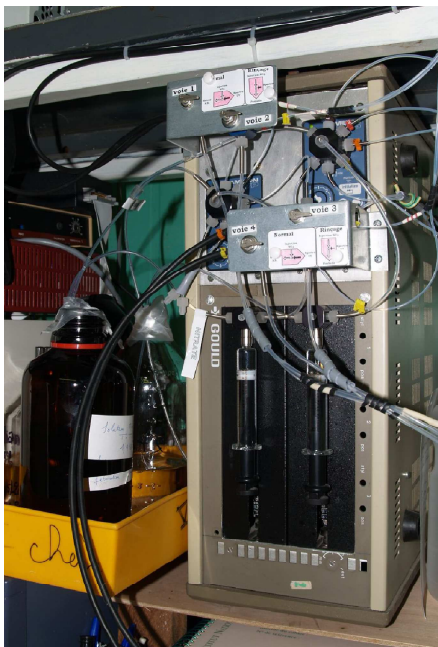
FIG. 6.3: Vue détaillée de l'automate de régulation des solutions nutritives : Pousse-seringues et vannes de distribution de solutions-mères.
