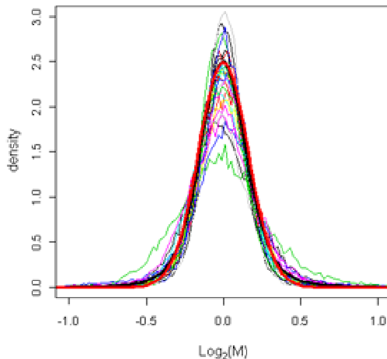
FIGURE 2.5: La transformation et la normalisation des données permettent de travailler sur des distributions comparables et proches d'une distribution gaussienne. En rouge et en gras est représentée une courbe de Gauss, en couleurs et en trait fin sont représentées les distributions des rapports des 28 puces.
