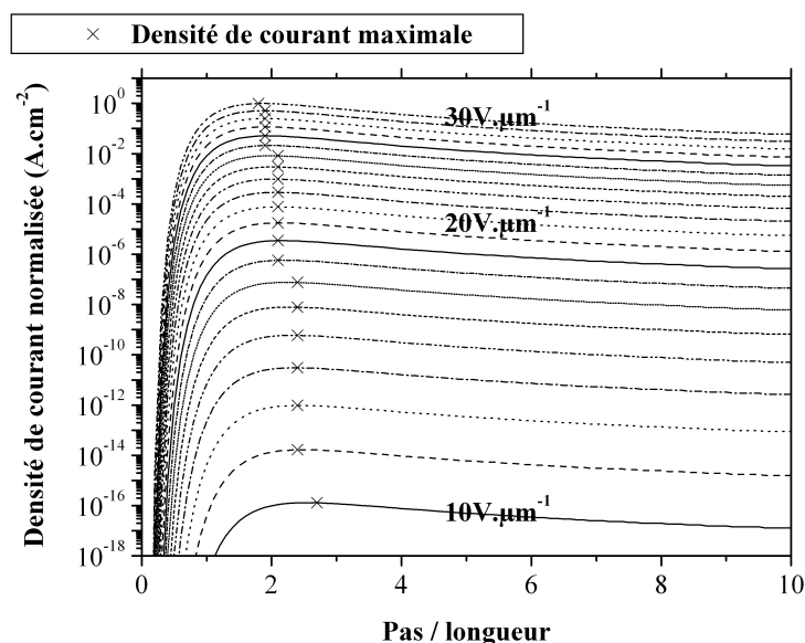
Figure 2-24: Densité de courant normalisée en fonction du rapport pas/longueur.
