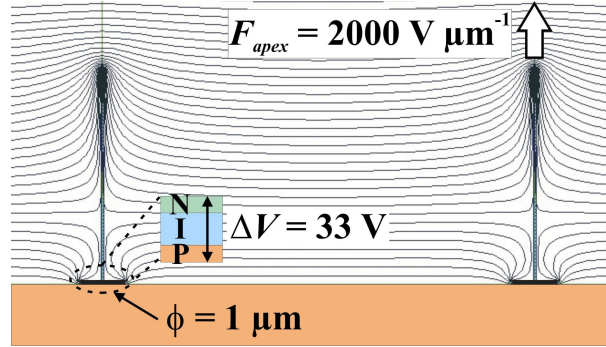
Figure 4-7 : Photocathode sous éclairage faible ou nul avec chute de potentiel de 33 V, U = 2000\text{ V} .
