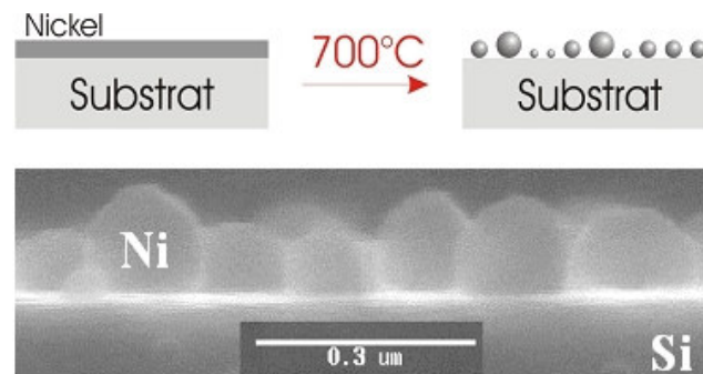
Figure 2-25: Formation des agrégats de nickel à 700^\circ\text{C} et images de celle-ci sur un substrat de silicium.
