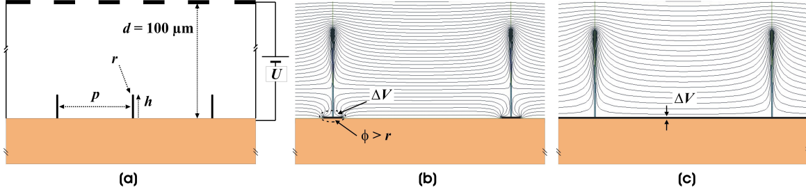
Figure 4-3 : (a) Configuration de base, (b) influence sur les lignes équipotentiellles d'une chute de potentiel localisée, (c) influence sur les lignes équipotentiellles d'une chute de potentiel étendue.
