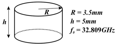
Figure 3-19 : Premier pré-dimensionnement des cavités 32 GHz.
