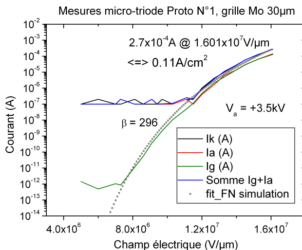
Figure 3-35 : Mesures DC dans la configuration triode.
