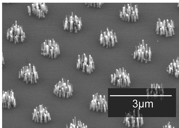
Figure 2-28: Croissance en utilisant une barrière de diffusion.
