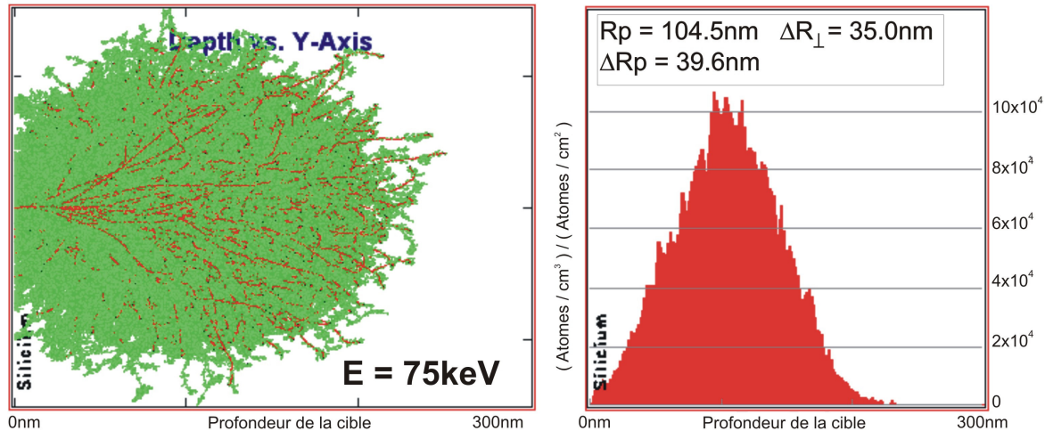
Figure 4-24 : Simulation SRIM : ions Phosphore dans Silicium, E = 75 keV.
