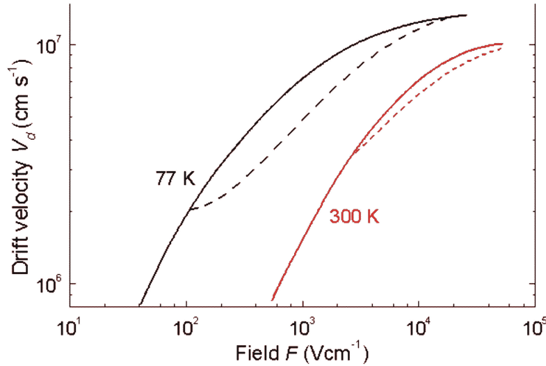
Figure 4-68 : Vitesse des porteurs dans le Silicium en fonction du champ électrique.
