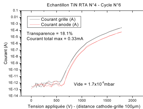
Figure 3-49 : Résumé des mesures obtenues en mode triode sur un échantillon TiN RTA (N°4).
