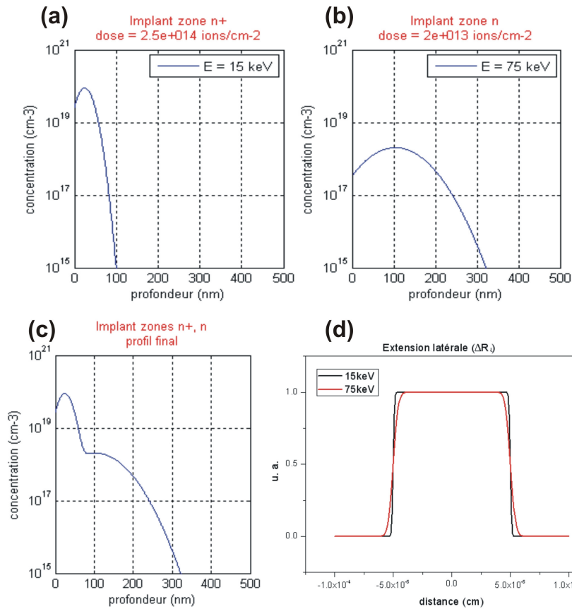
Figure 4-26 : Profil finale d'implantation
