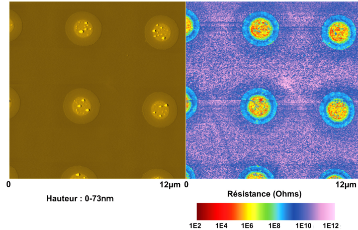
Figure 4-39 : Mesure AFM d'un réseau de plots TiN/Ni recuit 700°C – 20 min + 850°C – 10 min (image réalisée à – 2 V sur la pointe).
