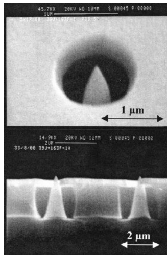
Figure 2-10: Réseau de pointes Spindt.
