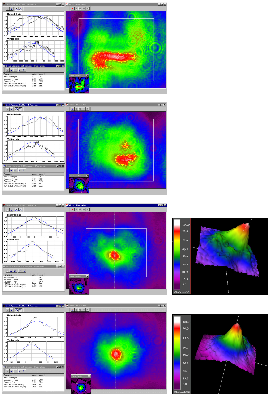
Figure 4-49 : Figures présentant l'allure du spot laser pour les puissances suivantes :290 mW, 400 mW, 500 mW et 520 mW.
