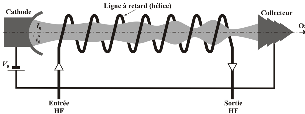
Figure 1-9 : Théorie du tube à onde progressive : schéma du tube et notations.
