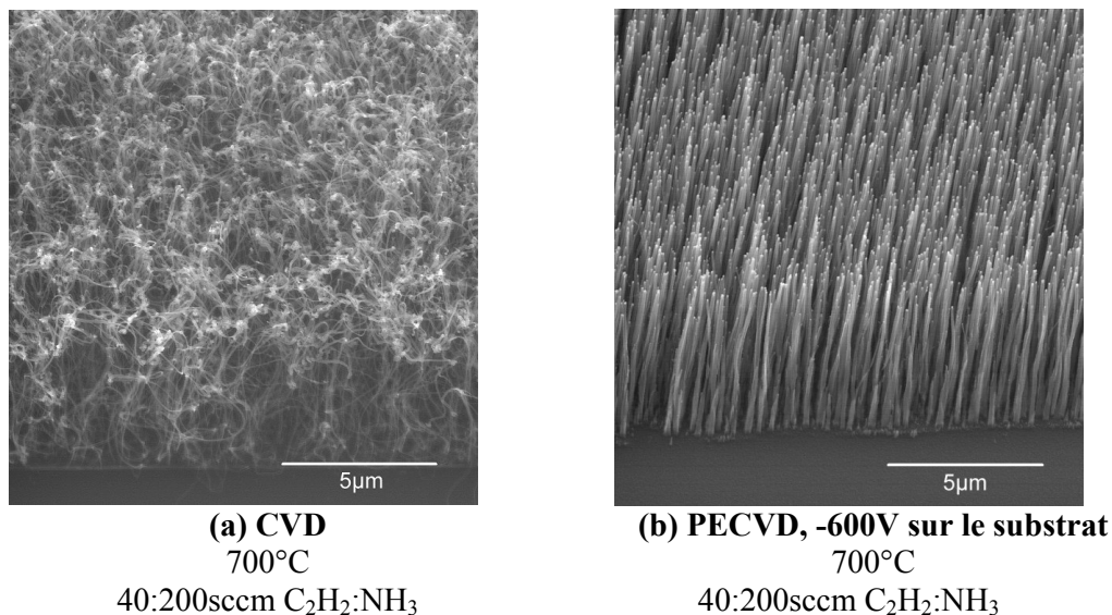
Figure 2-17 : (a) Croissance sans plasma. (b) Croissance avec plasma, alignement des nanotubes.
