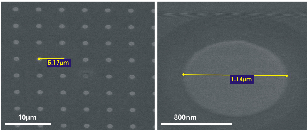
Figure 4-31 : Photos MEB de plots TiN/Ni sans recuit.
