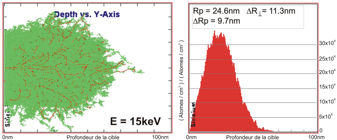
Figure 4-25 : Simulation SRIM : ions Phosphore dans Silicium, E = 15 keV.
