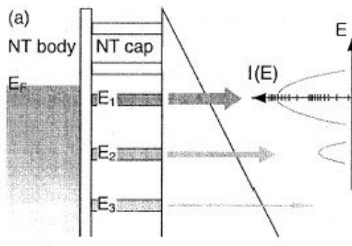
Figure 2-6: Des états localisés à l'extrémité des nanotubes induisent plusieurs pics dans la distribution en énergie.
