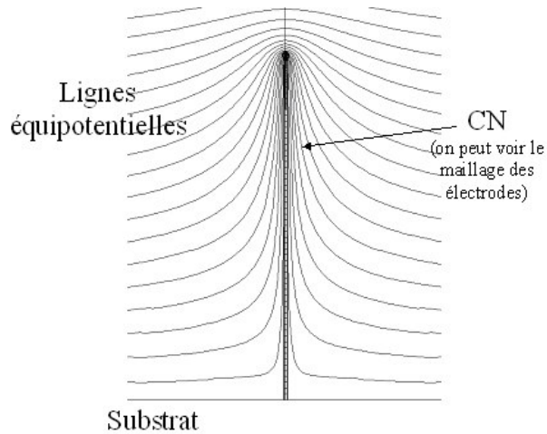
Figure 2-20: Simulation d'un nanotube de carbone soumis à un champ électrique. On peut distinguer le maillage du nanotube en plusieurs électrodes élémentaires.
