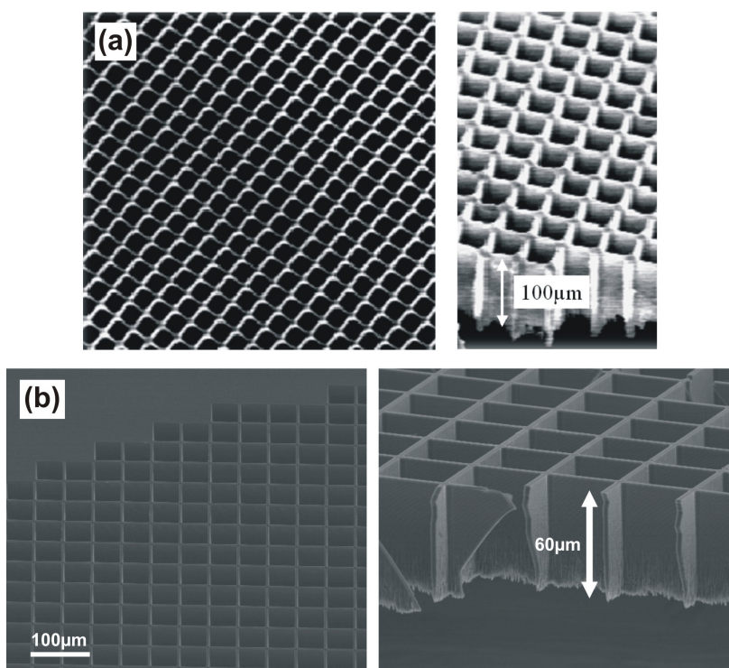
Figure 4-47: Grille d'extraction en silicium d'épaisseur 100 \mu\text{m} avec des ouvertures de 18 \mu\text{m} au pas de 20 \mu\text{m} (a), et d'épaisseur 60 \mu\text{m} avec des ouvertures de 45 \mu\text{m} au pas de 50 \mu\text{m} (b).
