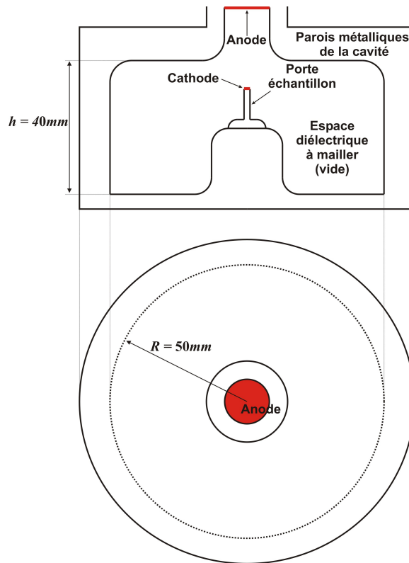
Figure 3-4 : Schéma de la cavité réentrante 1.5 GHz.
