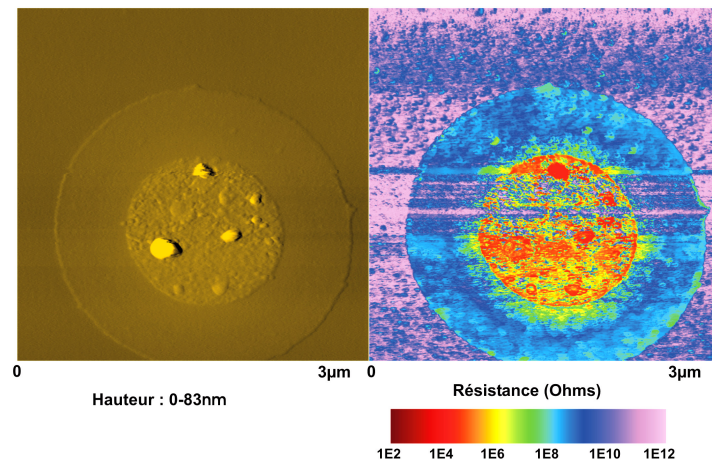
Figure 4-40 : Mesure AFM d'un plot TiN/Ni recuit 700°C – 20 min + 850°C – 10 min (image réalisée à –2 V sur la pointe).
