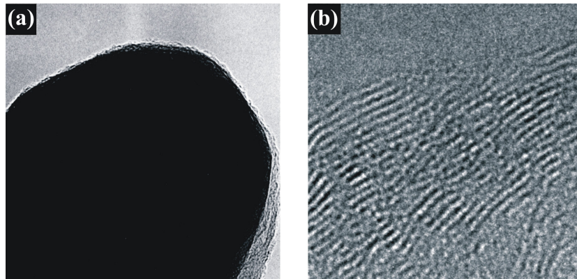
Figure 2-36: (a) Extrémité et (b) parois d'un nanotube de carbone après croissance par PECVD @ 700°C.
