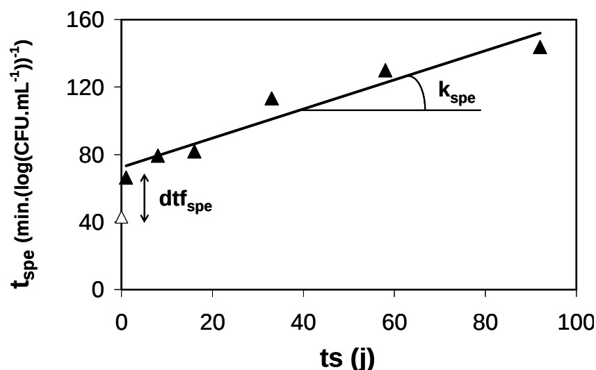
Figure II.4 : schéma de la méthode de quantification de la perte d'activité acidifiante spécifique des ferments lactiques pendant la congélation et au cours du stockage à l'état congelé de Lb. bulgaricus CFL1
