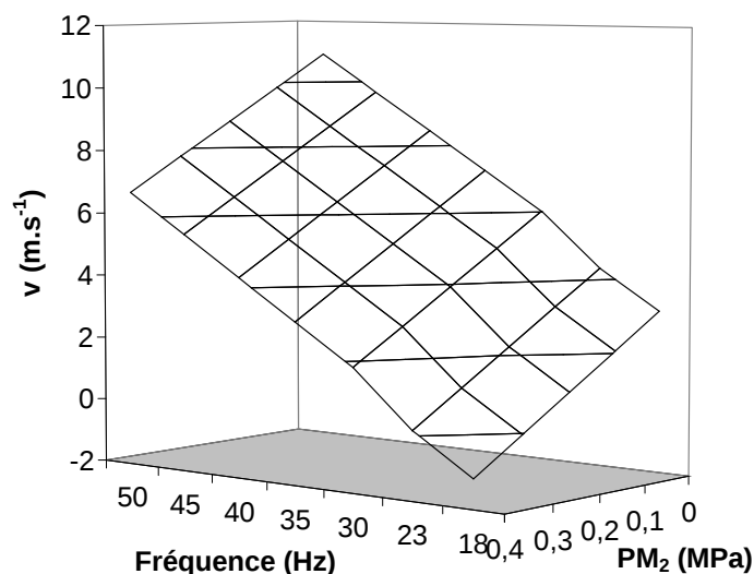
Figure II.9 : représentation tridimensionnelle du polynôme caractérisant la vitesse tangentielle ( v ) en fonction de la fréquence de pompage ( F ) et de la pression à la sortie du système ( PM_2 ).
