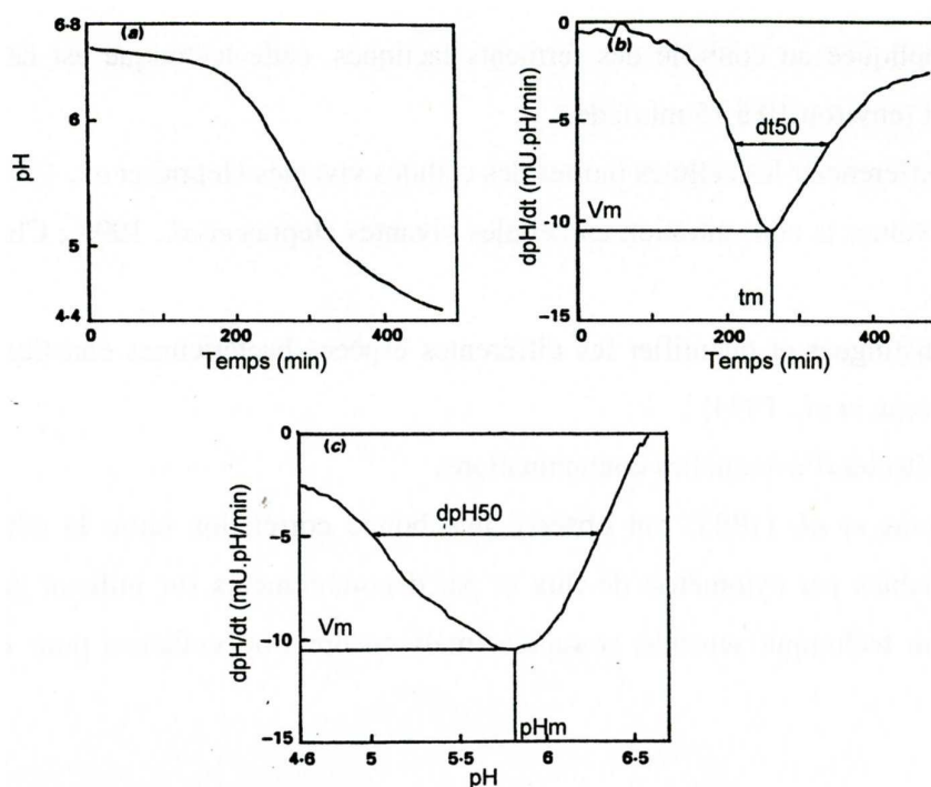
Figure I.2 : évolution du pH et de la vitesse d'acidification ( dpH/dt ) lors de l'incubation de Lactobacillus bulgaricus CNRZ 398 dans du lait à 40 °C (d'après Spinnler et Corrieu, 1989)
