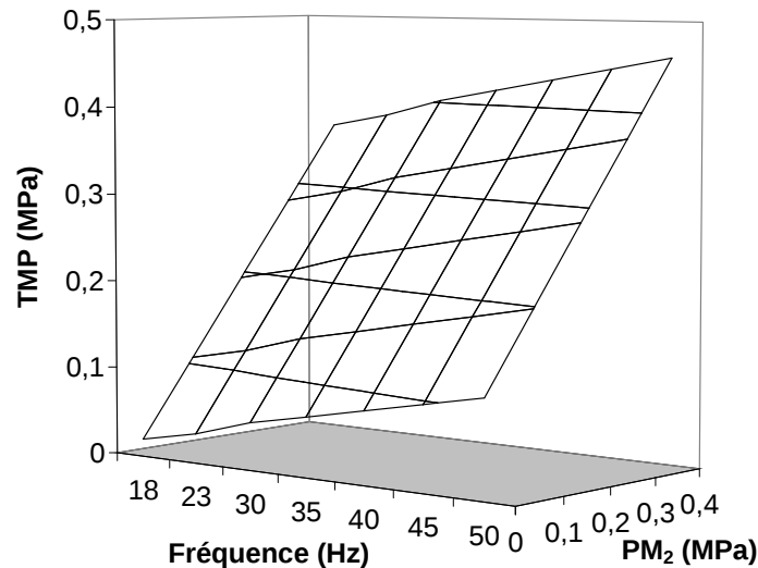
Figure II.8 : représentation tridimensionnelle du polynôme caractérisant la pression transmembranaire (TMP) en fonction de la fréquence de pompage (F) et de la pression à la sortie du système ( PM_2 ).
