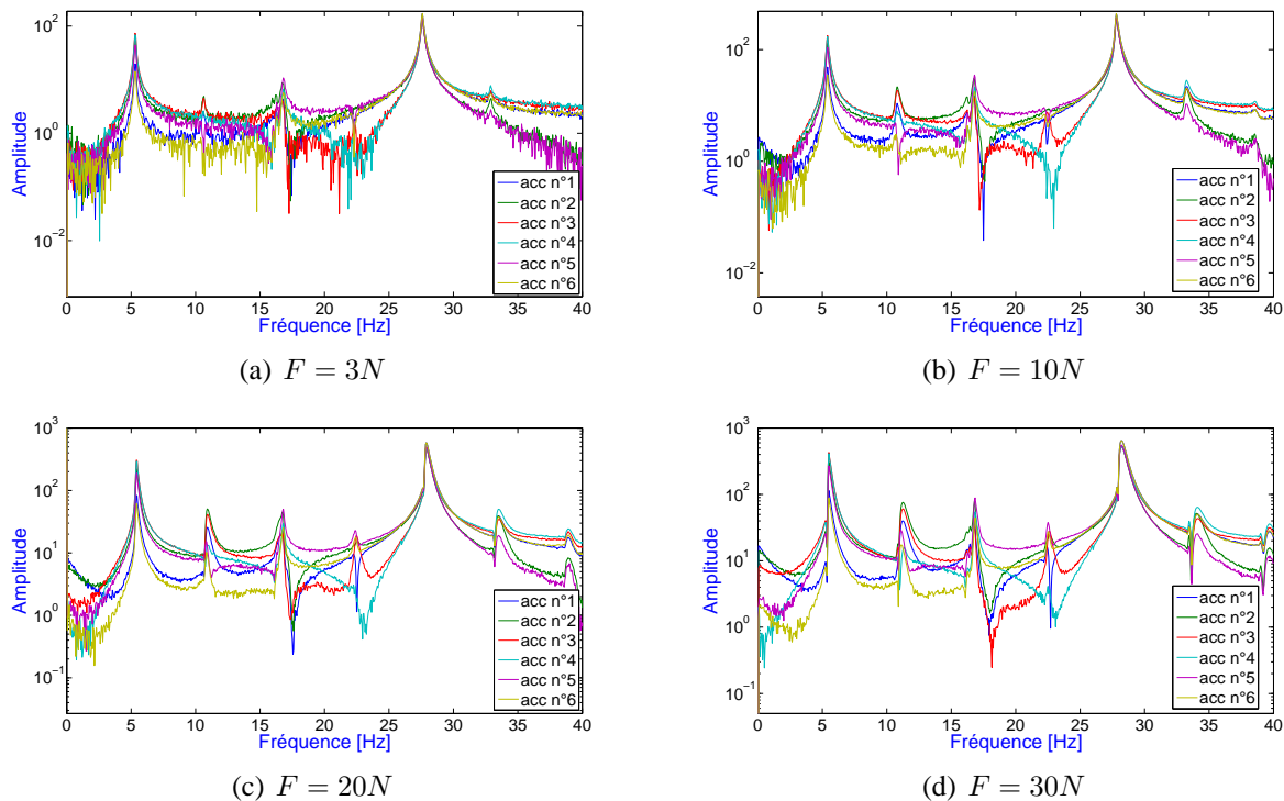
FIGURE 8.29: TF obtenues à partir des signaux de mesure des accéléromètres pour la poutre E-E pour différents niveaux de force et pour une excitation à l'abscisse x_0=0.85 m .
