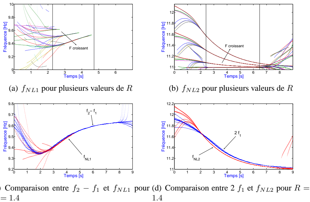
FIGURE 8.27: Comparaison des arêtes obtenues à partir de la TOC pour les deux premiers pics supplémentaires et les combinaisons de fréquences correspondantes ( f_2 - f_1 et 2 f_1 ) avec les ELB-CA et différents rapports R = 1.4 .
