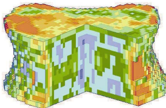
Figure 7. Modèle en éléments finis personnalisé de corps vertébral mis en place à partir de tomographie quantitative. Chaque élément correspond à un voxel de la reconstruction tomographique (taille 1x1x1,5 mm 3 ). [CRAW03a]
