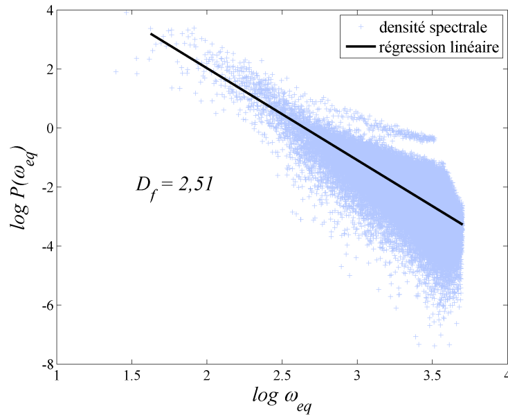
Fig. 3.13: Densité spectrale P de la surface sablée -
