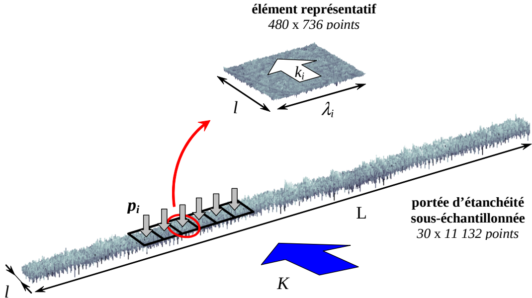
Fig. 5.13: Calcul de la transmissivité sur toute la portée d'étanchéité par découplage des échelles microscopiques et macroscopiques -
