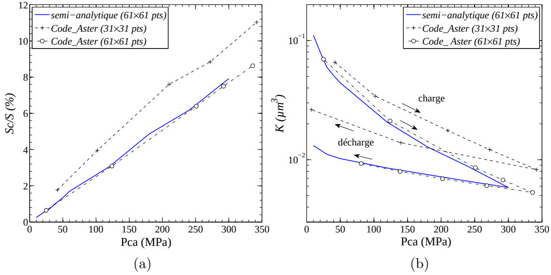
Fig. 5.17: Comparaison entre les résultats obtenus avec le code semi-analytique ( p_{lim} = 4500 MPa) et Code_Aster ( S_Y = 1500 MPa) : évolution (a) des aires de contact Sc/S et (b) des transmissivités K en fonction de la pression de contact apparente Pca -
