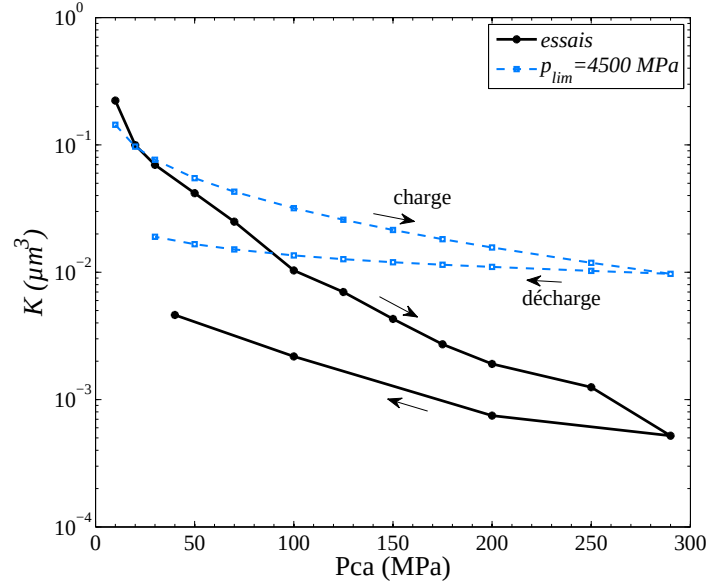
Fig. 5.3: Comparaison entre les mesures et les calculs de K effectués sur l'éprouvette 2 (42CD4) avec p_{lim} = 4500 MPa -
