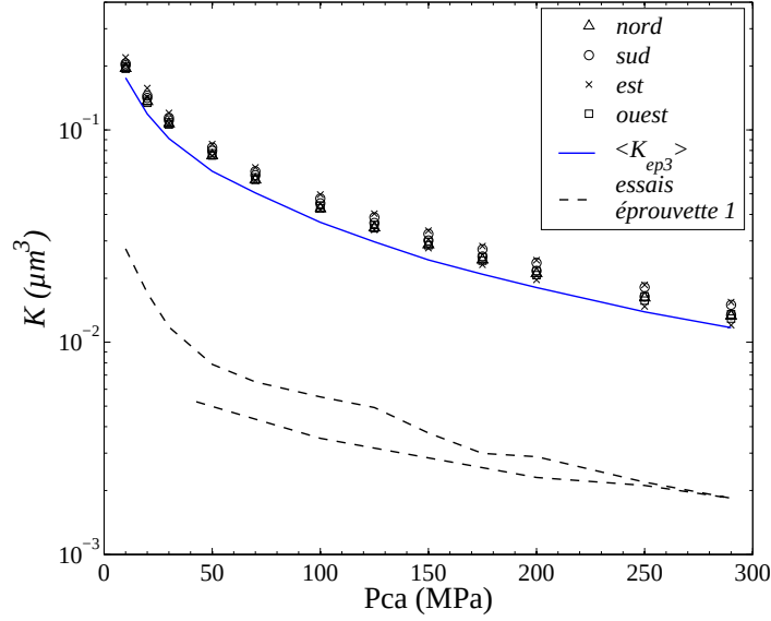
Fig. 5.4: Transmissivités K calculées sur les quatre relevés de l'éprouvette 3 (Stellite) avec p_{lim} = 4500 \text{ MPa} (symboles), moyenne des transmissivités \langle K_{ep3} \rangle calculées sur l'éprouvette 2 (ligne continue) et transmissivités mesurées sur l'éprouvette 3 (pointillés)
