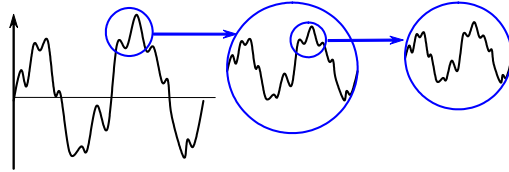
Fig. 3.7: Concept d'auto-similarité -
