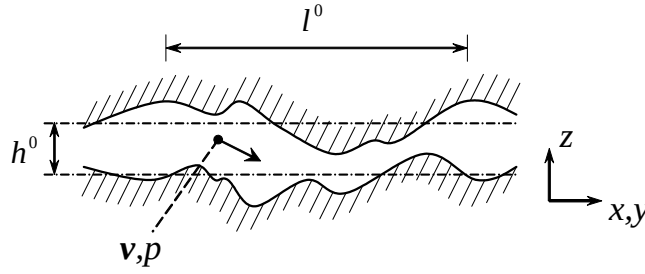
Fig. 2.2: Fracture rugueuse -
