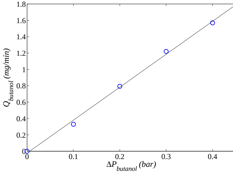
Fig. 4.8: Évolution du débit de fuite massique Q_{butanol} en fonction de la pression relative de butanol \Delta P_{butanol} pour l'éprouvette 3 et pour une pression de contact P_{ca} = 20 \text{ MPa} -
