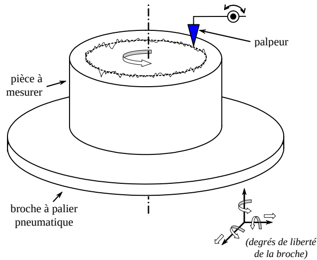
Fig. 5.10: Principe de la mesure des défauts d'ondulation par palpage mécanique -
