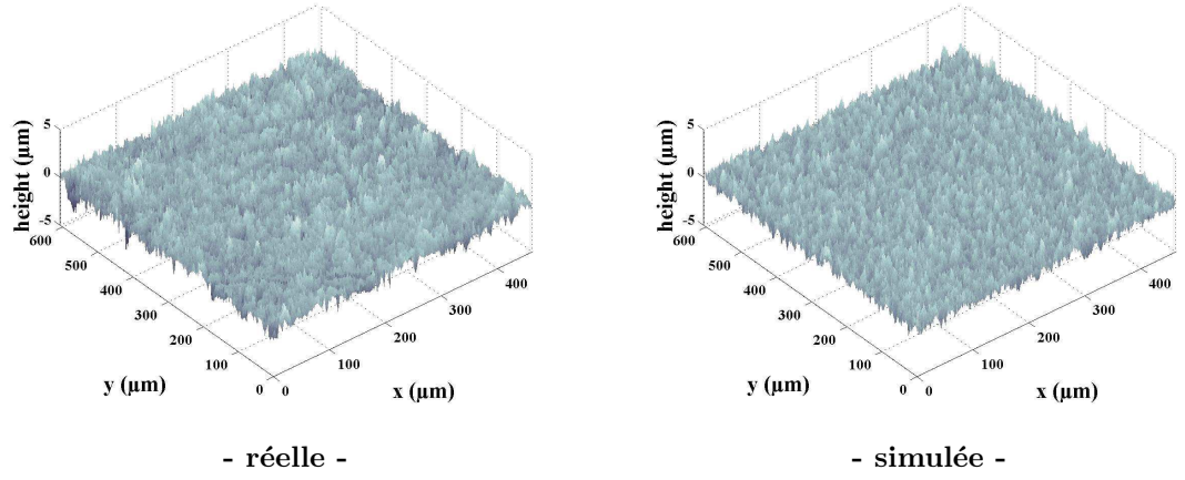
Fig. 3.17: Textures des surfaces rodées -
