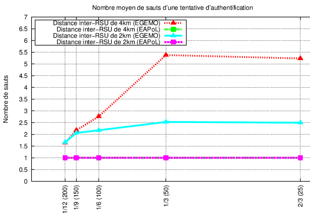
Figure 7: Nombre de sauts d'une tentative d'authentification
