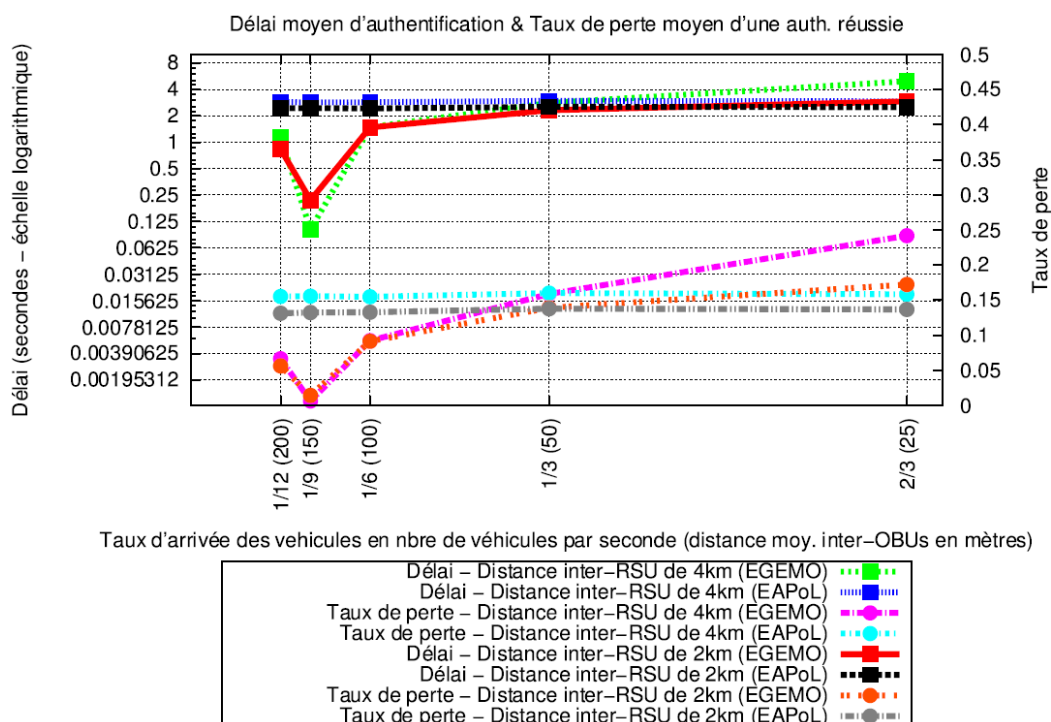
Figure 4: Délai d'authentification et Taux de perte d'une authentification réussie
