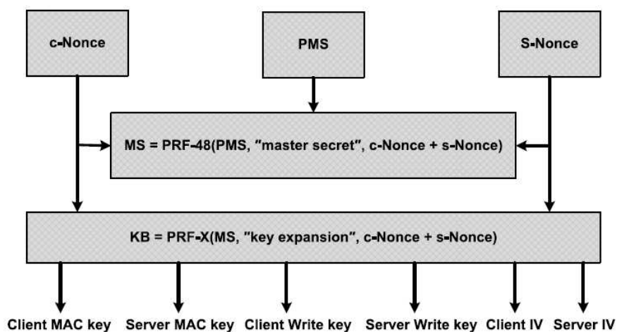
Figure 9: Hiérarchie des clés AUCRED [TLS]
