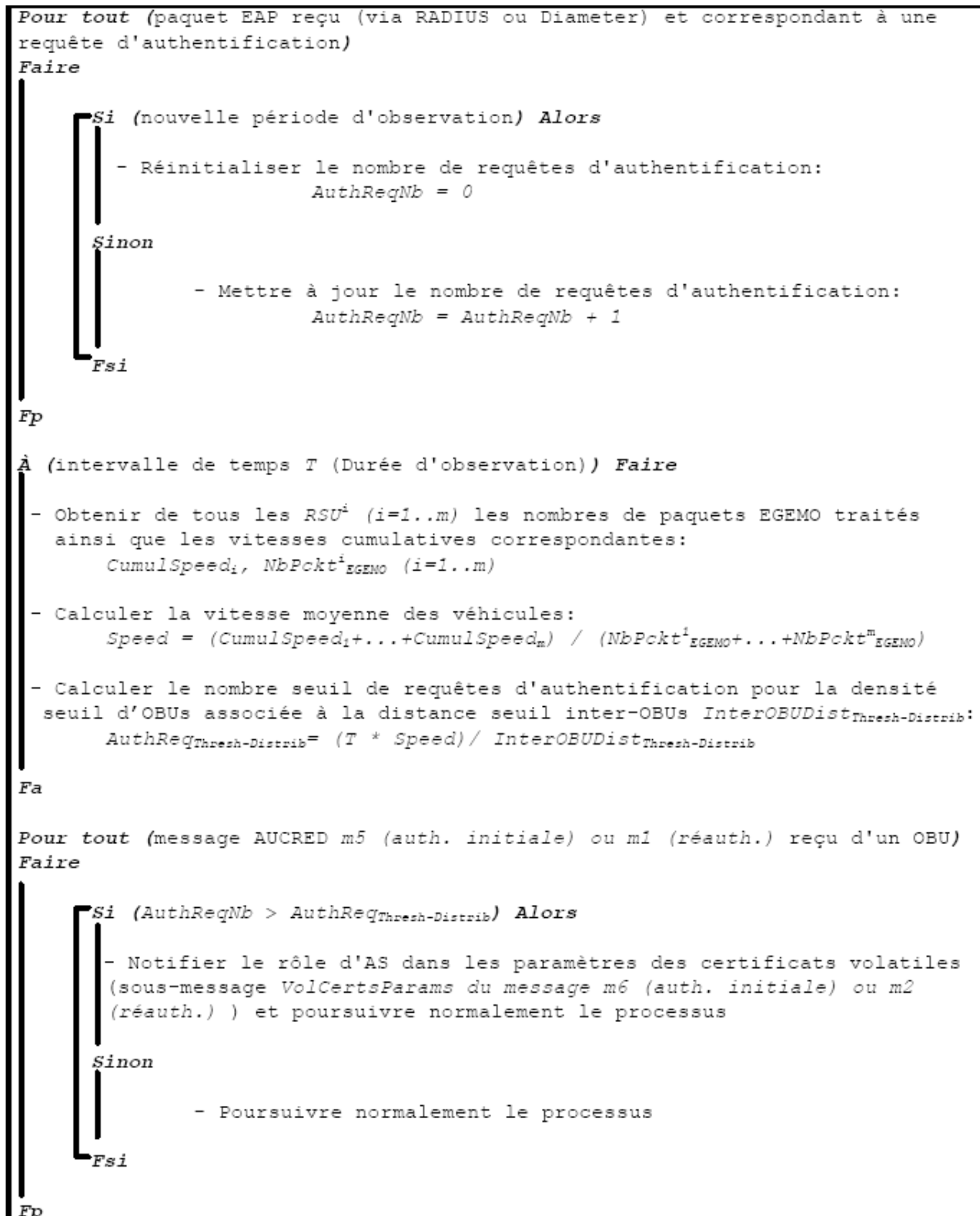
Figure 3: Pseudo-code de l'AS pour la distribution de l'authentification
