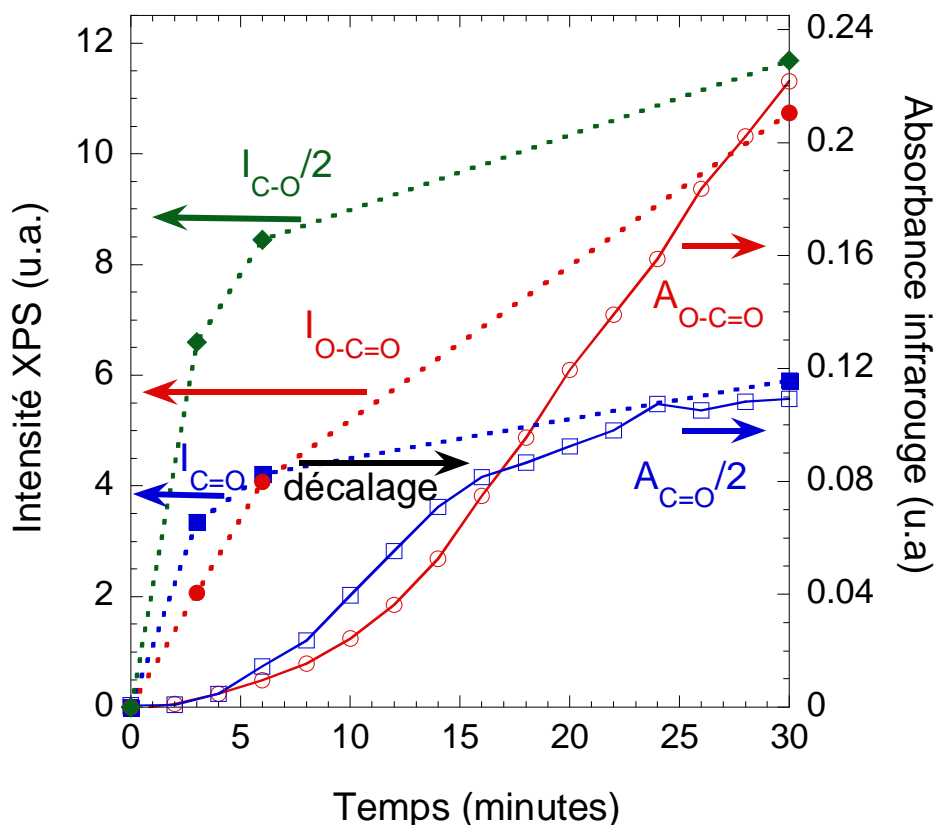
Figure 4.15 : Evolution comparée des ajustements des pics associés aux différentes fonctions carbonées hydrophiles obtenus par les spectroscopies infrarouge et XPS.
