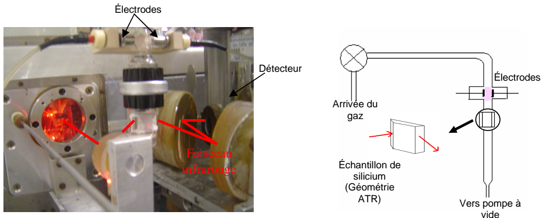
Figure 4.1 : Photos et schémas de la cellule utilisée.
