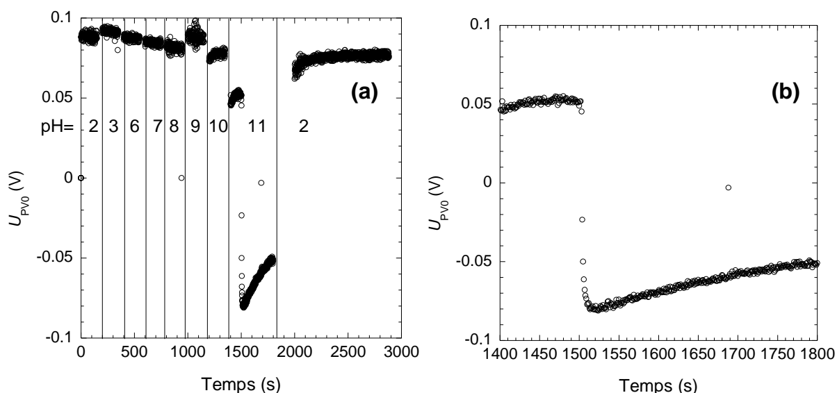
Figure 2.20 : Variation du photopotentiel de surface U_{PV0} à différents pH (tampons phosphates et borates, 10^{-2} \text{ mol.L}^{-1} ) pour des couches acides greffées sur du silicium de type p (résistivité 1000\text{-}3000 \Omega \text{ cm} ) (a) à différents pH (b) zoomé sur la zone à pH 11 .
