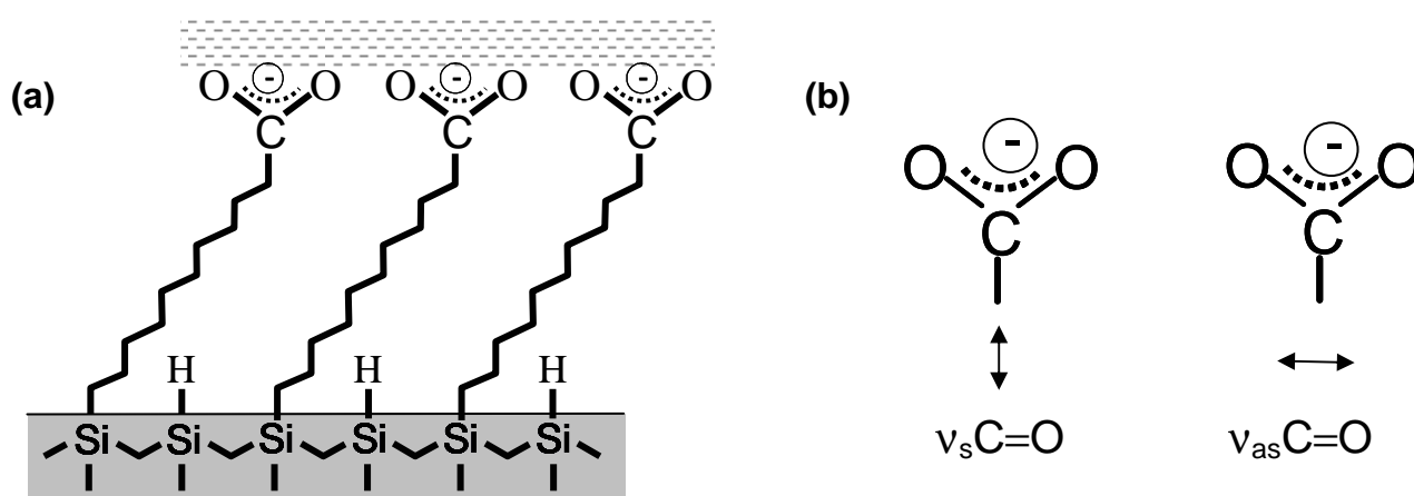
Figure 3.12 : (a) Orientation des groupements \text{COO}^- en contact avec l'électrolyte. (b) Modes d'élongation des liaisons CO. Les flèches indiquent les directions des dipôles dynamiques associés.
