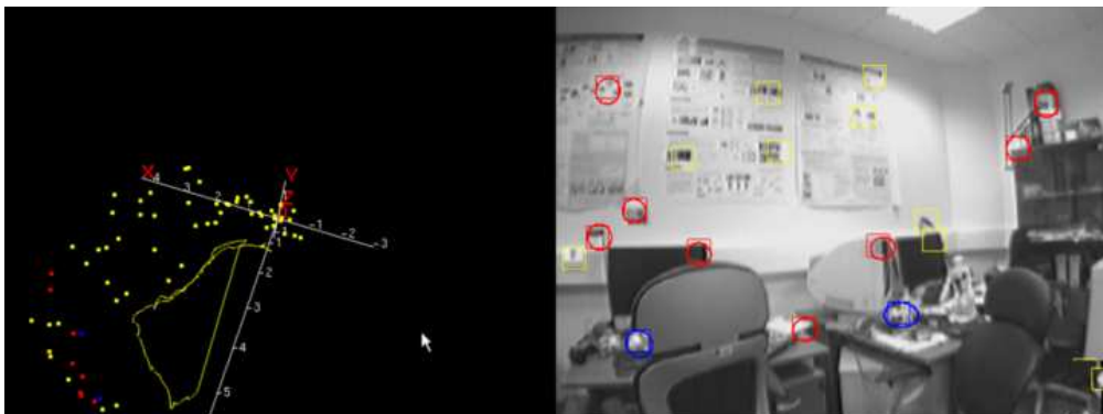
FIG. 11.7: Aperçu de la trajectoire de la caméra à la fin de l'expérience. Le cercle indique la pose finale de la caméra. On remarque que suite au kidnapping, une partie de la trajectoire parcourue à nouveau a été correctement reconnue.
