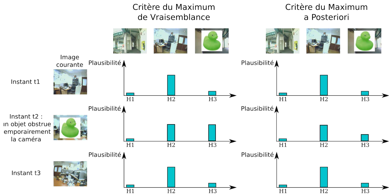
FIG. 1.2: Maximum de Vraisemblance vs. Maximum a Posteriori. Lorsque le canard vert passe devant la caméra à l'instant t_2 , les hypothèses H_2 et H_3 du modèle de l'environnement sont tout autant plausibles l'une que l'autre au sens du Maximum de Vraisemblance : ceci est dû au fait que le canard vert était déjà passé devant la caméra dans l'image correspondant à l'hypothèse H_3 . Dans le cas du critère de Maximum a Posteriori au contraire, même si l'hypothèse H_3 devient un peu plus plausible qu'auparavant, c'est toujours l'hypothèse H_2 qui est préférée. A l'instant t_3 , une fois que le canard vert a disparu, tout redevient normal.
