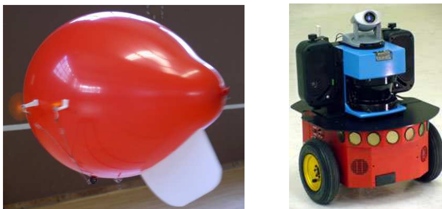
FIG. 2: L'utilisation de la vision permet de simplifier les dispositifs expérimentaux : une caméra monoculaire sans fil peut être facilement fixée à un ballon de baudruche gonflé à l'hélium (gauche), alors que l'utilisation d'un télémètre laser requiert une plate-forme plus imposante, dotée d'une charge utile et de réserves d'énergies conséquentes, comme en atteste le Pioneer 3DX d'ActivMedia Robotics (droite).
