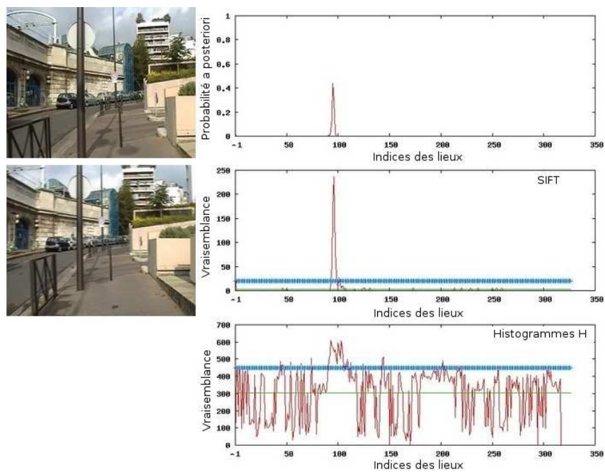
FIG. 3.10: Exemple d'une détection correcte de fermeture de boucle pour la séquence d'intérieur. Encore une fois, on peut observer que la vraisemblance obtenue dans l'espace de représentation SIFT est très importante et discriminante.
