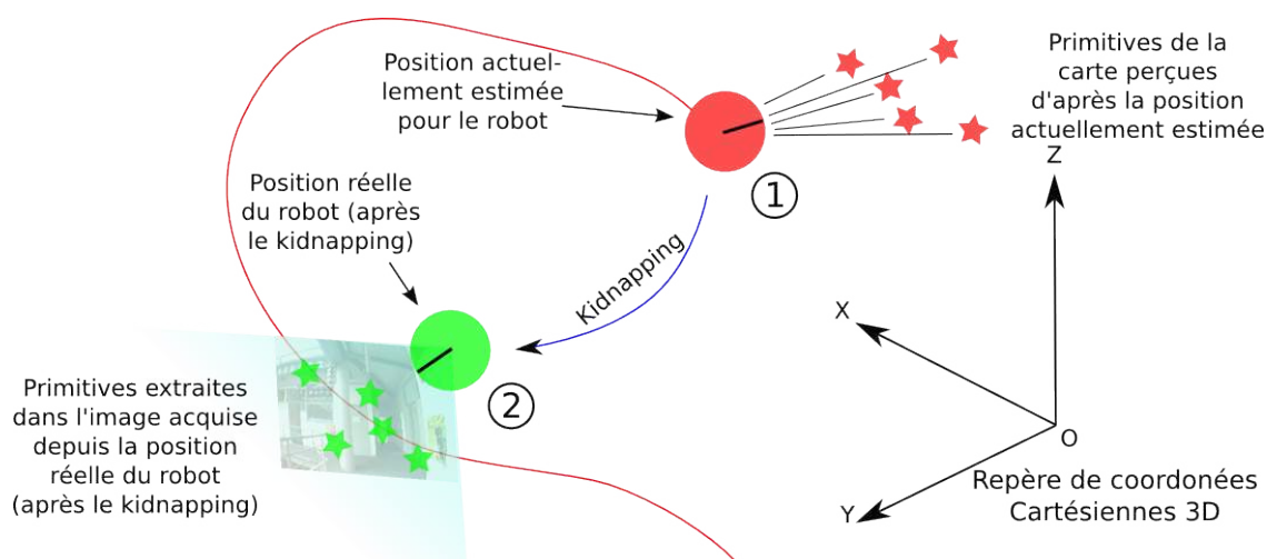
FIG. 1.12: Illustration du problème du robot kidnappé. Alors que le robot pense être à la position (1), il est kidnappé pour être déplacé à la position (2). Il faut alors mettre en correspondance les primitives extraites dans l'image acquise depuis la position (2) avec celles de la carte pour retrouver la bonne position. On peut notamment remarquer que les primitives localisées aux alentours de la position avant kidnapping ne sont plus cohérentes avec la nouvelle position.
