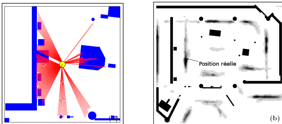
FIG. 1.11: Illustration du problème de la localisation globale : à partir des mesures provenant des capteurs (a), le robot doit inférer sa position dans la carte (b). Plus les positions sont plausibles, plus le niveau de gris est foncé. A partir d'une seule mesure il est difficile de reconnaître précisément le lieu où se trouve le robot, plusieurs positions distantes apparaissent donc comme plausibles. Source : [Fox, 1998].
