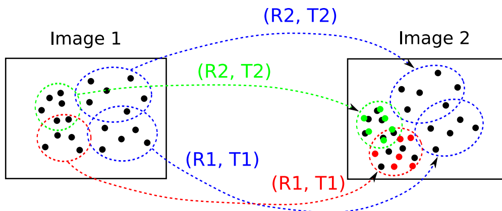
FIG. 2.14: Illustration de la procédure permettant de déterminer (si elle existe) la transformation joignant les points de vue de deux images. A partir de l'appariement d'un sous-ensemble de primitives locales entre les deux images (ellipse bleue), une première transformation (R1, T1) est calculée. Celle-ci est utilisée pour essayer de projeter d'autres primitives (ellipse rouge) d'une image à l'autre : les projections (points rouges) sont trop éloignées de leurs correspondants dans la seconde image, la transformation est rejetée. Une seconde transformation (R2, T2) est calculée à partir d'un nouveau sous-ensemble de primitives, permettant cette fois-ci des projections cohérentes (points verts) dans l'autre image : la transformation est retenue.
