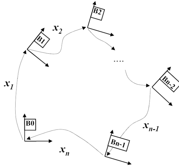
FIG. 1.14: Détection de fermeture de boucles dans le cadre d'une approche hiérarchique : par l'appariement de primitives entre les cartes B_{n-1} et B_0 , on peut exprimer la position relative x_n du référentiel de B_0 dans le référentiel de B_{n-1} , et ainsi détecter une fermeture de boucle entre ces cartes. Source : [Estrada et al., 2005].
