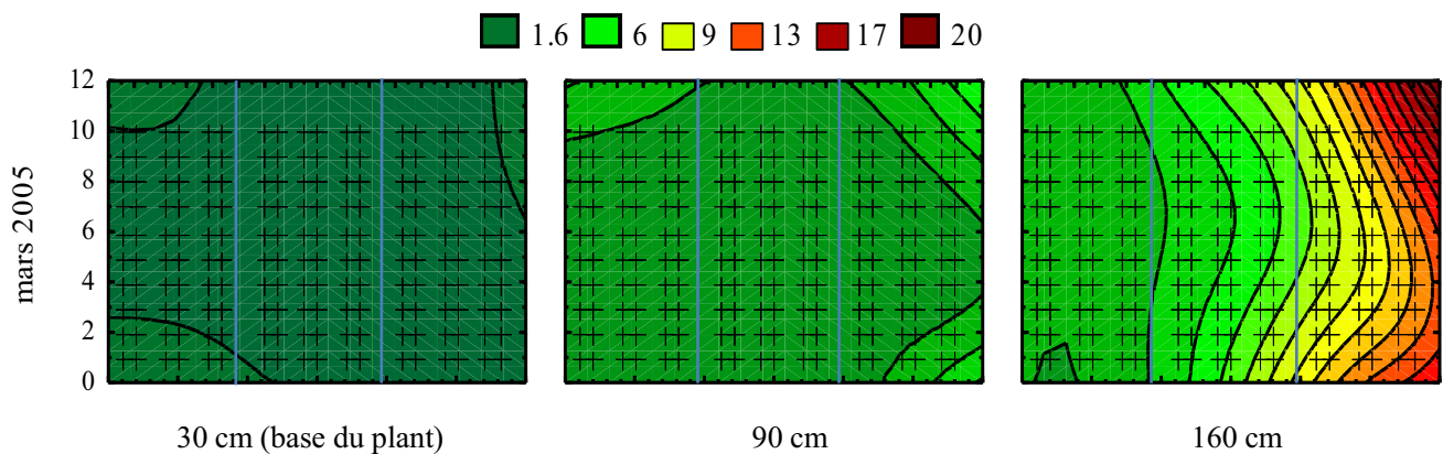
Figure 10. Courbes d'isoréponse de l'éclairage relatif dans la serre expérimentale. Les mesures ont été réalisées à l'aide d'un ceptomètre (AccuPAR, Model PAR-80, Decagon Devices, Inc., USA) à trois hauteurs : 30 cm, 90 cm et 160 cm du sol en mars 2005. Les croix représentent la position des points de mesures dans chacun des 3 traitements. L'éclairage relatif est exprimé en % du rayonnement solaire extérieur.
