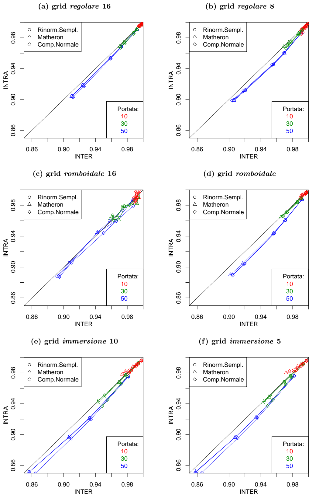
Figura 4.23: Scatter plot dei flussi cumulativi inter/intra-maglia, rapportati ai rispettivi casi omogenei, su ognuno dei sei grid considerati. Il calcolo delle trasmissività inter-blocco fornisce flussi cumulativi sistematicamente superiori, anche se di poco, all'intra, con la sola eccezione della portata 10.
