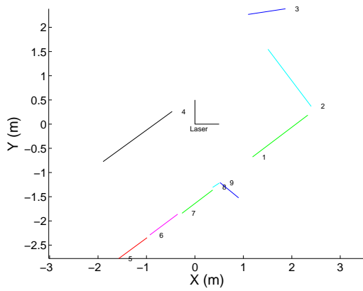
Figure 27: Segments extraits d'une coupe laser
