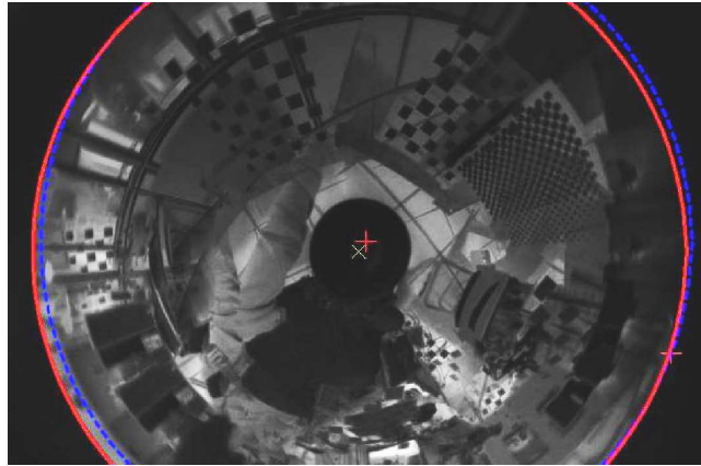
Figure 8: Extraction de la bordure du miroir pour estimer le point principal
