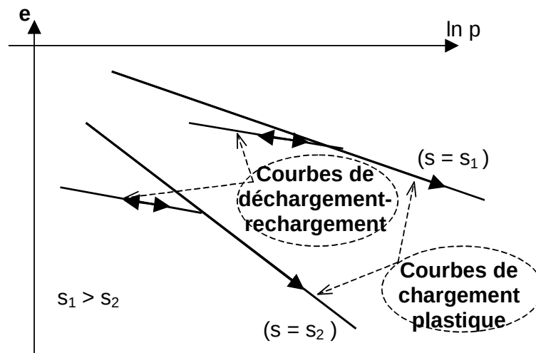
Figure 2.9. Variation de l'indice des vides avec la contrainte moyenne nette et la succion, en déchargement-chargement, Alonso et al. , (1990)
