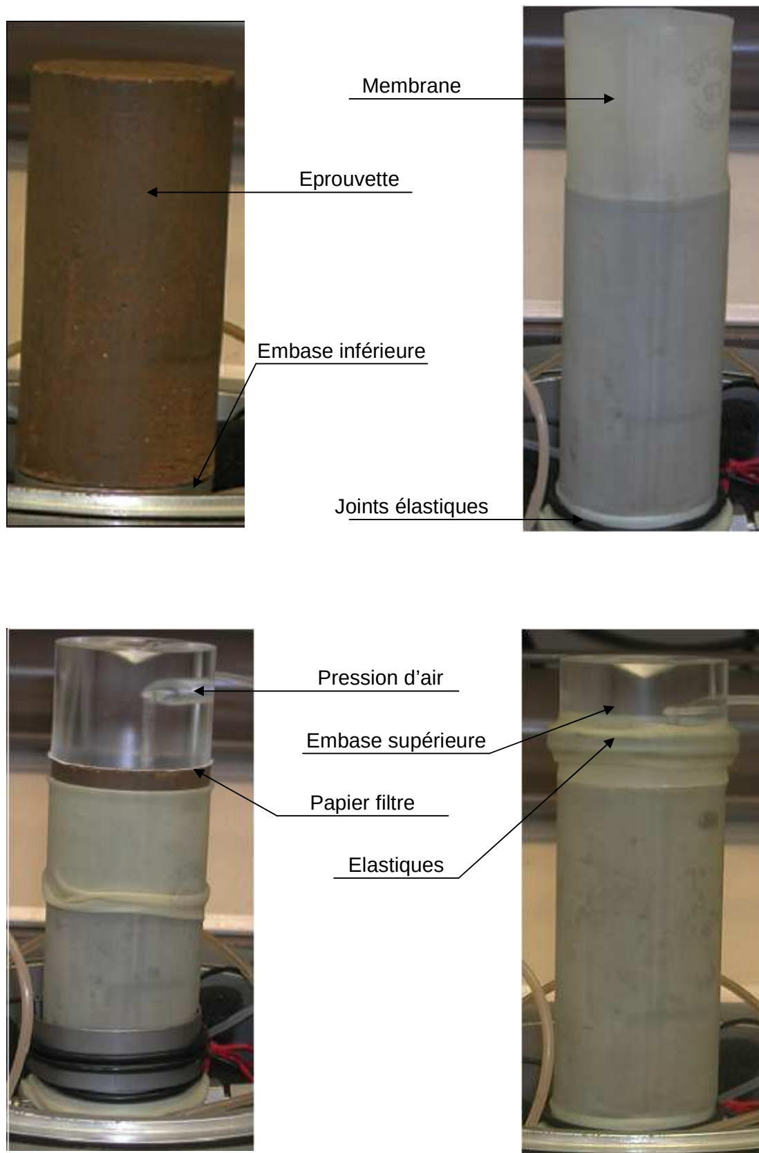
Figure 6.6. Différentes étapes de la mise en place de l'éprouvette
