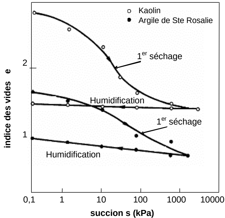
Figure 1.8. Variation de l'indice des vides en fonction de la succion pour deux argiles (Yong et al. , 1971 ; Alonso et al. , 1987)
