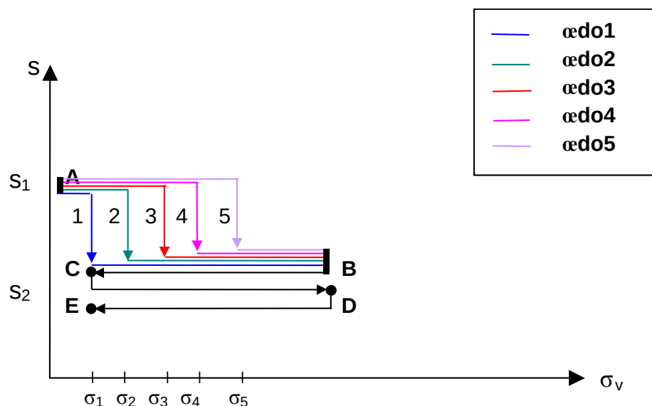
Figure 5.5. Chemin de sollicitation suivi pour les essais œdométriques avec imbibition, bloc A et bloc B
