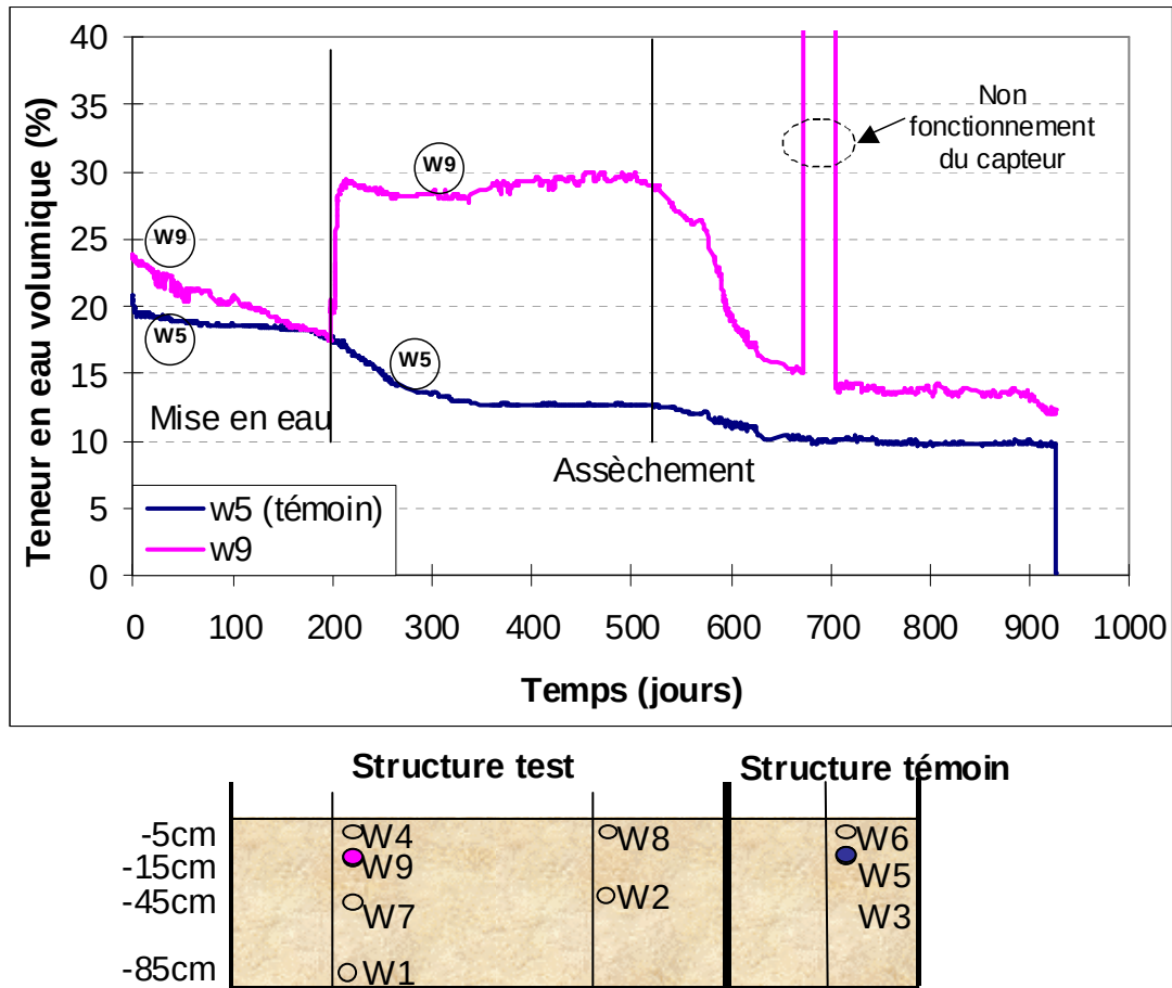
Figure 3.25. Évolution de la teneur en eau à 15 cm de profondeur
