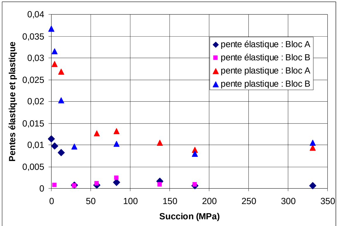
Figure 5.8. Pentes de la partie élastique ( \kappa ) et de la partie plastique ( \lambda ) des courbes de compressibilité en fonction de la succion imposée (bloc A et bloc B)
