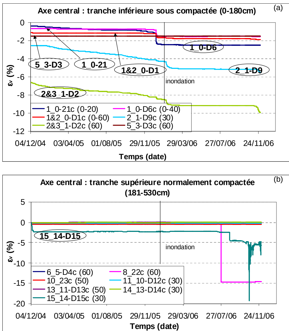
Figure 4.22. Déformation verticale au cours du temps sur l'axe central du remblai : a) tranche inférieure, b) tranche supérieure
