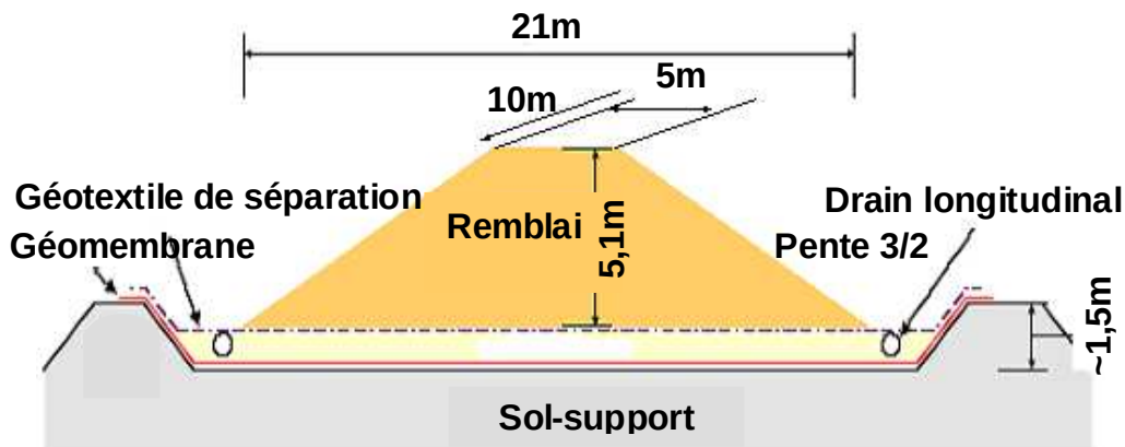
Figure 4.8. Profil en travers du remblai, structure du dispositif d'étanchéité et de drainage
