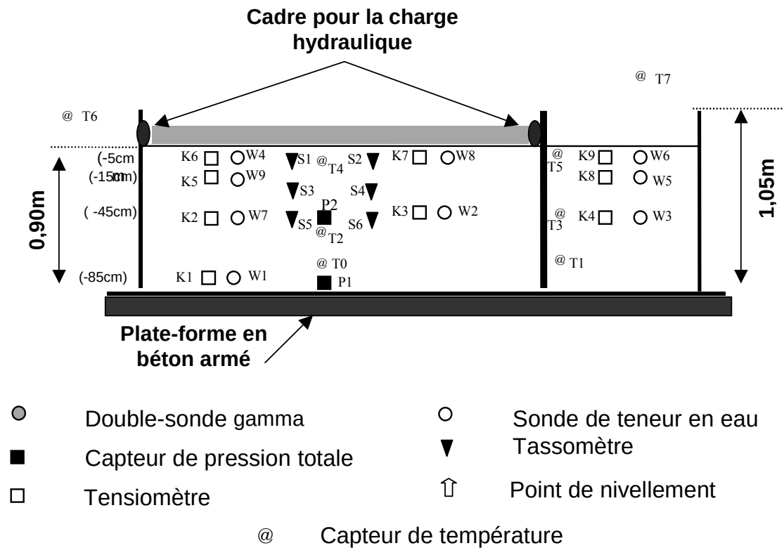
Figure 3.5. Coupe verticale des deux zones du remblai R1
