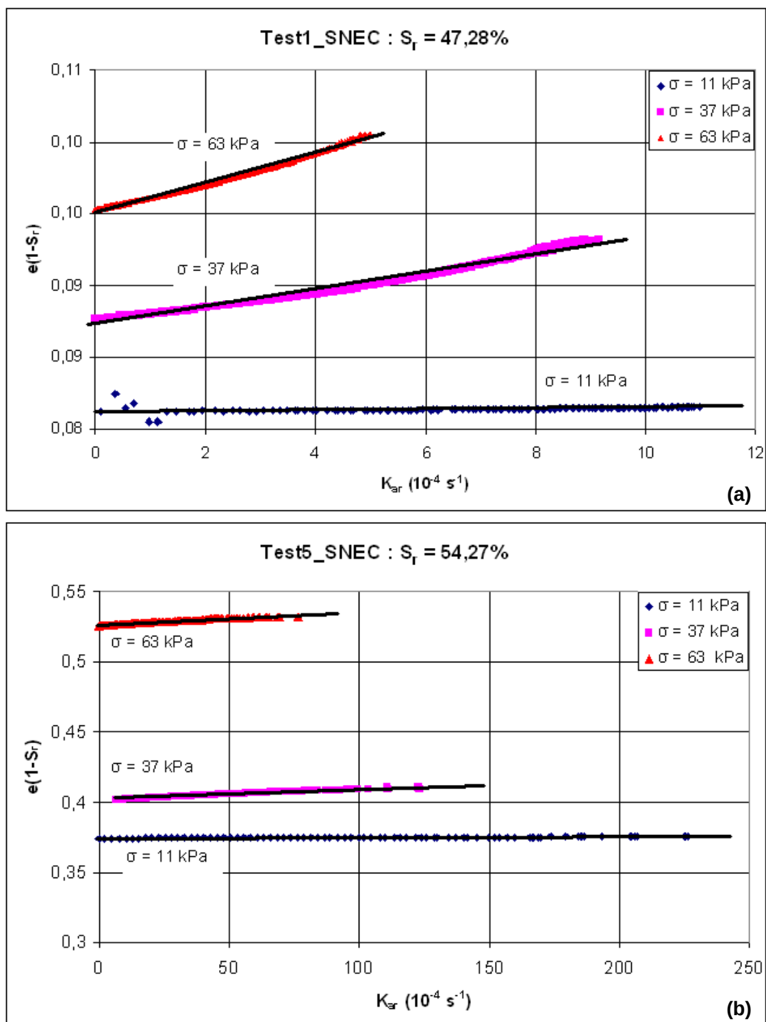
Figure 7.9. Variations de la perméabilité à l'air en fonction de l'indice des vides et du degré de saturation, pour le limon SNEC : (a) saturation de 47% (b) saturation de 54%
