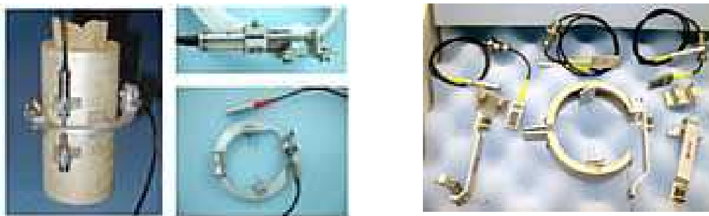
Figure 6.5. Capteurs locaux de déformation et leur montage autour de l'éprouvette
