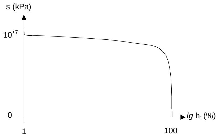
Figure 1.4. Relation entre la succion s et l'humidité relative de l'air à 20°C, d'après la loi de Kelvin
