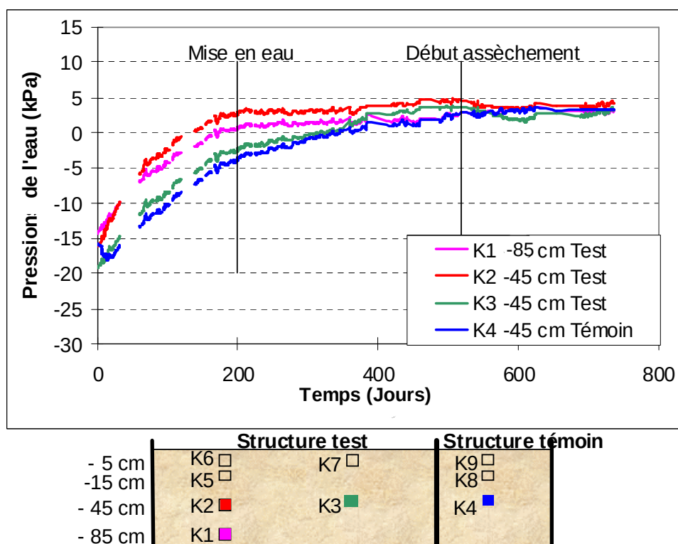
Figure 3.18. Évolution de la pression interstitielle à -45cm et -85cm en fonction du temps, zone expérimentale et zone témoin
