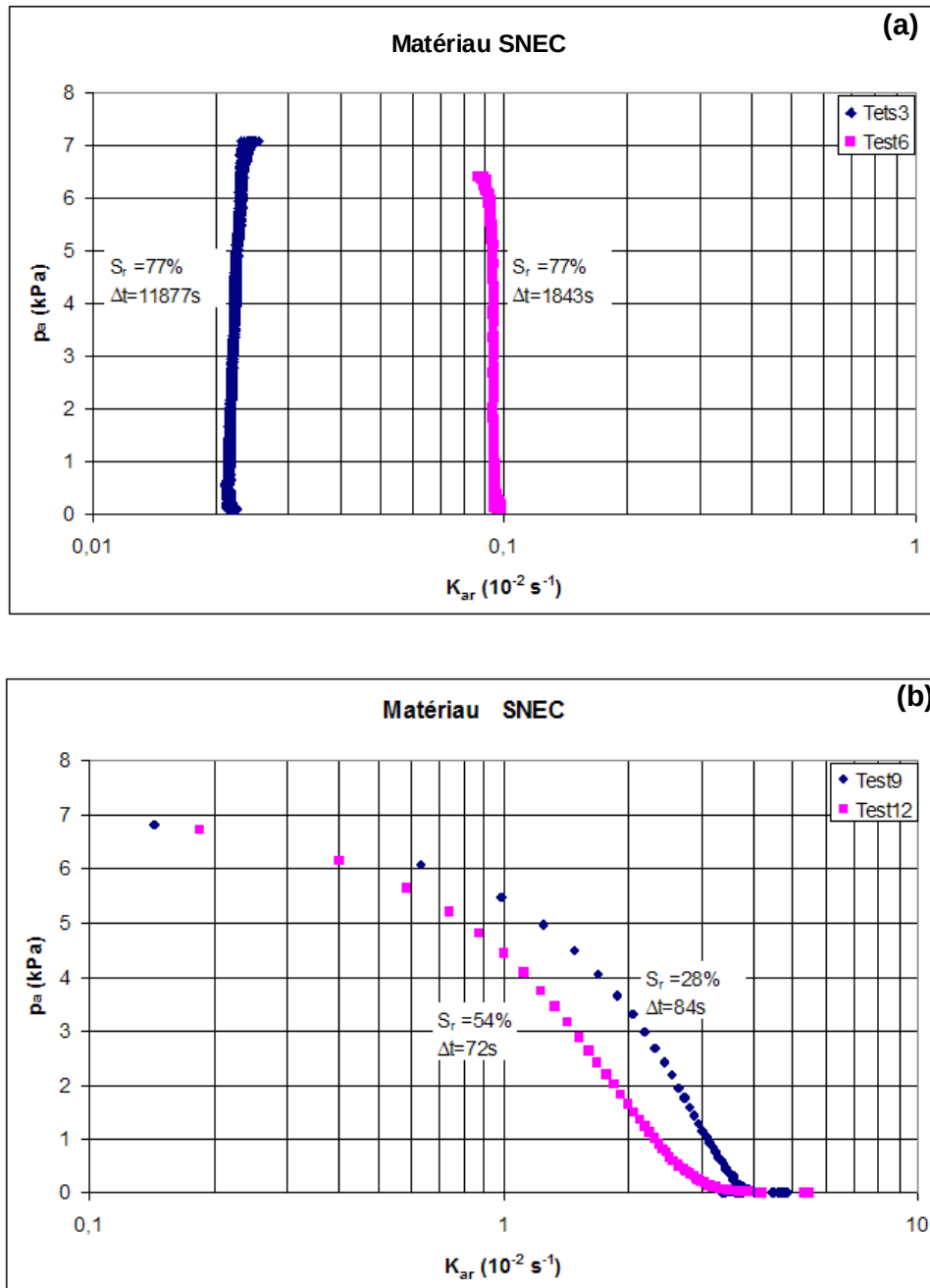
Figure 7.7. Variations de la pression d'air et de la perméabilité à l'air dans le limon SNEC : (a) poids volumique sec de 15 \text{ kN/m}^3 ; (b) poids volumique de 19 \text{ t/m}^3
