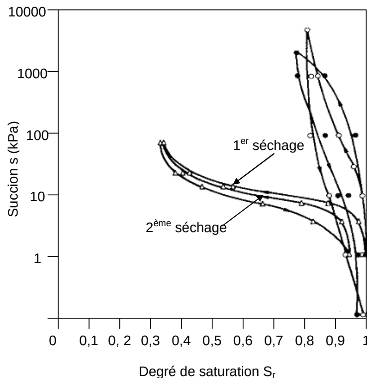
Figure 1.7. Variation du degré de saturation en fonction de la succion pour un sable fin (Croney et al. , 1958) et deux argiles (Yong et al. , 1971 ; Alonso et al. , 1987)
