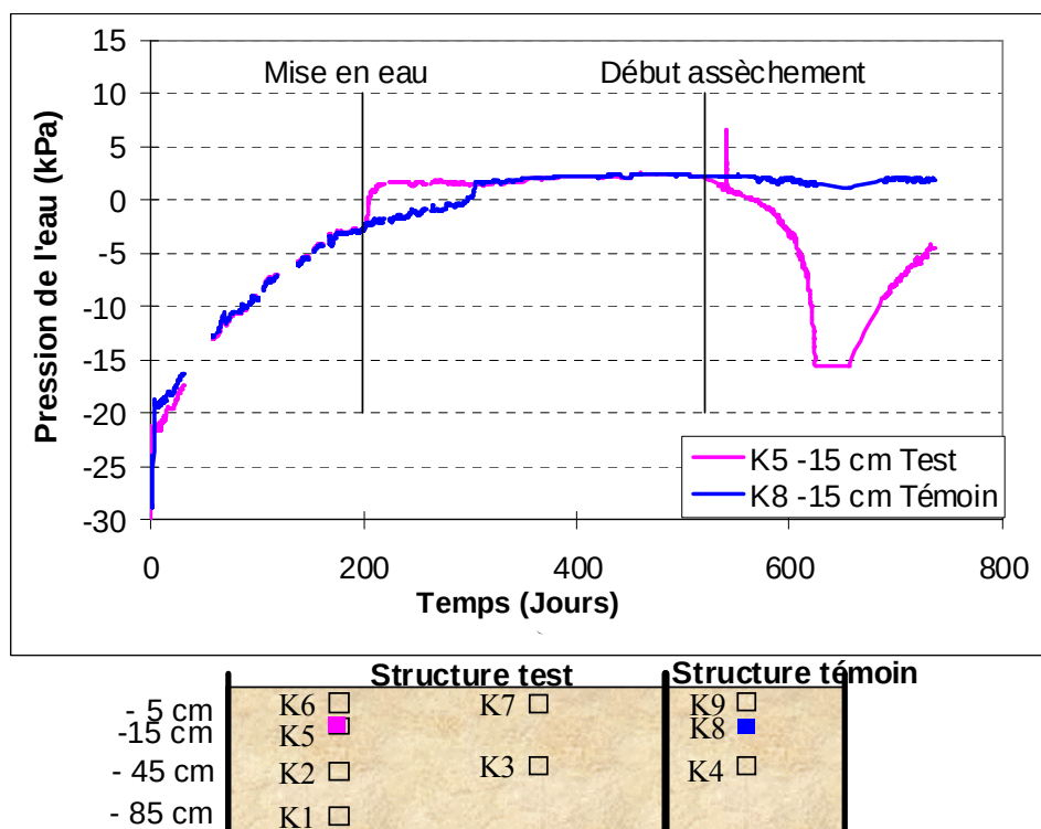
Figure 3.17. Évolution de la pression interstitielle à -15 cm en fonction du temps (zone expérimentale et zone témoin)
