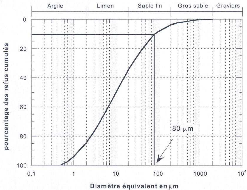
Figure 3.1. Courbe granulométrique de l'argile de Bavent (Alshihabi, 2002)
