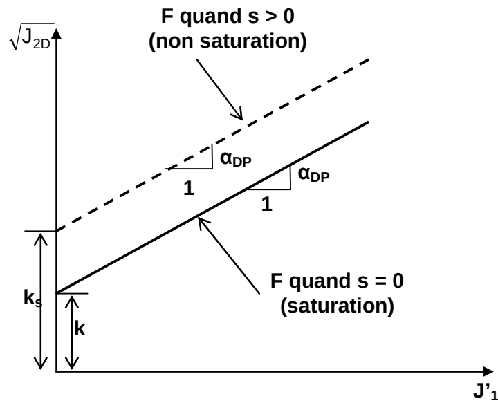
Figure 2.32. Surface d'état du modèle DP-s, (Rifa'l et al., 2002)
