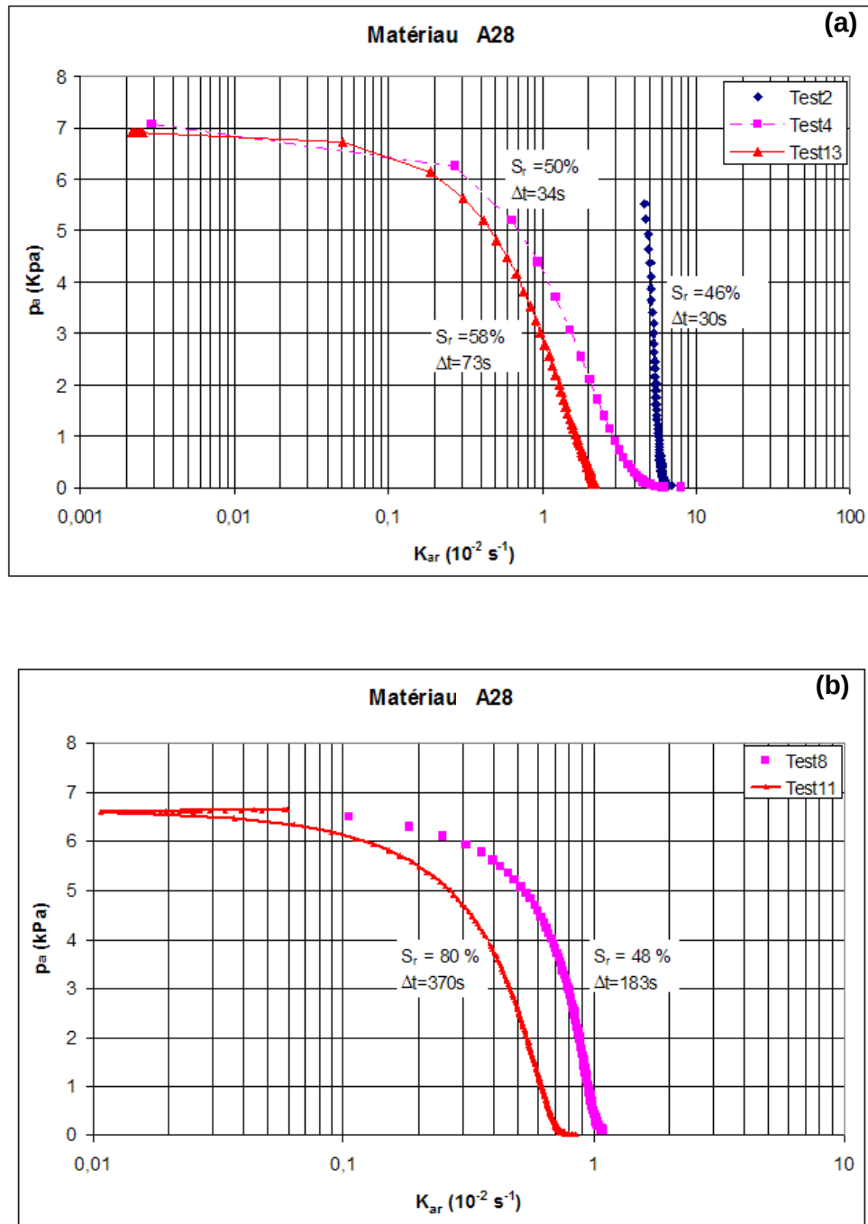
Figure 7.6. Variations de la pression d'air et de la perméabilité à l'air dans le limon A28 : (a) poids volumique sec de 14 \text{ kN/m}^3 ; (b) poids volumique de 16,4 et 17 \text{ kN/m}^3
