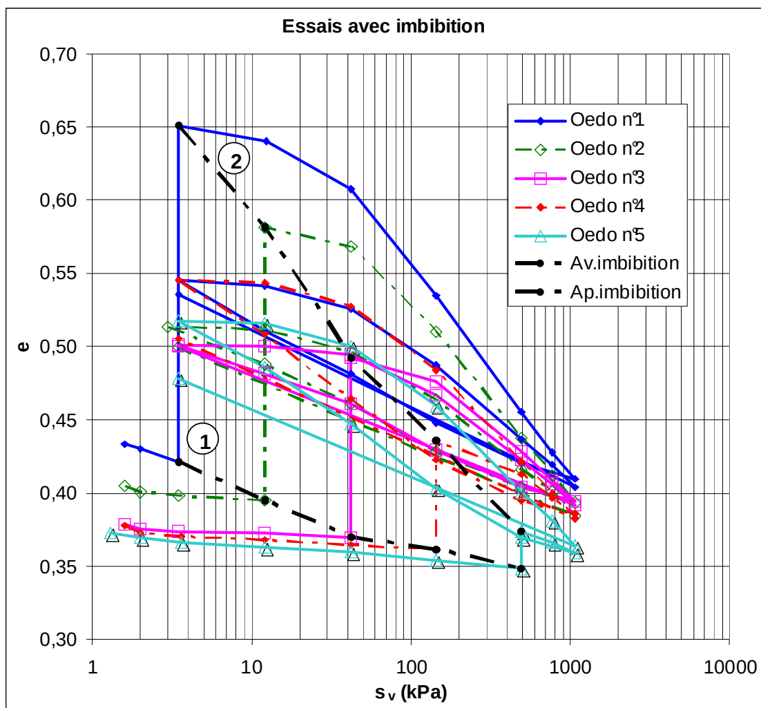
Figure 5.11. Indice de vides en fonction de la pression verticale avant et après imbibition, bloc témoin A
