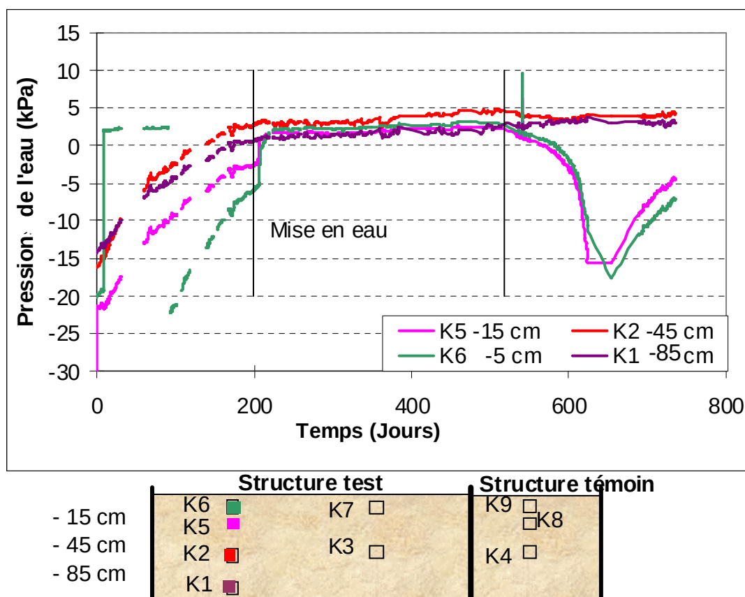
Figure 3.14. Évolution de la pression interstitielle dans le profil 1 en fonction du temps
