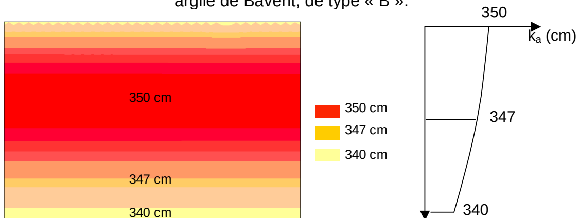
Figure 8.24. Isovaleurs de la charge d'air à la fin du calcul, s = 4,2 MPa argile de Bavent, de type « B ».
