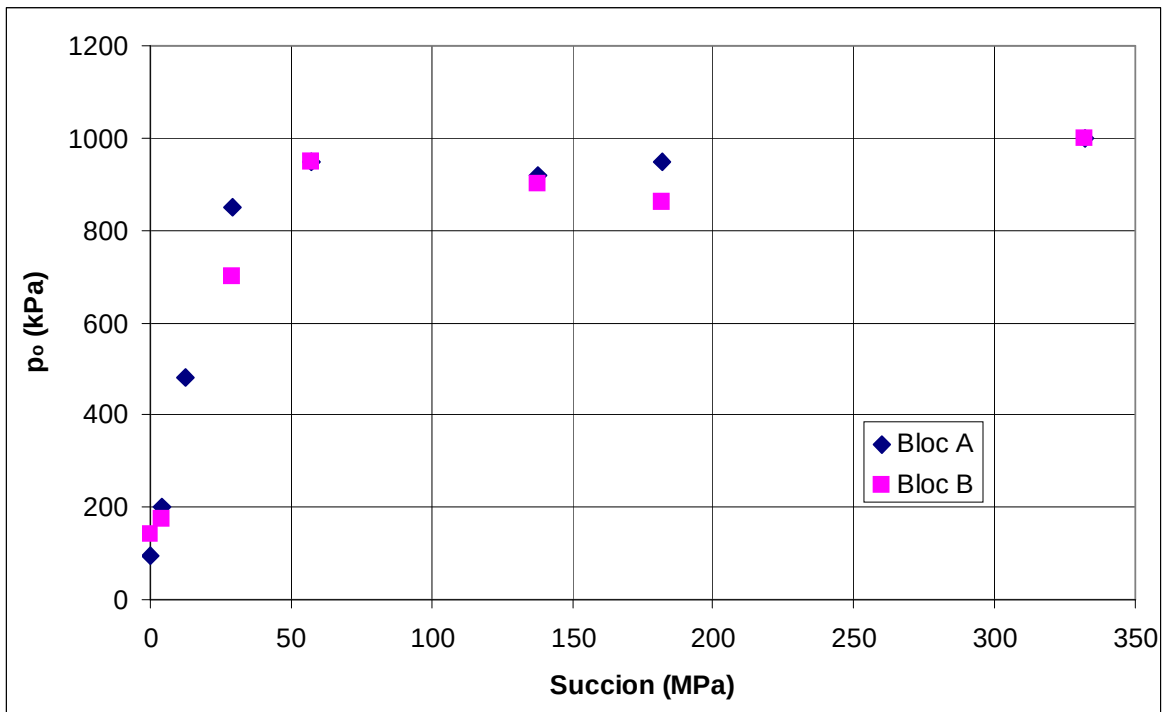
Figure 5.9. Variation de la pression de préconsolidation p_0 en fonction de la succion imposée (Bloc A et Bloc B)
