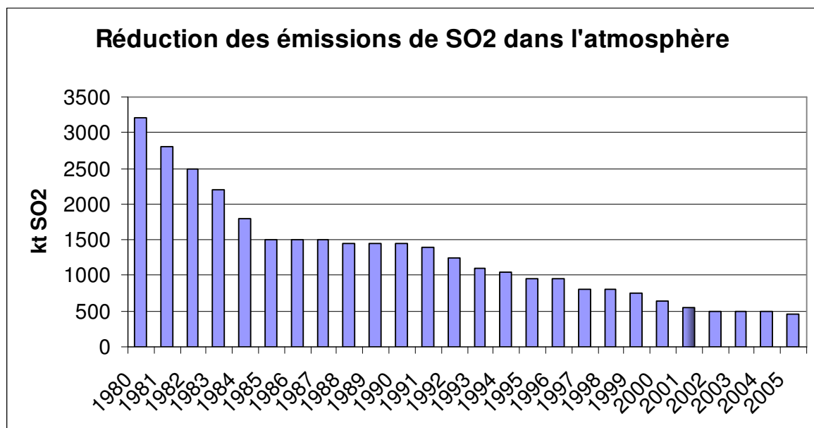
Figure 2 : Réduction des émissions de SO 2 dans l'atmosphère (Source CITEPA)
