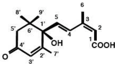
FIG. 1.1 – Formule semi-développée de l'acide abscissique
