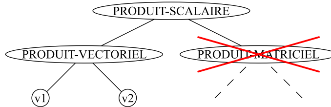
(b) Instanciation invalide : La fonction PRODUIT-SCALAIRE attend un vecteur en entrée et la fonction PRODUIT-MATRICIEL renvoie une matrice.
