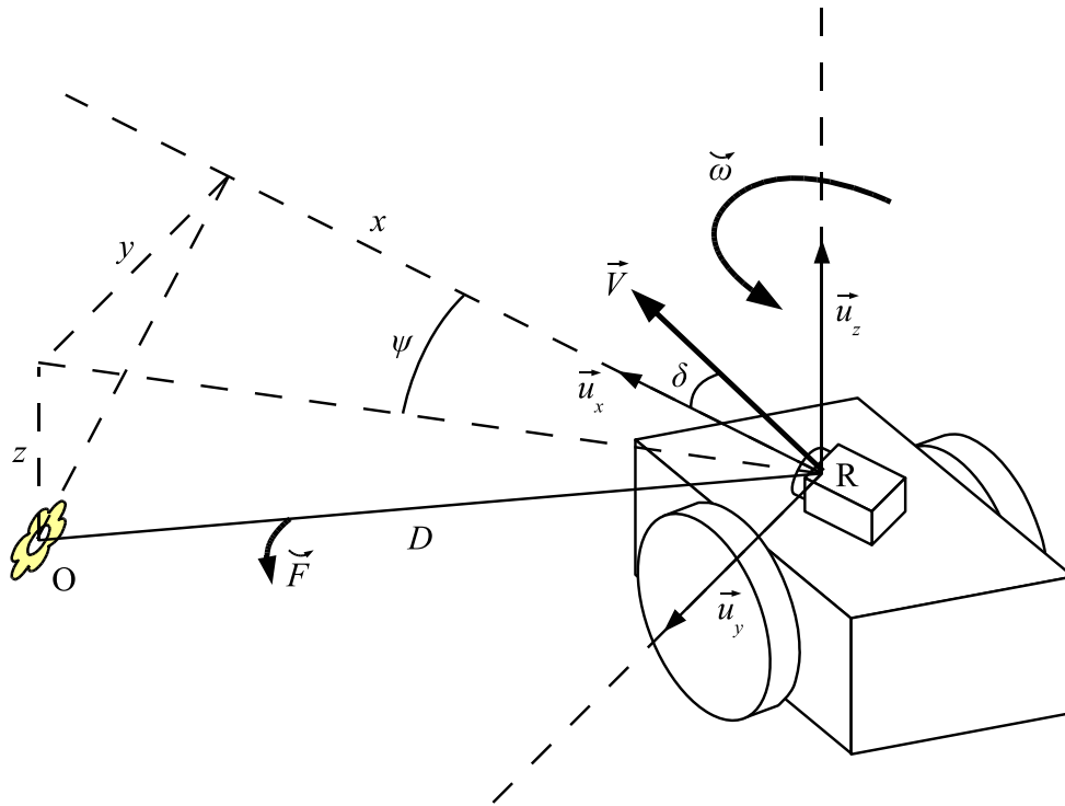
FIG. A.1 : Déplacement du robot générant le flux optique.
