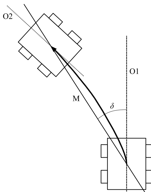
FIG. 2.2 : Angle généré par la séparation de deux images successives dans le temps. Le flux optique est calculé dans le repère correspondant à la première position du robot (axe optique O1), mais le déplacement correspondant a eu lieu selon l'axe M.
