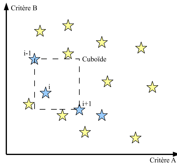
FIG. 3.10 : Calcul de la distance de voisinage avec l'algorithme NSGA-II. Les étoiles représentées en bleu correspondent aux solutions appartenant au même rang de non-domination. La distance de voisinage pour la solution i correspond au périmètre du cuboïde représenté sur la figure.
