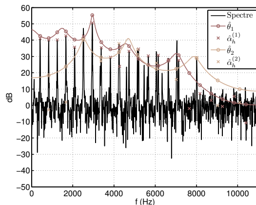
(e) Mélange Lab 3 (415 Hz) + Lab 4 (831 Hz) analysé par un modèle de Lab 3 + Lab 4.
