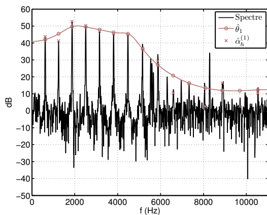
(b) Mib 4 (622 Hz) analysé par un modèle de Mib 4.
