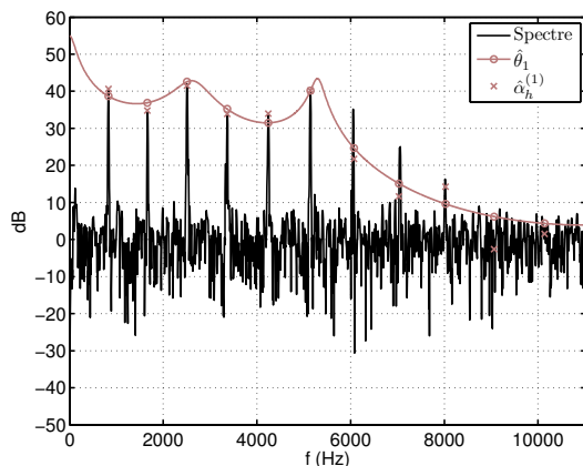
(d) Lab 4 (831 Hz) analysé par un modèle de Lab 3.
