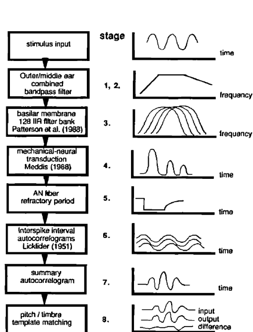
FIGURE 1.1 – Modèle de Meddis et Hewitt (Source : Meddis et Hewitt [1991a])
