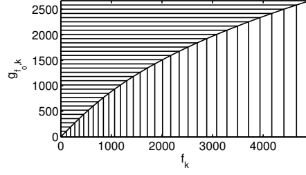
FIGURE 3.2 – Correction de l'inharmonicité : pour chaque fréquence fondamentale, les fréquences f_k sont transformées en g_{f_0,k} , afin de corriger les effets de l'inharmonicité. La figure représente un partiel sur cinq, avec f_0 = 27,5 Hz et \beta = 2,54 \cdot 10^{-4} .
