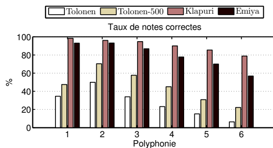
FIGURE 6.10 – Résultats de l'estimation de fréquences fondamentales multiples, la polyphonie étant connue. Le taux de notes correctes est représenté pour chaque algorithme, en fonction de la polyphonie originale.
