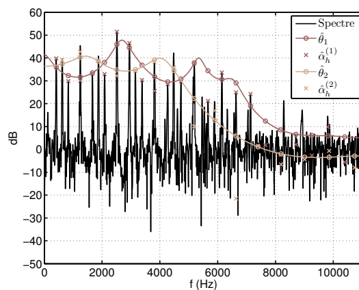
(c) Mélange Lab 3 (415 Hz) + Mib 4 (622 Hz) analysé par un modèle de Lab 3 + Mib 4.
