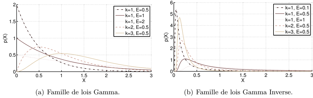
FIGURE A.1 – Densités des lois Gamma (gauche) et Gamma Inverse (droite) pour quelques valeurs de paramètres de forme k et d'échelle e .
