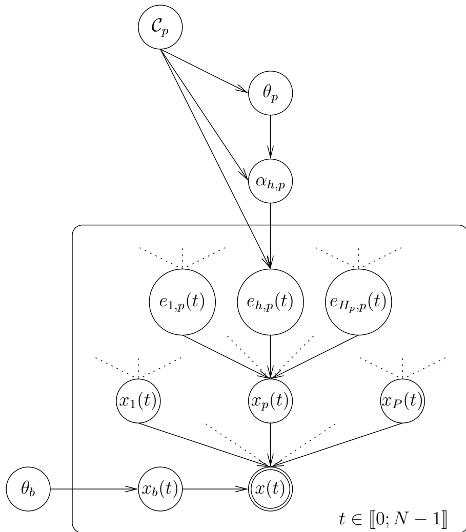
FIGURE 4.3 – Réseau bayésien représentant le modèle de son
