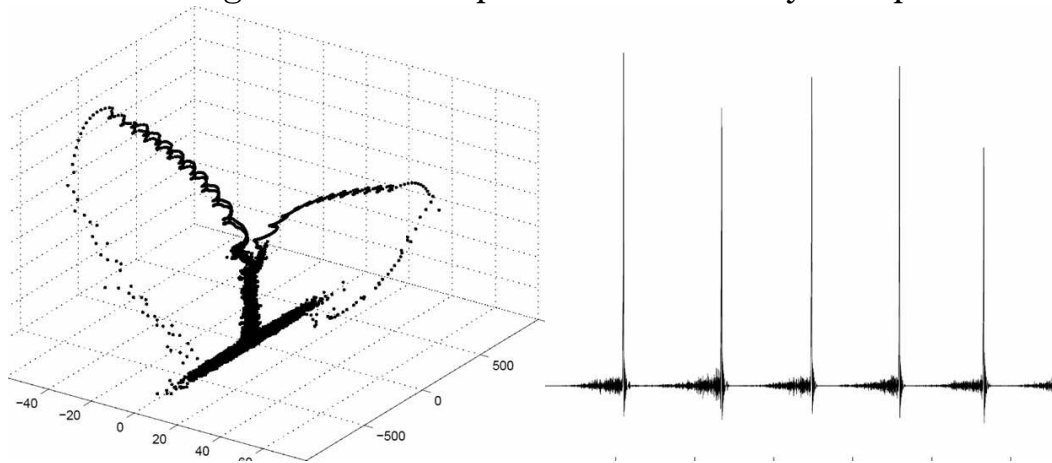
FIGURE 4.14 – La superposition des deux modes à l’opposé du spectre, dans le régime \nu \approx g est bien visible sur l’attracteur. L’envergure des deux ailes de papillons est très importante. Elles correspondent à des décharges de tout le plasma, i.e. à la dynamique d’ensemble.
