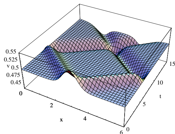
FIGURE 4.1 – Solution numérique (logiciel Mathematica) de l'équation (4.1) pour x \in [0; 6] avec les conditions aux limites v(0, t) = v(6, t) = 0.5 , v(x, 0) = 0.5 + 0.05 * \exp(-3(x - 3)^2) et \partial_t v(x, 0) = 0 .
