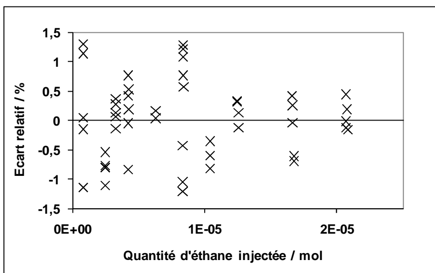
Figure 83 : Écarts relatifs entre les quantités d'éthane injectées et celles mesurées par le TCD en utilisant la corrélation de son facteur de réponse avec l'éthane
