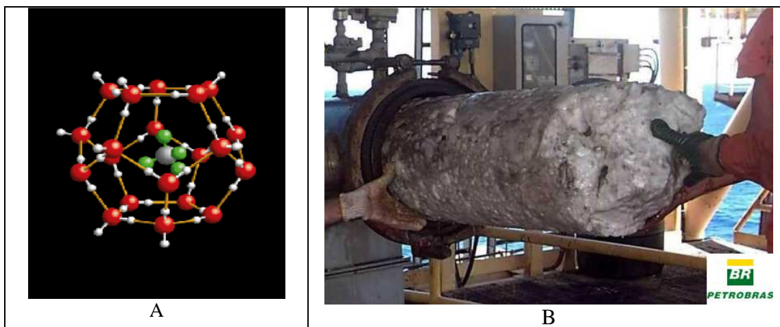
Figure 1 : A) Représentation d'un hydrate contenant une molécule de méthane [Kri08] B) Photographie d'un bouchon d'hydrate de gaz provenant d'un gazoduc [Min08]
