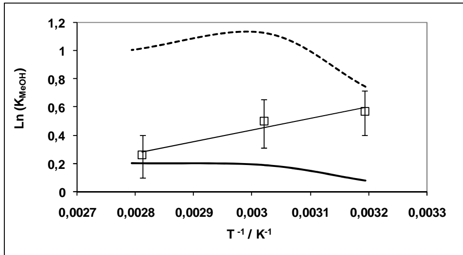
Figure 53 : Évolution de \ln ( K_{MeOH}^{\infty} ) (méthanol dans le propane) en fonction de l'inverse de la température
