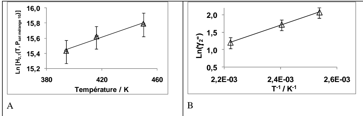
Figure 60 : A Évolution de \text{Ln} [H_{2,1}(T, P_{\text{sat}} \text{ mélange } 10)] du méthanol (2) dans le mélange 10 (1) en fonction de la température B Évolution de \text{Ln} (\gamma_2^{\text{inf}}) du méthanol dans le mélange 10 en fonction de l'inverse de la température ( \Delta ) : valeurs calculées à partir des constantes de Henry déterminées à chaque température, avec une courbe de tendance du premier ordre ; barres d'erreur estimées à partir de l'incertitude sur la mesure du coefficient de partage du méthanol
