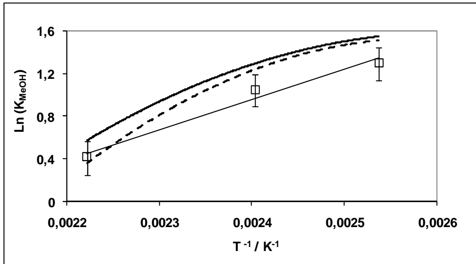
Figure 58 : Évolution \text{Ln} ( K_{MeOH}^{\infty} ) (méthanol dans le mélange 10) en fonction de l'inverse de la température
