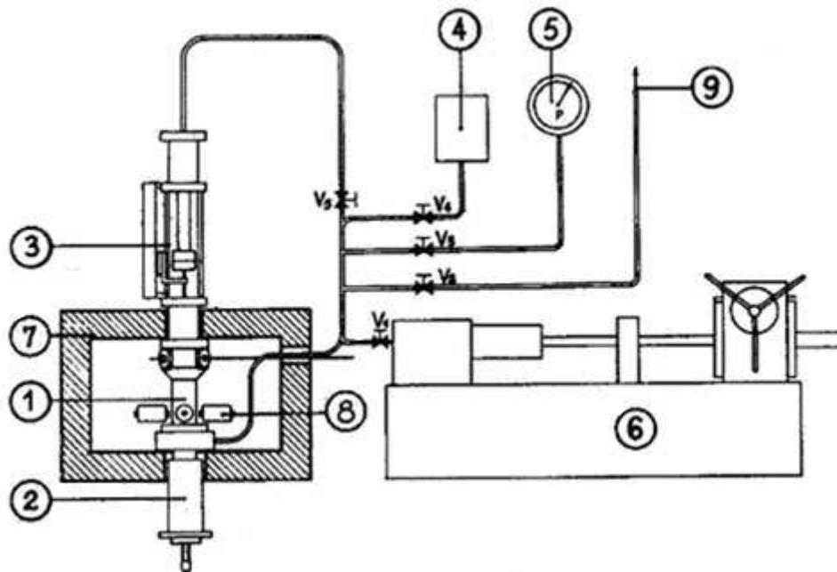
Figure 27 : Schéma de la cellule à volume variable
