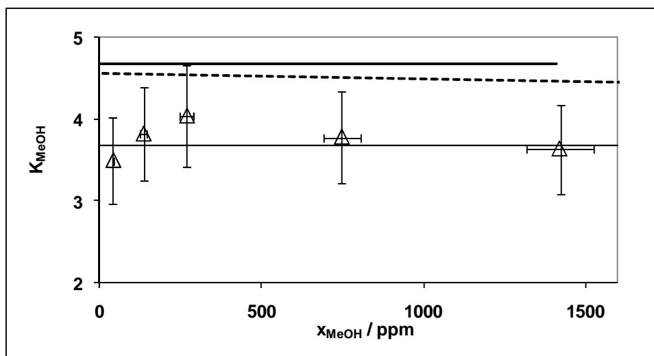
Figure 57 : Évolution du coefficient de partage du méthanol ( K_{\text{MeOH}} ) en fonction de sa fraction molaire en phase liquide ( x_{\text{MeOH}} ) pour l'ELV du système 'mélange 10 - méthanol' à 394 K
