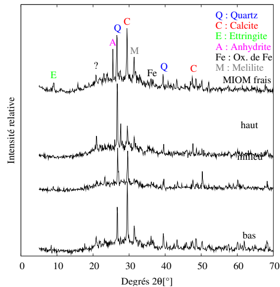
FIG. C.4 – Comparaison des diffractogrammes des MIOM frais avec ceux des MIOM correspondant à la carotte C (haut, milieu et bas de carotte) annotés des principaux pics (ettringite, calcite, quartz, ménilite, oxyde de fer).
