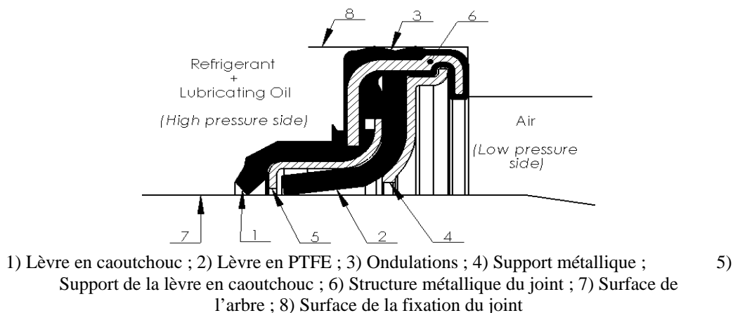
Figure 4 Vue en coup d'un joint tournant de compresseur
