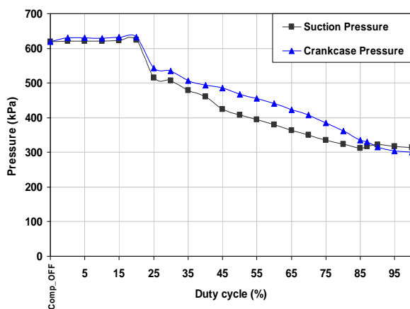
b) 1000 rev -1 , sh=5 K
