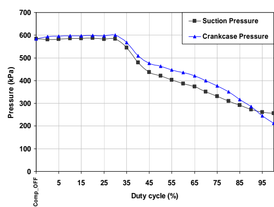
b) 3000 rev -1 , sh=5 K
