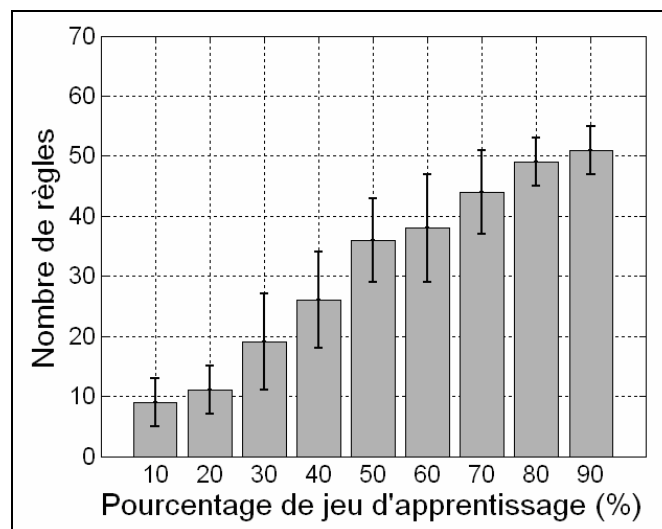
Figure 51. Nombres de règles générées automatiquement en utilisant les différents pourcentages de jeu d'apprentissage. Chaque barre représente le nombre moyen des règles obtenues pour 10 itérations et la barre d'erreur correspond à l'écart type.
