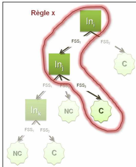
Figure 37. Schéma général d'un arbre de décision flou. Les nœuds In_i , ..., In_k sont des sous-ensembles de valeurs d'indicateurs, les FSS sont les sous-ensembles flous utilisés dans la partition de chaque indicateur, et C (coupe) et NC (Non Coupe) sont les possibilités de la sortie. Chaque chemin entre la racine et une feuille constitue une règle de décision ( e.g. Règle x : Si In_i est FSS_1 et In_j est FSS_2 Alors C ).
