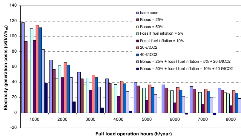
Figure 1.3 – Coût de production électrique actualisé (2007) pour différents systèmes de chauffage
