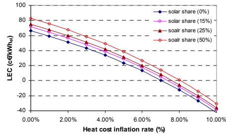
Figure 4.8 – Coût d'électricité actualisé fonction de l'inflation du prix du chauffage évité.
