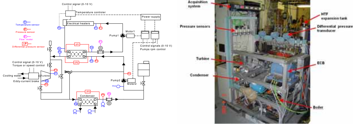
Figure 3.1 – Schéma et photo du banc d'essais des turbines
