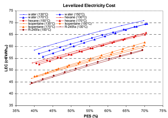
Figure 4.6 – Variation du coût d'électricité actualisé en fonction de l'économie d'énergie primaire, température d'ébullition et du fluide de travail.
