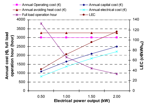
Figure 4.9 – L'effet de la capacité électrique sur le prix de la micro-cogénération et sa durée de fonctionnement annuelle.
