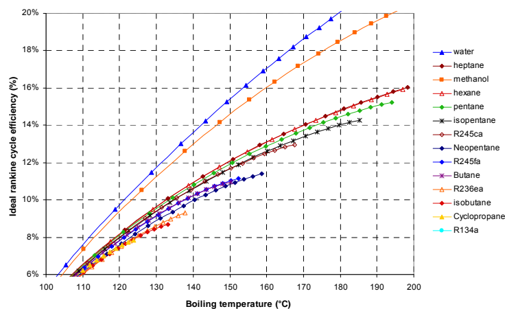
Figure 2.1 – Rendement idéal du cycle Rankine ( \eta_t = 1 , \eta_p = 1 , T_{sub} = 10 K, T_{sup} = 25 K si l'eau est le fluide de travail et 1 K pour les différents autres fluides de travail)
