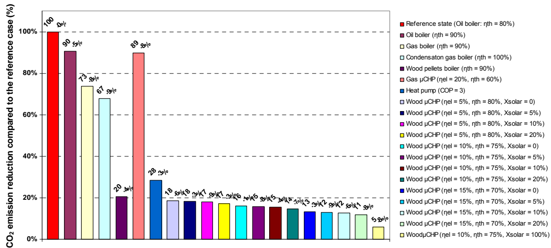
Figure 1.2 – Réductions d'émissions du \text{CO}_2 pour différents systèmes de chauffage
