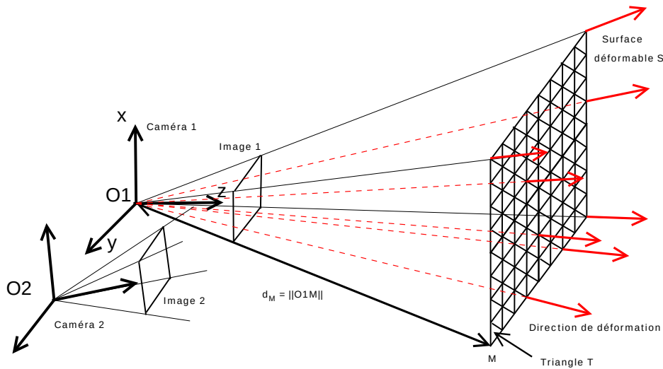
FIGURE 5.2 – Modèle à deux caméras. La caméra 1, de centre optique O1 est la caméra de référence. Pour chaque point M de S est lancé un rayon à partir de O1 , ce rayon détermine la direction de déplacement pour M .
