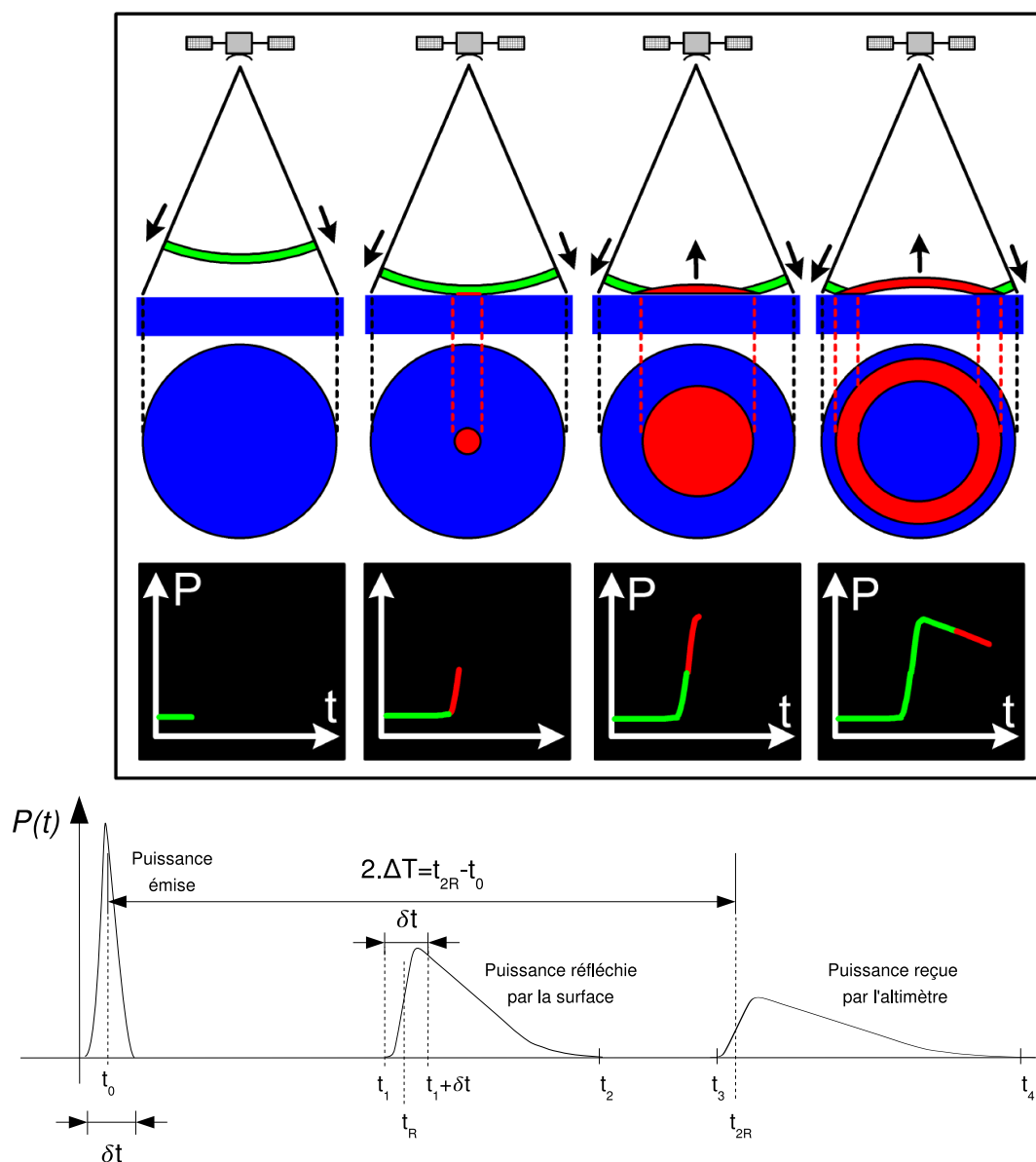
FIG. 1.4: Illustration de la formation au cours du temps de l'onde radar réfléchie par la surface au nadir (en haut, d'après un document CNES) et de l'onde radar reçue par l'altimètre (en bas).
