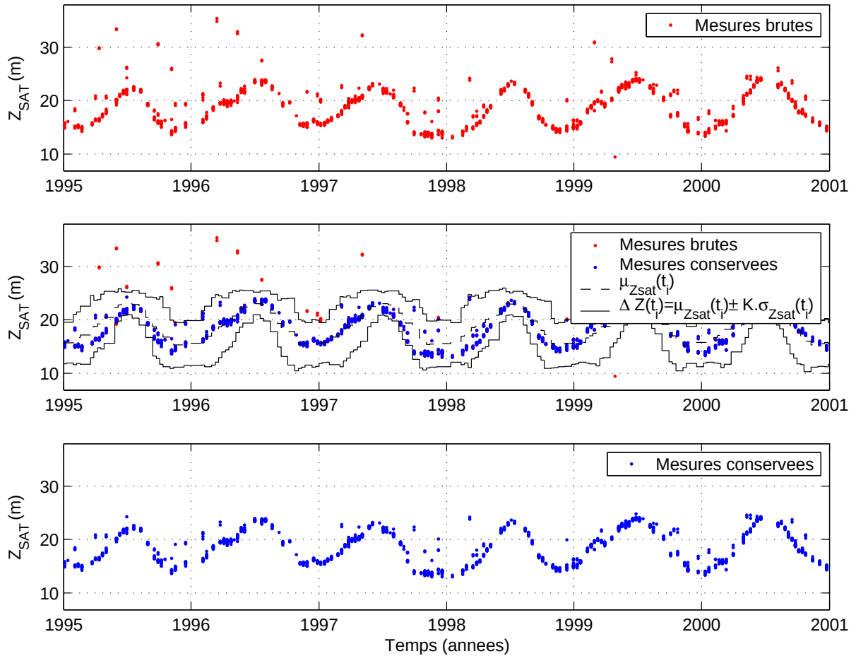
Illustration du filtrage calendaire ( \Delta T/2=15 (jours), K=2.5 , qT=1 (jours)), "TP-241A-Negro"
