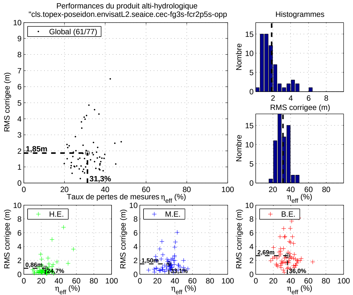
FIG. 7.17: Figure de synthèse pour le meilleur produit alti-hydrologique issu du groupe CLS ENVISAT-L2, retracker SeaIce (Topex/Poseidon).
