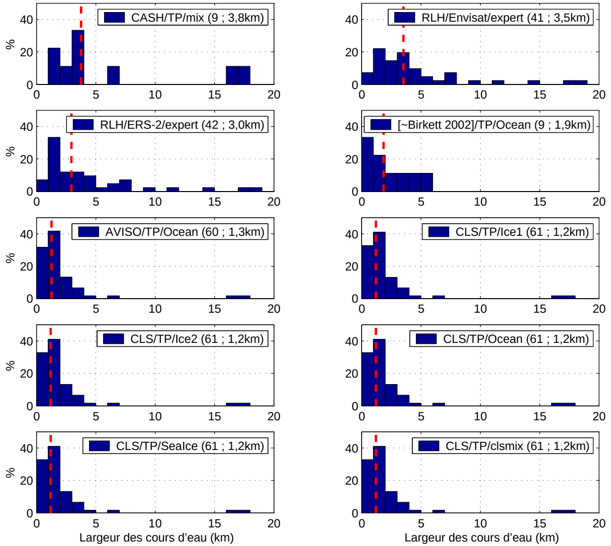
FIG. 7.24: Histogrammes des largeurs de rivières aux stations virtuelles des 10 produits alti-hydrologiques (cf. table 7.23 et figure 7.23).
