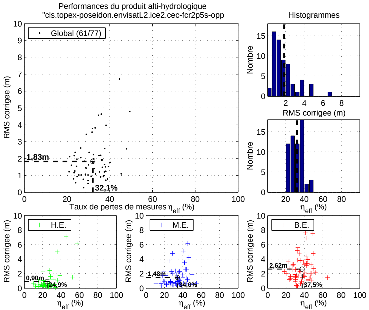
FIG. B.39: Figure de synthèse pour le produit alti-hydrologique « cls.topex-poseidon.envisatL2.ice2.cec-fcr2p5s-opp ».
