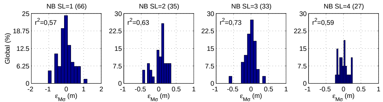
FIG. 6.6: Histogrammes de l'erreur résiduelle ( \epsilon_{\mathcal{M}} ) des quatre modèles d'estimation de \sigma_{\varepsilon_{Rec}} .
