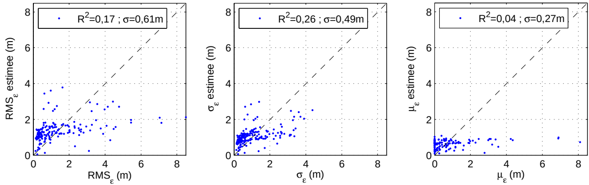
FIG. 8.3: Modèles saisonniers : Illustration de la sortie des modèles multivariables d'estimation des indicateurs de précision pour le produit alti-hydrologique AVISO/TP/M-GDR en fonction de leurs valeurs réelles. La ligne en pointillé illustre la droite de corrélation idéale. Les valeurs de \sigma présentées dans les graphiques sont les écart-types de l'erreur résiduelle des modèles.
