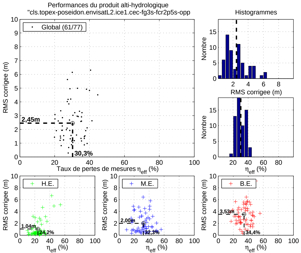
FIG. B.31: Figure de synthèse pour le produit alti-hydrologique « cls.topex-poseidon.envisatL2.ice1.cec-fg3s-fcr2p5s-opp ».
