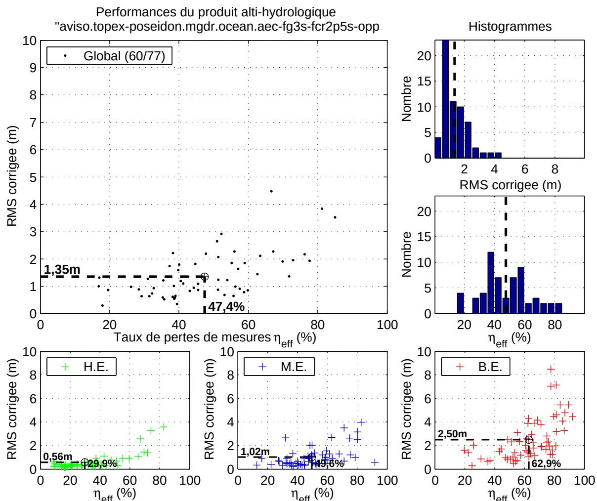
FIG. B.10: Figure de synthèse pour le produit alti-hydrologique « aviso.topex-poseidon.mgdr.ocean.aec-fg3s-fcr2p5s-opp ».
