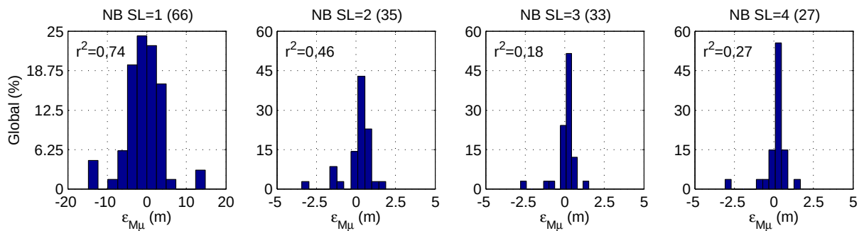
FIG. 6.5: Histogrammes de l'erreur résiduelle ( \epsilon_{\mathcal{M}} ) des quatre modèles d'estimation de \mu_{\varepsilon_{Rec}} .
