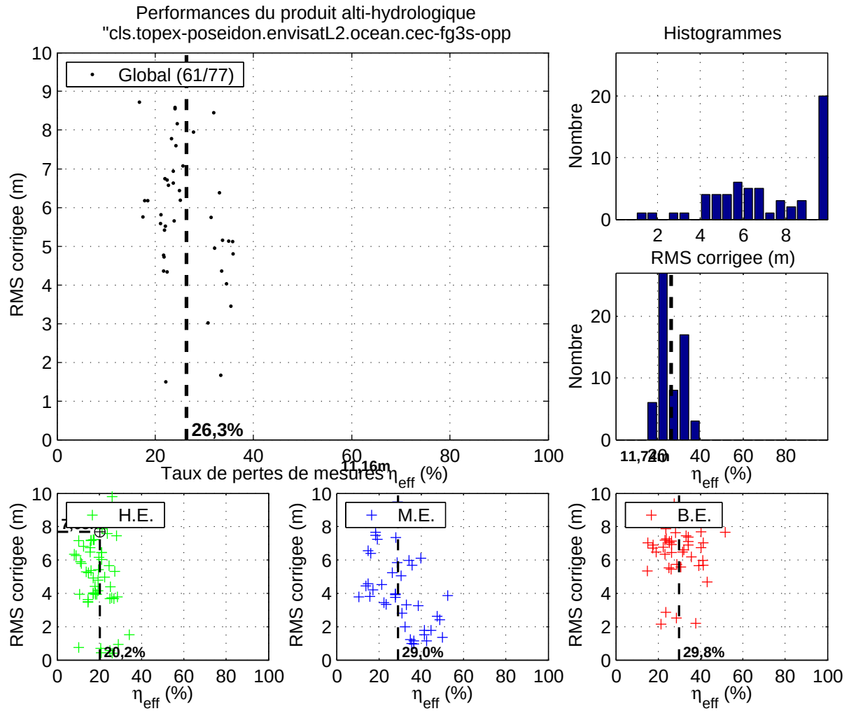
FIG. B.23: Figure de synthèse pour le produit alti-hydrologique « cls.topex-poseidon.envisatL2.ocean.cec-fg3s-opp ».
