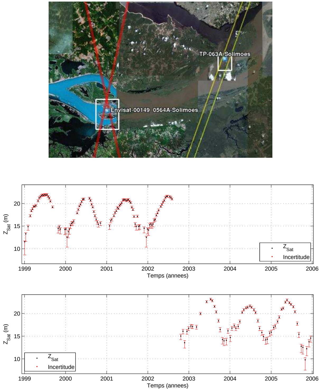
FIG. 8.12: Illustration de séries temporelles alti-hydrologiques avec valeurs d'incertitude associées. Les deux séries temporelles alti-hydrologiques sont issues de deux stations virtuelles voisines (distantes de 30km) sur le fleuve Solimões. En haut : station virtuelle sur la trace 63 de Topex/Poseidon (produit alti-hydrologique AVISO/TP/M-GDR) ; En bas : station virtuelle sur les traces 149 et 564 d'ENVISAT (produit alti-hydrologique RLH/ENVISAT). Cette dernière série temporelle est construite par agglomération des mesures altimétriques collectées sur les deux traces 149 et 564, et présente une période d'échantillonnage inférieure à 35 jours (nominalement \frac{35}{2} jours). On peut constater pour ces deux séries temporelles alti-hydrologiques que l'incertitude sur les mesures est plus grande pendant les périodes de basses eaux.
