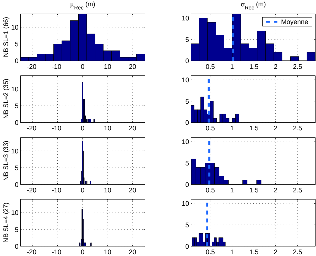
FIG. 6.3: Histogrammes des indicateurs de précision de reconstitution ( \mu_{\varepsilon_{Rec}} et \sigma_{\varepsilon_{Rec}} ) quantifiés sur les stations limnimétriques de test. Les histogrammes de chaque ligne illustrent les résultats obtenus pour chacune des méthodes de reconstitution, s'appuyant respectivement sur les mesures in-situ issues de 1, 2, 3 ou 4 (Nb SL) stations limnimétriques amont et aval. Colonne de gauche : histogrammes des valeurs moyennes de l'erreur de reconstitution \mu_{\varepsilon_{Rec}} ; Colonne de droite : écart-types de l'erreur de reconstitution \sigma_{\varepsilon_{Rec}} . Le nombre de combinaisons de stations limnimétriques pour chacune des méthodes illustrées est indiqué entre parenthèses (sur la gauche de la colonne de gauche).
