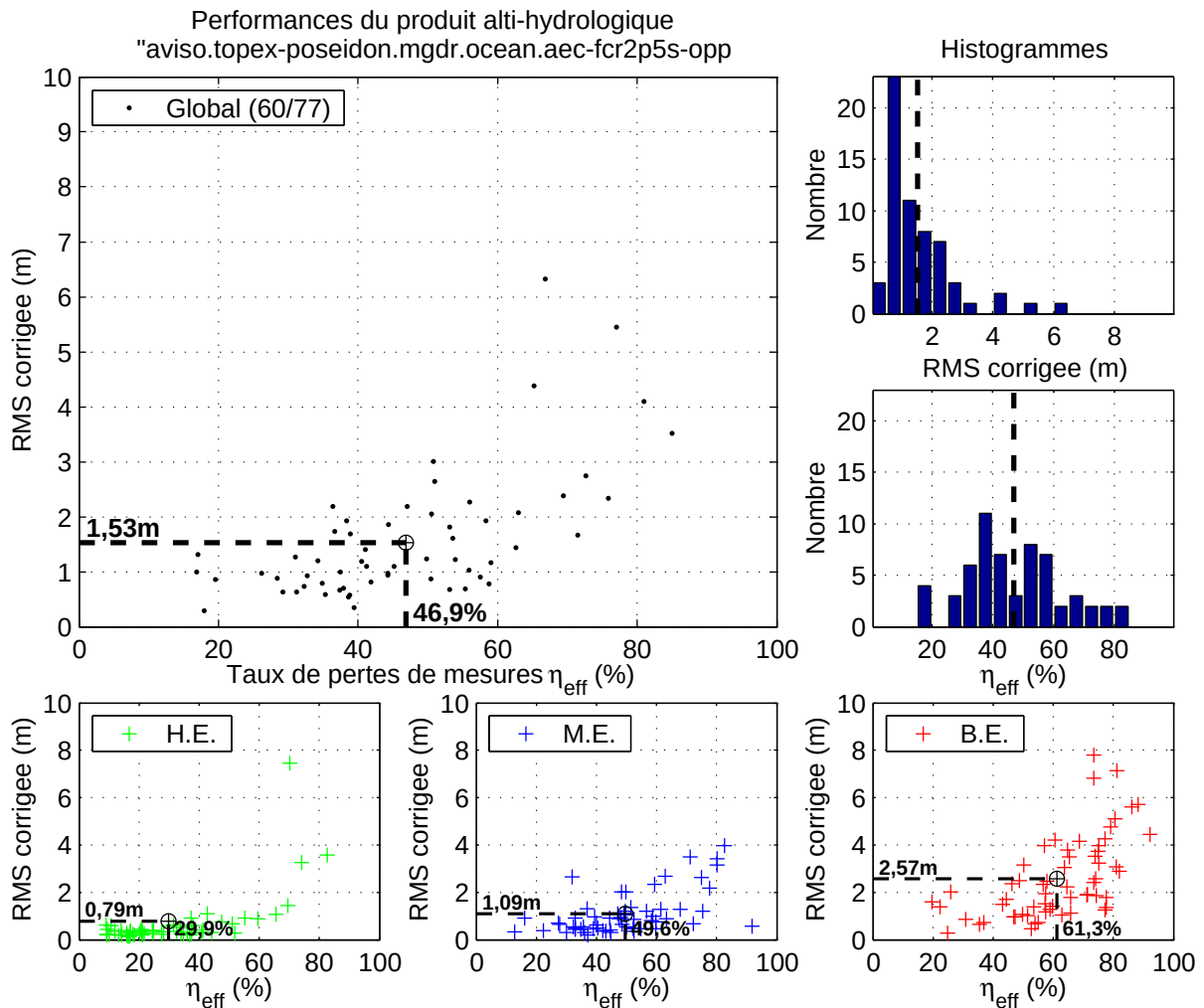
FIG. B.11: Figure de synthèse pour le produit alti-hydrologique « aviso.topex-poseidon.mgdr.ocean.aec-fcr2p5s-opp ».
