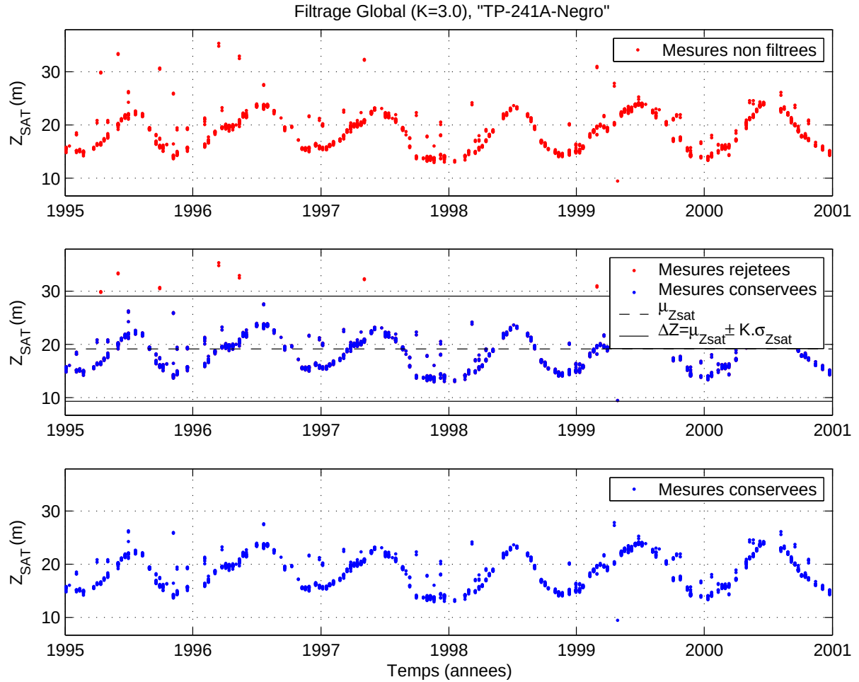
FIG. 3.7: Illustration du filtrage global sur la série temporelle de la station virtuelle « TP-241A-Negro », pour K = 3 . En haut : La série temporelle avec plusieurs mesures par passage contenant un certain nombre de mesures aberrantes. Au milieu : Les mesures en rouge sont en dehors des limites définies par l'intervalle \Delta_Z (lignes en trait plein noirs en haut et en bas) et sont retirées de la série temporelle. En bas : la série temporelle résultante. Ce filtre permet de retirer les mesures aberrantes dont l'altitude n'est pas comprise dans la dynamique générale de la série temporelle.
