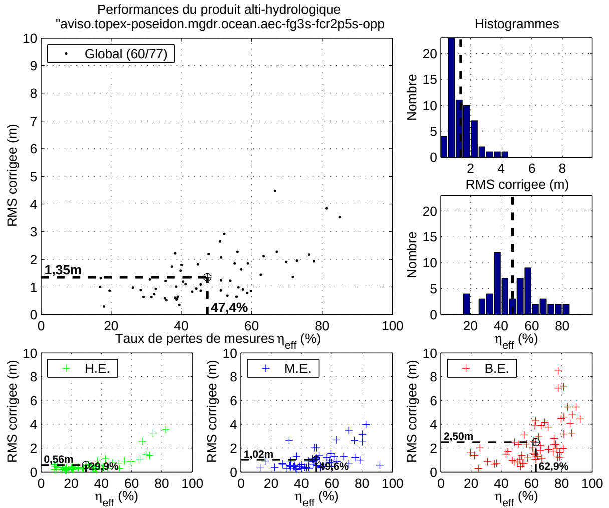
FIG. 7.13: Figure de synthèse pour le meilleur produit alti-hydrologique issu du groupe AVISO M-GDR, tracker Ocean (Topex/Poseidon).
