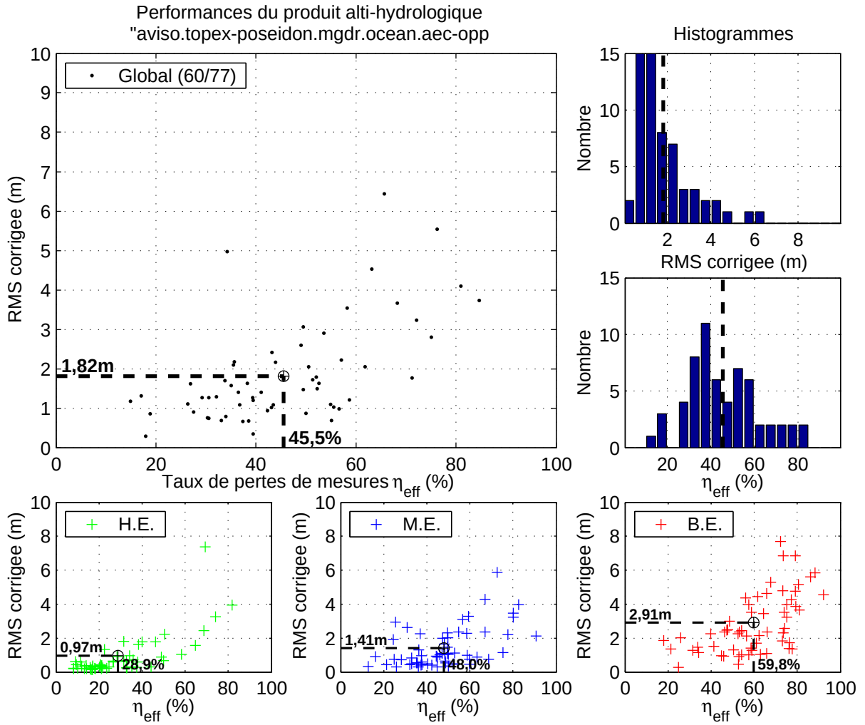
FIG. B.5: Figure de synthèse pour le produit alti-hydrologique « aviso.topex-poseidon.mgdr.ocean.aec-opp ».
