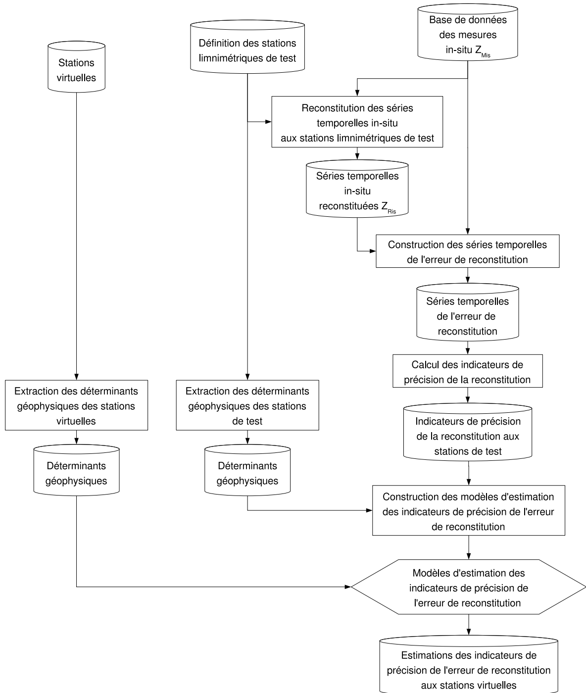
FIG. 6.9: Schéma détaillé de l'étape 5 de la Méthode Standard de Quantification de la Qualité des Produits Alti-Hydrologiques. L'estimation des indicateurs de précision de reconstitution se déroule en 2 phases parallèles comme l'illustre cette figure : les modèles multivariés sont construits à partir de l'erreur de reconstitution issue des stations limnimétriques de test et de leurs déterminants géophysiques. Les modèles sont ensuite employés en production pour estimer l'écart-type de l'erreur imputable à la méthode de reconstitution des séries temporelles in-situ. Enfin, cette erreur est retranchée par différence quadratique (cf. équation 6.18).
