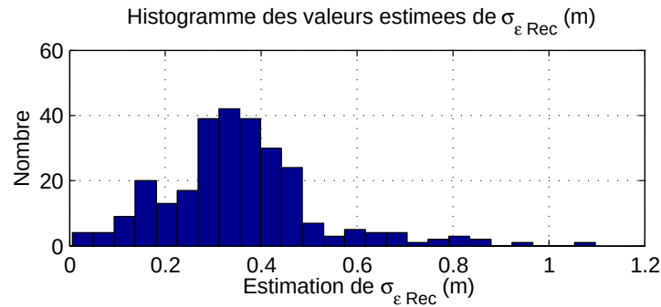
FIG. 6.8: Histogramme des valeurs de \hat{\sigma}_{\varepsilon_{Rec}} estimées pour les stations virtuelles.
