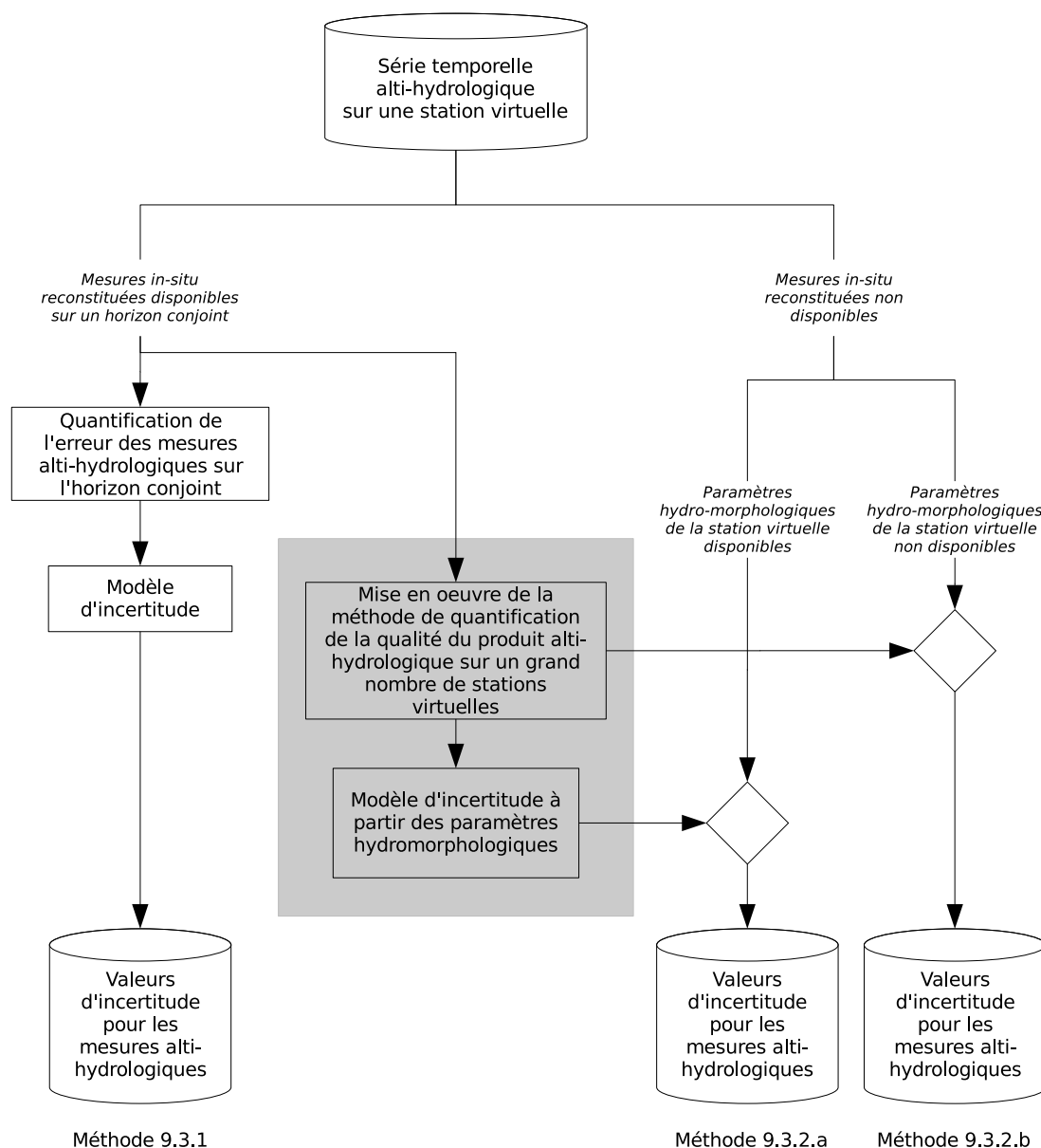
FIG. 8.11: Organigramme des méthodes de détermination de l'incertitude des mesures altimétriques, de gauche à droite : de la plus précise à la moins précise.
