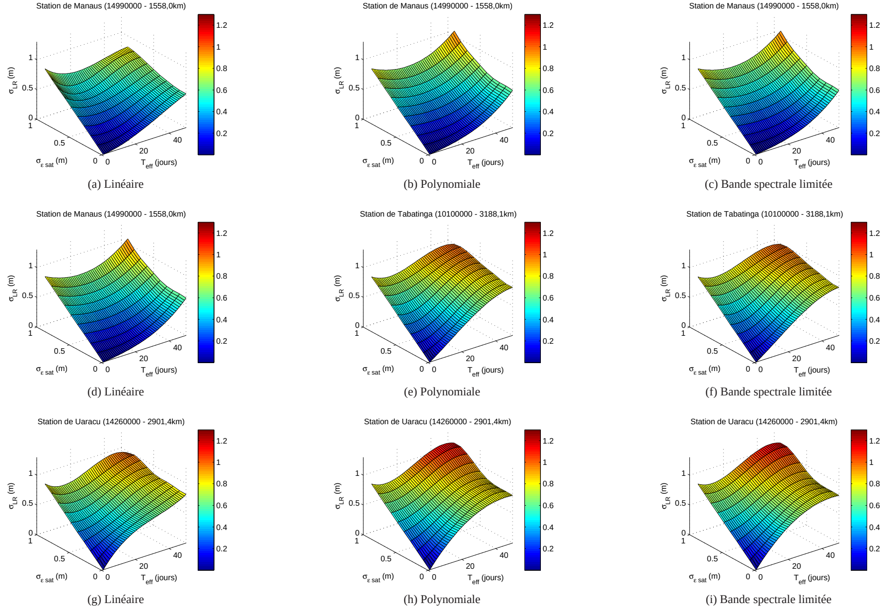
FIG. 9.7: Illustration des effets couplés, sur l'écart-type de l'erreur d'une série temporelle alti-hydrologique suréchantillonnée, d'une technique de suréchantillonnage, d'un bruit de mesure (gaussien centré) pour différentes valeurs de variance et d'un sous échantillonnage pour différentes périodes.
