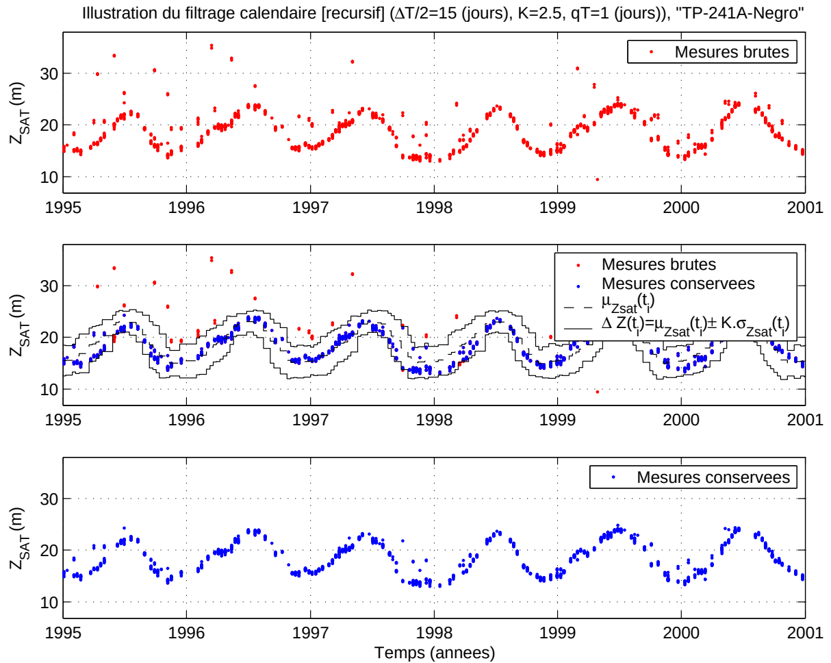
FIG. 3.11: Illustration du filtrage calendaire récursif sur la série temporelle de la station virtuelle « TP-241A-Negro », pour K = 2, 5 ; \Delta_T = 15 jours et qT = 1 jour. En haut : La série temporelle avec plusieurs mesures par passage contenant un certain nombre de mesures aberrantes. Au milieu : Les mesures en rouge sont en dehors des limites définies par l'intervalle mobile \Delta_Z(t_i) (lignes en trait plein noirs en haut et en bas) et sont retirées de la série temporelle résultante. En bas : la série temporelle. Ce filtre permet de retirer les mesures aberrantes comprises dans la dynamique générale de la série temporelle. Cette variante récursive permet de définir un gabarit de filtrage plus resserré sur les données.
