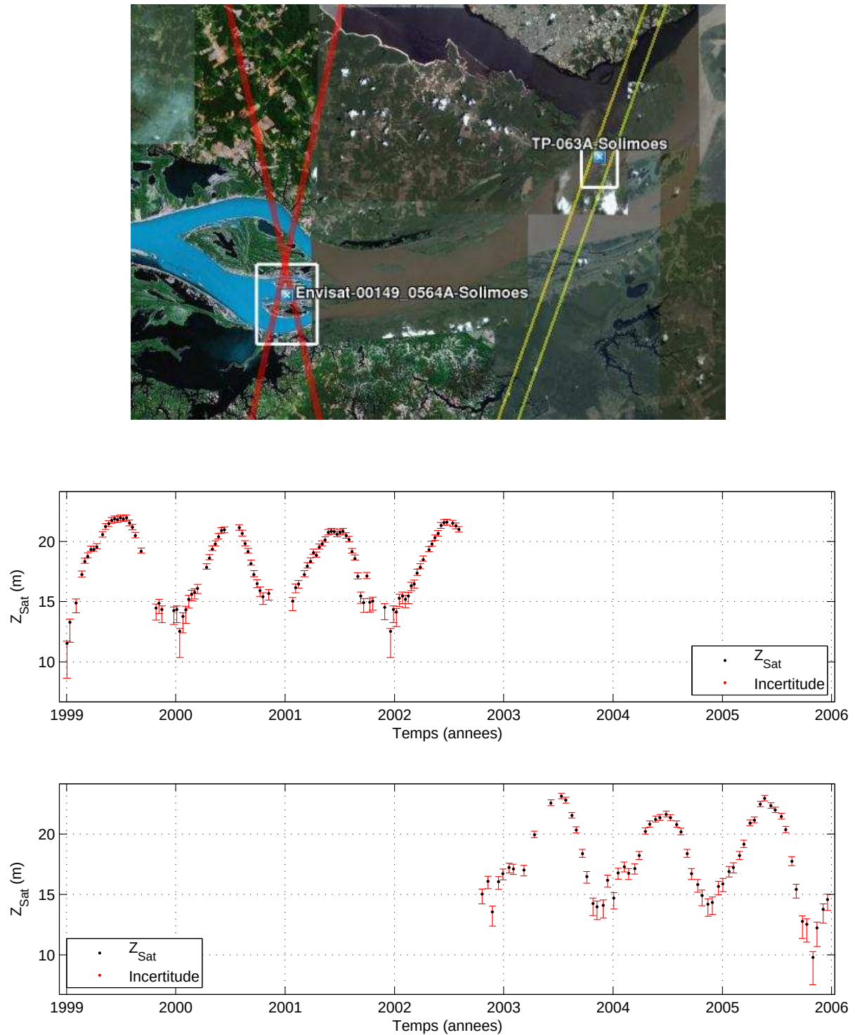
FIG. 9.10: Illustration de séries temporelles alti-hydrologiques avec valeurs d'incertitude associées.
