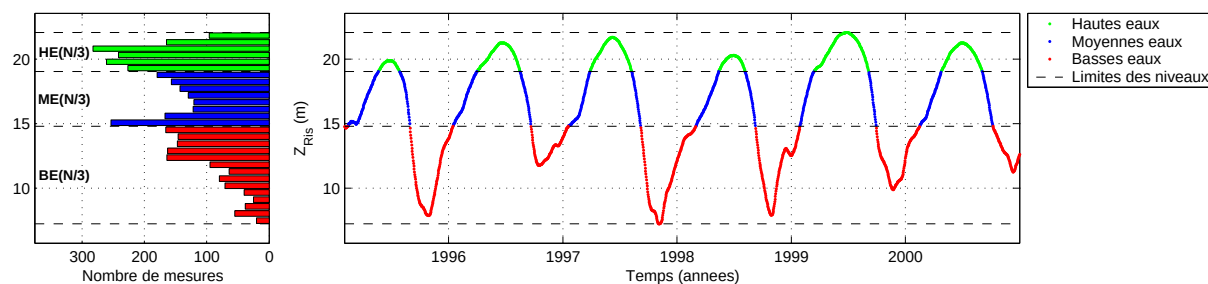
FIG. 5.9: Illustration du découpage en trois périodes hydrologiques de la dynamique de la série temporelle in-situ reconstituée à la station virtuelle « TP-063A-Solimoës » (série temporelle de droite). Le découpage est effectué de manière à ce que les trois périodes contiennent un nombre égal de mesures (à \pm une mesure près), soit N/3 mesures in-situ reconstituées par période si la série temporelle contient N mesures. Dans cet exemple, le découpage calculé sur l'horizon de la série temporelle in-situ reconstituée intégrale (mi-1995 à mi-2005) donne 1274 mesures/période (l'horizon temporel du limigramme a été tronqué pour améliorer la lisibilité de la figure). L'histogramme de gauche illustre ce découpage ainsi que la répartition des mesures in-situ reconstituées en fonction du niveau des eaux.
