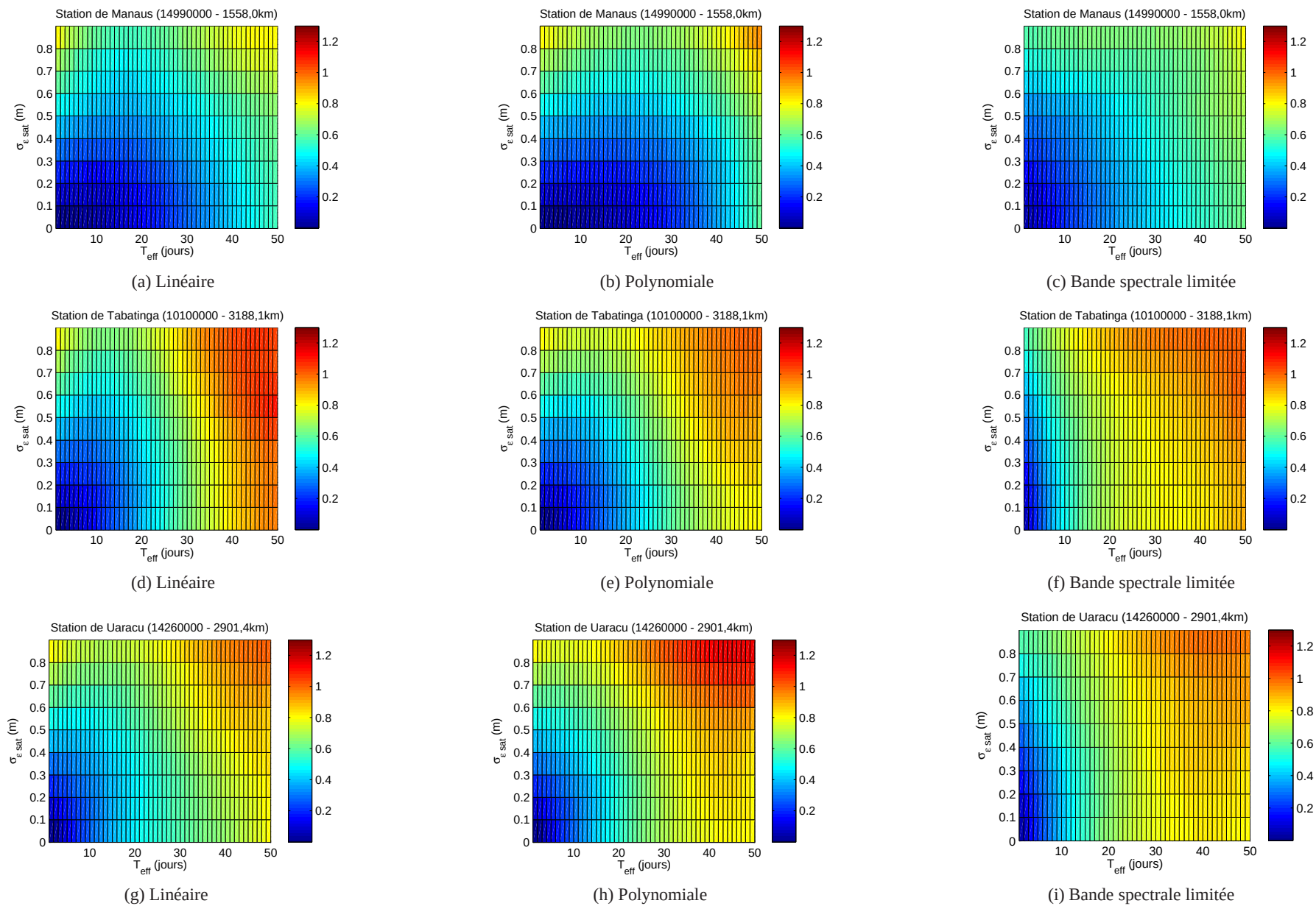
FIG. 9.6: Illustration des effets couplés, sur l'écart-type de l'erreur d'une série temporelle alti-hydrologique suréchantillonnée, d'une technique de suréchantillonnage, d'un bruit de mesure (gaussien centré) pour différentes valeurs de variance et d'un sous échantillonnage pour différentes périodes.
