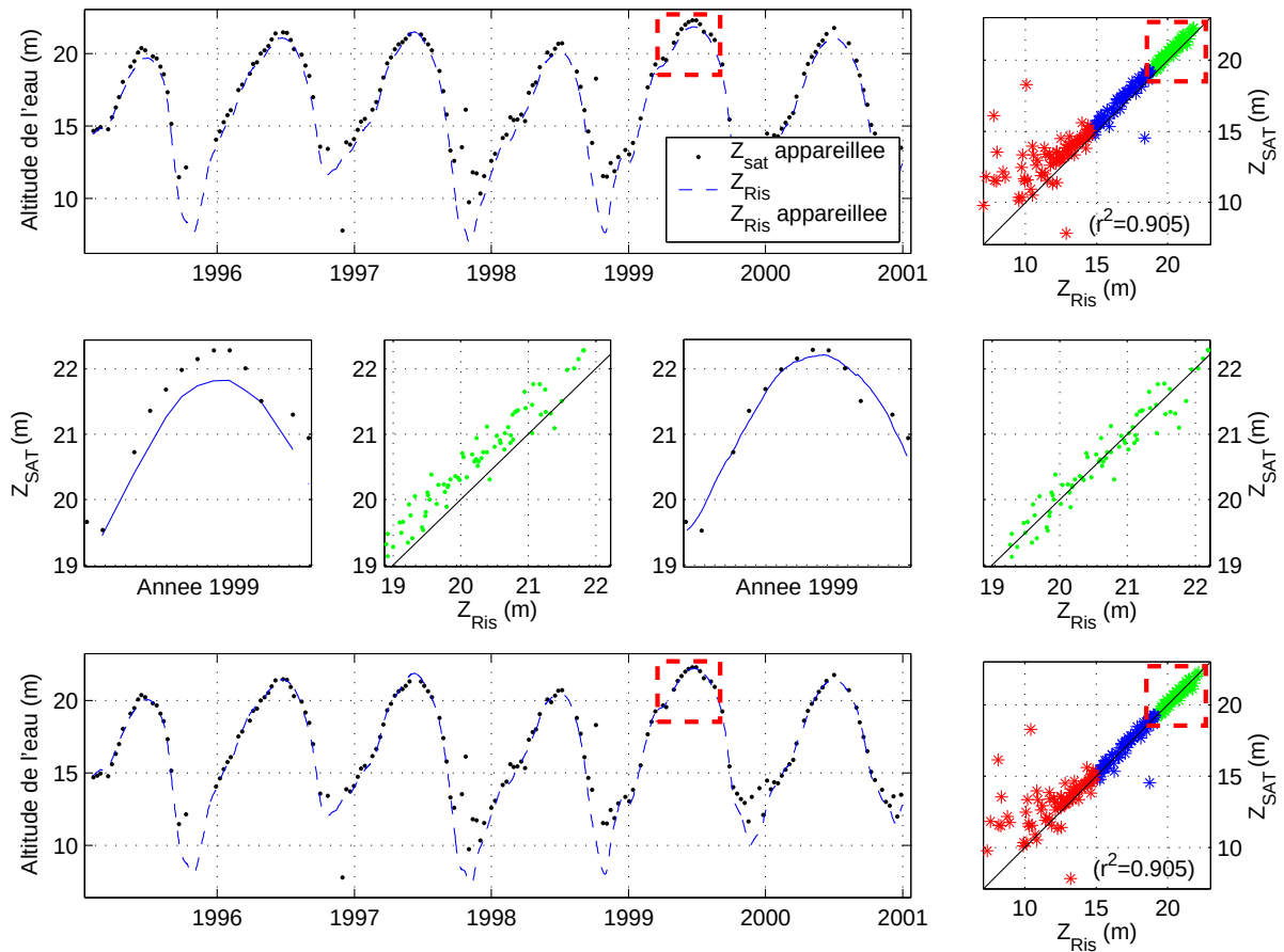
FIG. 6.11: Détail du processus de correction du biais systématique de hautes eaux entre une série temporelle alti-hydrologique et une série temporelle in-situ reconstituée pour la station virtuelle « TP-063A-Solimoès ». Haut gauche : les deux séries temporelles altimétrique et in-situ reconstituée. L'erreur des mesures est variable dans le temps : elle est corrélée aux variations du cycle hydrologique. La corrélation entre les mesures altimétriques et les mesures in-situ est meilleure lorsque le niveau des eaux est maximal (haut droite). Rangée du milieu, de gauche à droite : 1. zoom sur la période de hautes eaux de l'année 1999, le biais systématique apparaît nettement ; 2. zoom sur la droite de corrélation où le biais s'observe nettement ; 3. zoom sur la période de hautes eaux de l'année 1999, le biais systématique a été ajouté à la série temporelle in-situ reconstituée afin de faire correspondre au mieux les deux séries temporelles ; 4. zoom sur la droite de corrélation : les mesures sont parfaitement ajustées. Les lignes noires en diagonale illustrent les droites de corrélation idéales.
