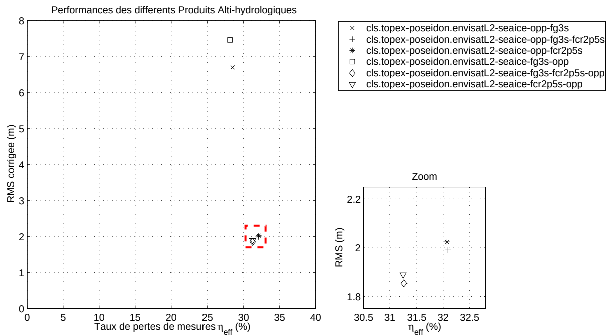
FIG. 7.19: Comparaison de performances des familles de produits alti-hydrologiques pour le groupe CLS/ENVISAT-L2/SeaIce (cf. table 7.16 (page 204) pour les valeurs numériques).
