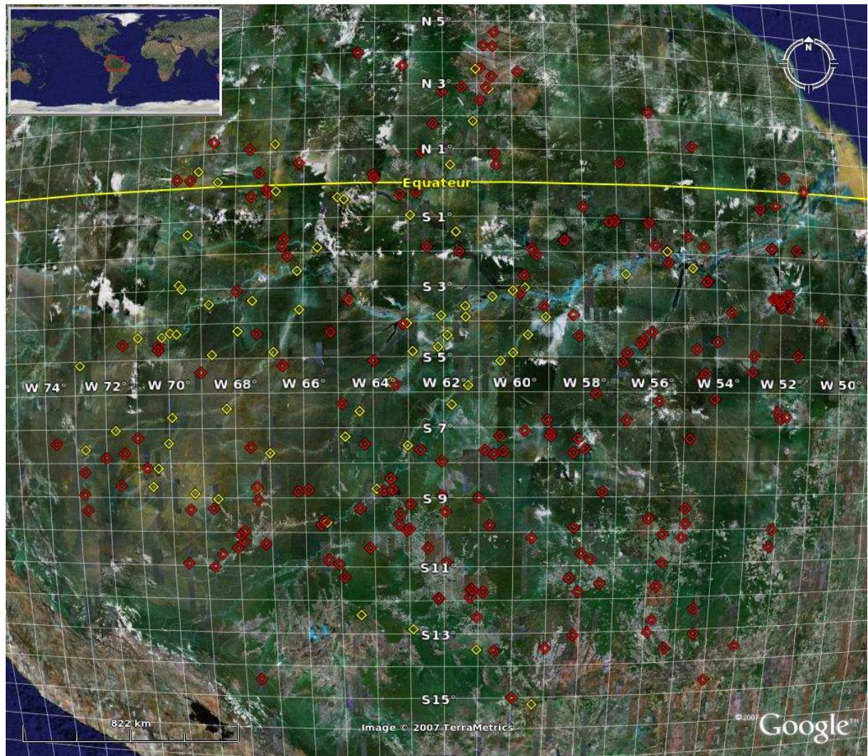
FIG. 2.6: Carte des 302 stations limnimétriques du bassin amazonien (Brésil) fournissant des mesures de niveaux des cours d'eau (losanges rouges). Seuls les losanges jaunes représentent des stations limnimétriques dont l'altitude du zéro de l'échelle est nivelé par rapport au niveau des moyen océans (98 en tout, voir [Kosuth et al., 2006]).
