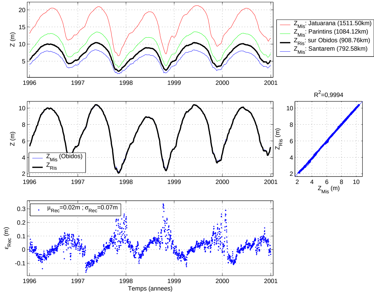
FIG. 6.1: Illustration de l'erreur de reconstitution sur la station limnimétrique d'Obidos située sur le fleuve Amazone. La série temporelle in-situ est reconstituée à partir des stations limnimétriques amont et aval de Jatuarana, Parintins et Santarem (chronogramme du haut). Sur le chronogramme du milieu, les deux séries temporelles mesurée ( Z_{Mis} en bleu) et reconstituée ( Z_{Ris} en noir) se confondent. L'erreur de reconstitution (série temporelle en bas) est caractérisée par un biais systématique \mu_{\varepsilon_{Rec}} = 0,02\text{m} et un écart-type \sigma_{\varepsilon_{Rec}} = 0,07\text{m} . Le graphe de droite illustre la corrélation entre les deux séries temporelles mesurée et reconstituée, cette corrélation est caractérisée par un coefficient r^2 = 0,9994 .
