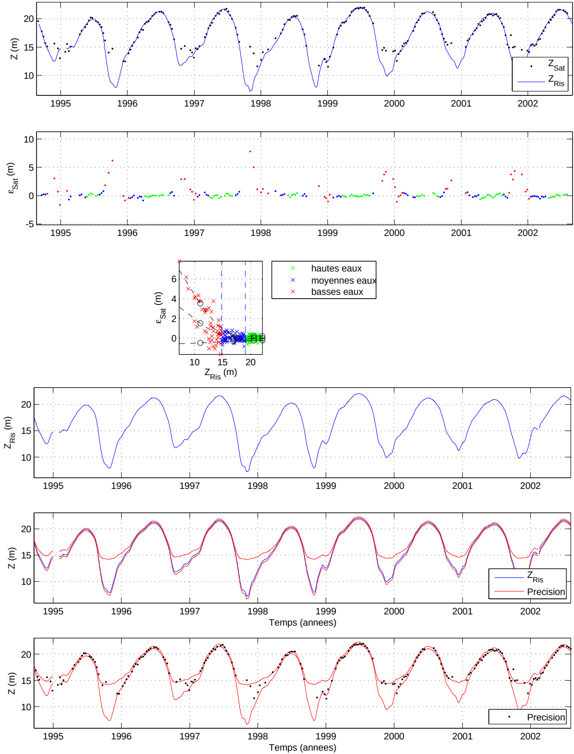
FIG. 8.9: Illustration de la construction d'un modèle de précision des mesures alti-hydrologiques et de son application. L'exemple s'appuie sur une station virtuelle à l'intersection entre la trace 63 de Topex/Poseidon et le fleuve Solimões. De haut en bas : (1) Les deux séries temporelles alti-hydrologique et in-situ reconstituée permettent de construire la série temporelle de l'erreur des mesures altimétriques (2). (3) Le modèle de précision \mathcal{M}_p ( \hat{\mu}_{\mathcal{M}_p} et \hat{\sigma}_{\mathcal{M}_p} ) est construit à partir des indicateurs de précision de l'erreur des mesures alti-hydrologiques par ajustement de courbes (noires en pointillé) sur les points de contrôle (ronds noirs). (4) Série temporelle in-situ reconstituée Z_{Ris} , à laquelle (5) on superpose les limites de précision [\hat{\mu}_{\mathcal{M}_p}(Z_{Ris}) \pm \hat{\sigma}_{\mathcal{M}_p}(Z_{Ris})] . (6) On vérifie que les mesures alti-hydrologiques sont, dans de bonnes proportions ( \sim 91\% des cas), situées dans l'intervalle de précision.
