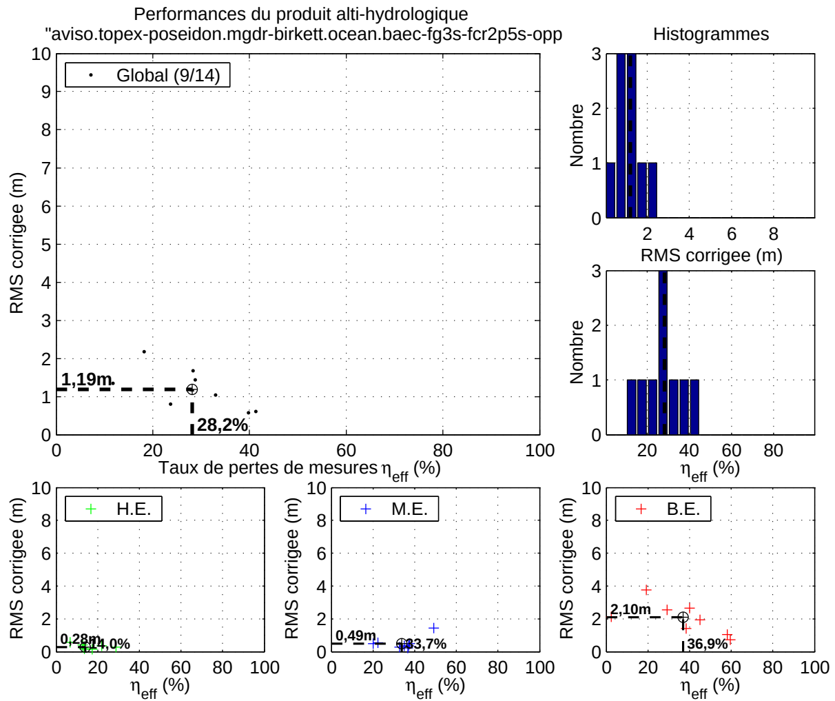
FIG. 7.12: Figure de synthèse pour le produit alti-hydrologique [~Birkett 2002] (Topex/Poseidon).
