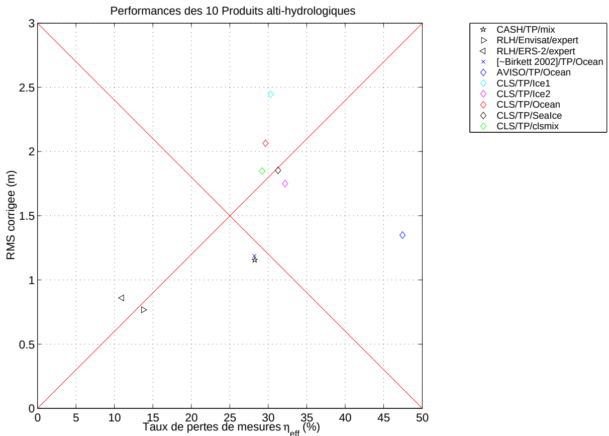
FIG. 7.23: Comparaison brute de la qualité de 10 produits alti-hydrologiques sur des jeux hétérogènes de stations virtuelles. Comme expliqué dans le texte, cette comparaison brute n'est pas pertinente (cf. 7.27 pour une comparaison pertinente).
