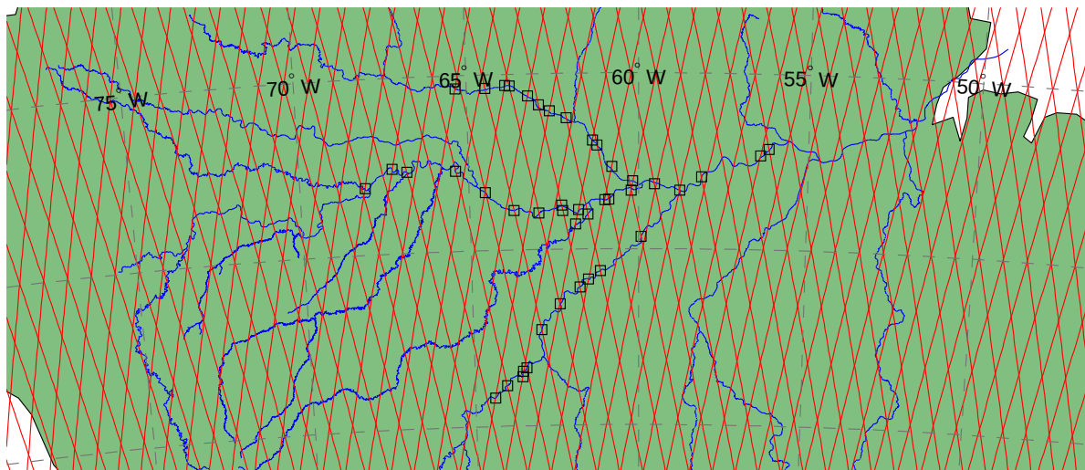
FIG. 7.6: Carte des 43 stations virtuelles ERS-2 (carrés noirs) définies sur quelques grands fleuves du bassin amazonien pour le produit alti-hydrologique RLH/ERS-2 aux intersections avec les traces de (traits rouges) de l'orbite à 35 jours de ERS-2 et ENVISAT (Projection cylindrique équidistante).
