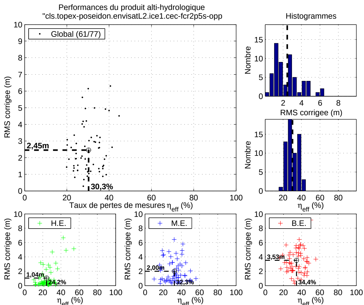
FIG. B.32: Figure de synthèse pour le produit alti-hydrologique « cls.topex-poseidon.envisatL2.ice1.cec-fcr2p5s-opp ».
