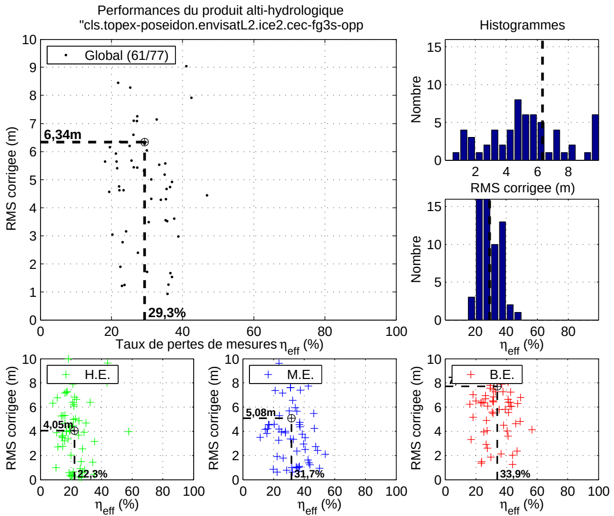
FIG. B.37: Figure de synthèse pour le produit alti-hydrologique « cls.topex-poseidon.envisatL2.ice2.cec-fg3s-opp ».
