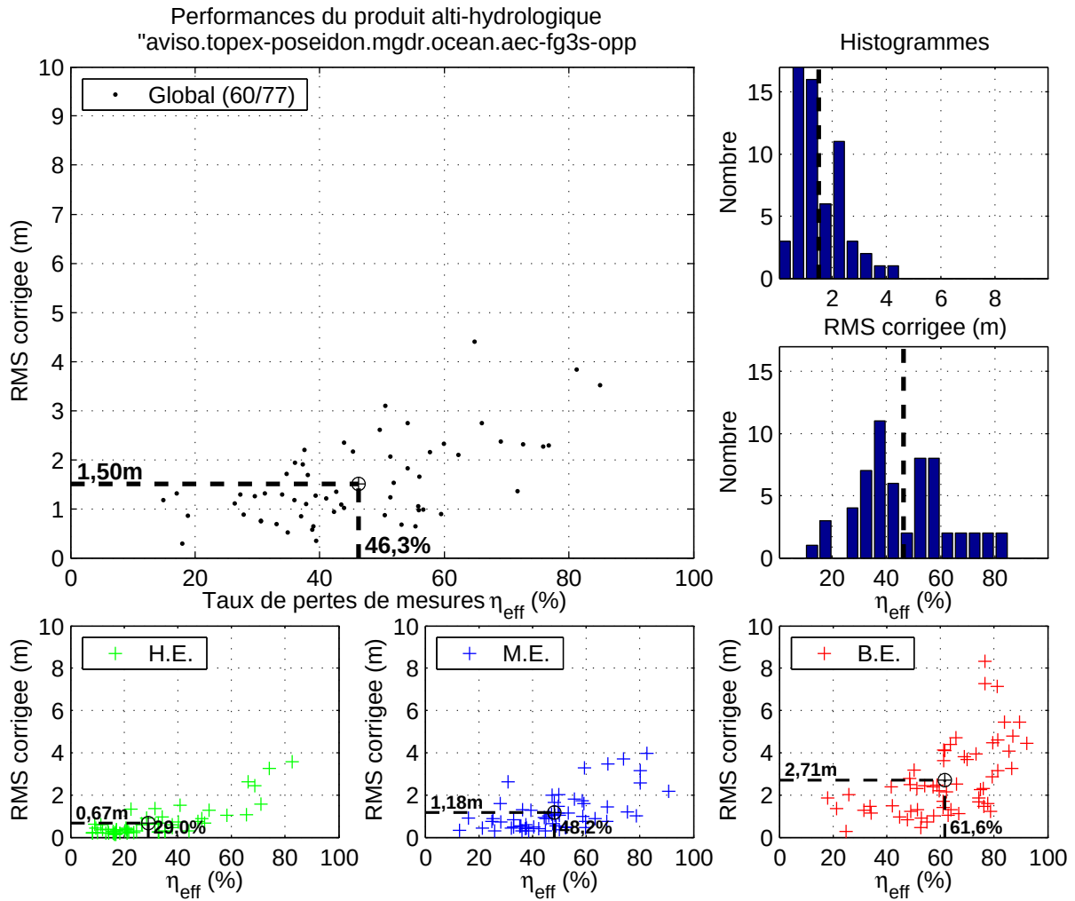
FIG. B.9: Figure de synthèse pour le produit alti-hydrologique « aviso.topex-poseidon.mgdr.ocean.aec-fg3s-opp ».
