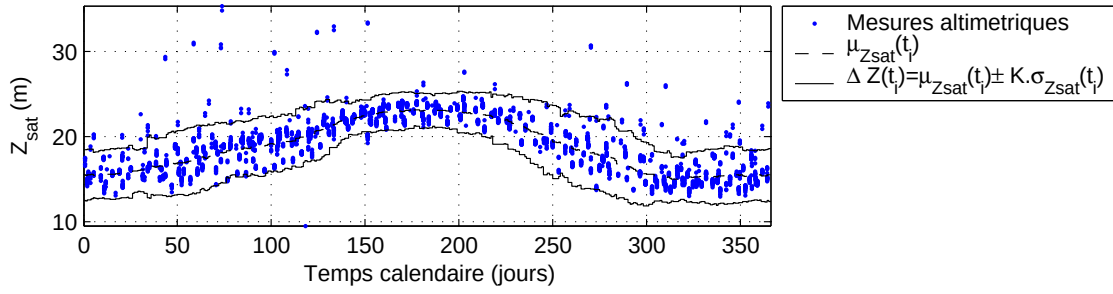
Illustration du gabarit du filtrage calendaire [récursif] ( \Delta T/2=15 (jours), K=2.5 , qT=1 (jours)), "TP-241A-Negro"
