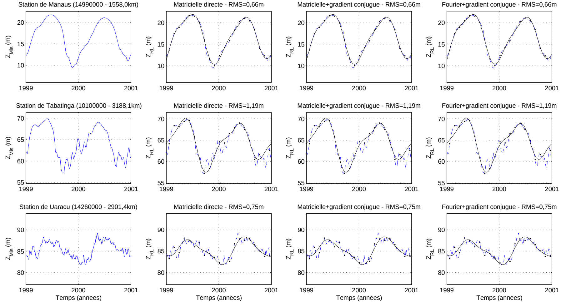
FIG. 9.4: Application de la méthode de suréchantillonnage par interpolation à « bande spectrale limitée » selon trois approches de résolution du système de l'équation (9.3). Afin d'estimer l'erreur induite par les méthodes de suréchantillonnage, on procède au sous-échantillonnage des séries temporelles mesurées in-situ (colonne de gauche) ; les échantillons résultants sont matérialisés par les points noirs. On tente ensuite de reconstituer les séries temporelles originales à l'aide de la technique d'interpolation à « bande spectrale limitée » en prenant en compte \frac{1}{4} de la bande spectrale à basse fréquence du signal sous-échantillonné. Dans ces trois exemples de résolution du système (9.3), les résultats sont strictement équivalents (valeurs RMS égales à 10^{-6} m près). Nous adoptons la méthode de résolution « matricielle direct » plus économe en temps de calcul.
