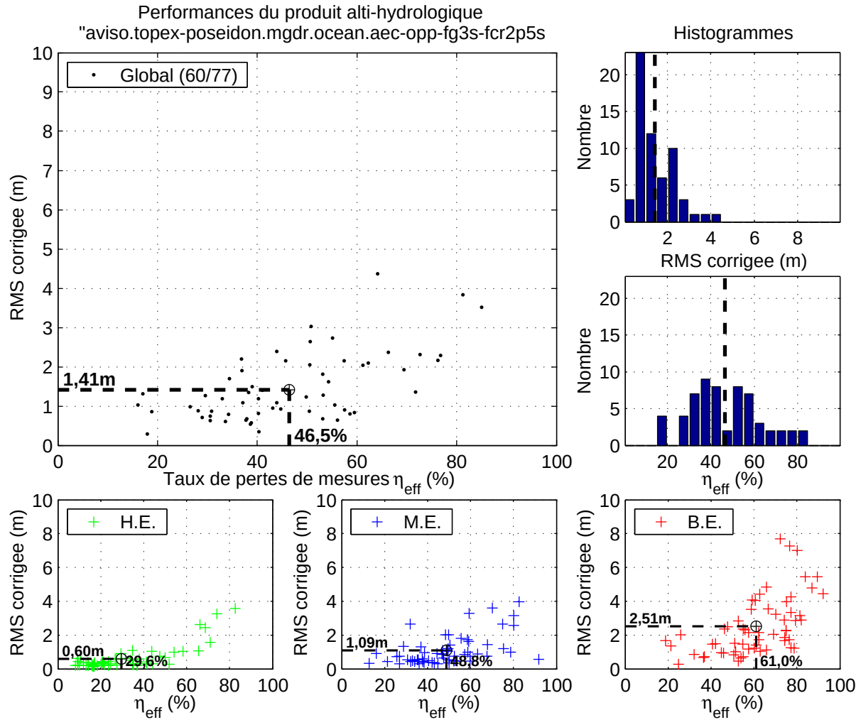
FIG. 7.8: Exemple de représentation graphique synthétique de la qualité du produit alti-hydrologique AVISO/M-GDR/aec-opp-fg3s-fcr2p5s (Topex/Poseidon) pour les 77 stations virtuelles définies par la première orbite de Topex/Poseidon sur le bassin amazonien ("aec-opp-fg3s-fcr2p5s" signifie que les étapes suivantes ont été appliquées au produit altimétrique AVISO/M-GDR : "critères de sélection AVISO" - "une mesure par passage" - "filtrage global ( K = 3 )" - "filtrage calendaire, variante récurrente K = 2, 5 ; \Delta T/2 = 15 jours").
