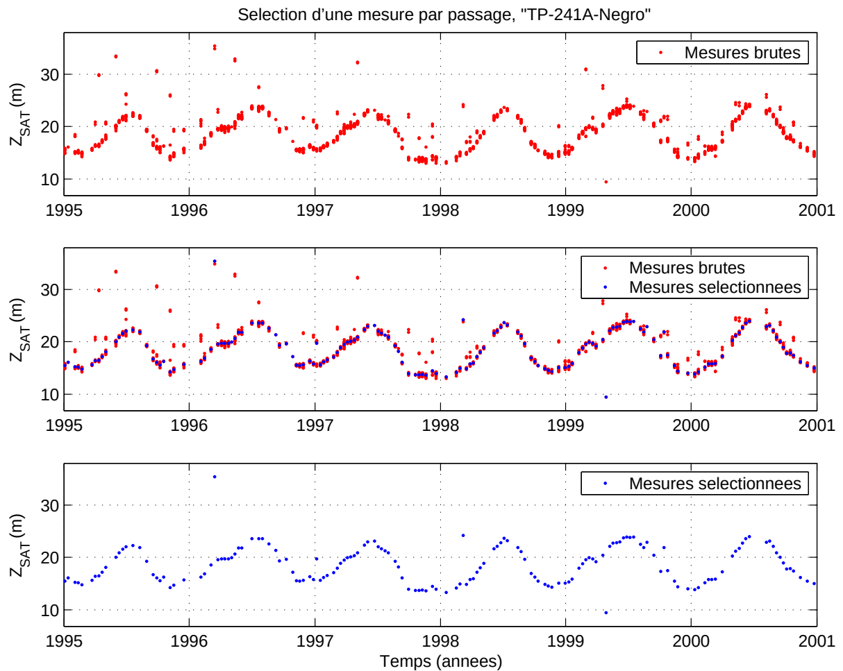
FIG. 3.6: Illustration du processus de sélection d'une mesure par passage du satellite pour la station virtuelle « TP-241A-Negro ». En haut : série temporelle brute où l'on peut observer les groupes de mesures collectées lors de chacun des passages du satellite à la station virtuelle. Au milieu : une comparaison entre les mesures brutes et les mesures sélectionnées. En bas : le résultat du processus de sélection d'une mesure représentative par passage du satellite. Le résultat est proche de celui qui pourrait être fourni par une technique de filtrage, mais laisse quand même quelques mesures aberrantes dans la série temporelle.
