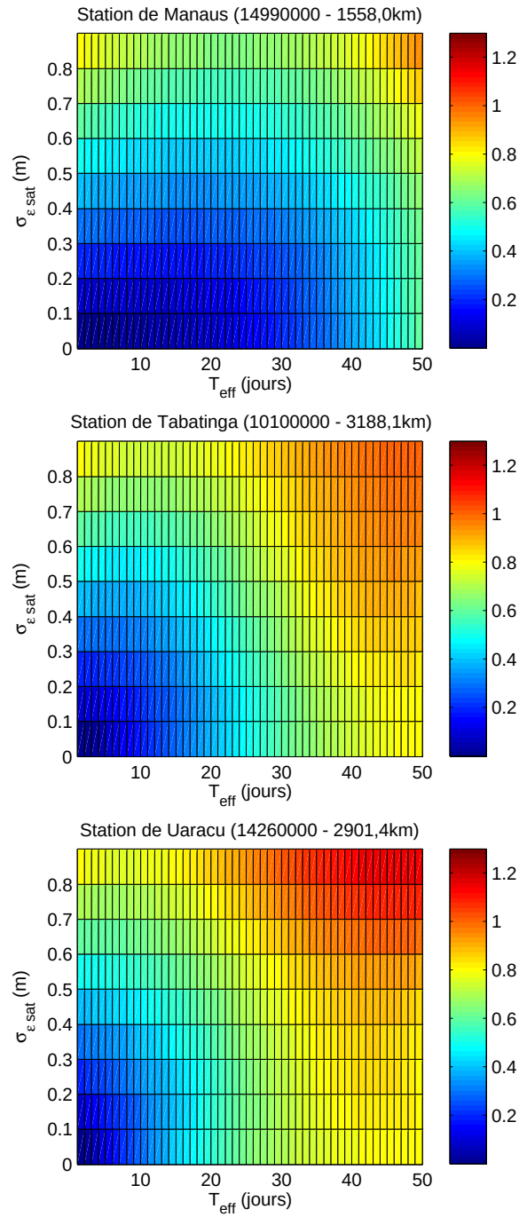
FIG. 9.8: Extrait de la figure 9.6 (colonne centrale) pour la méthode de suréchantillonnage « polynomiale de degré 4 avec contrainte d'énergie ».
