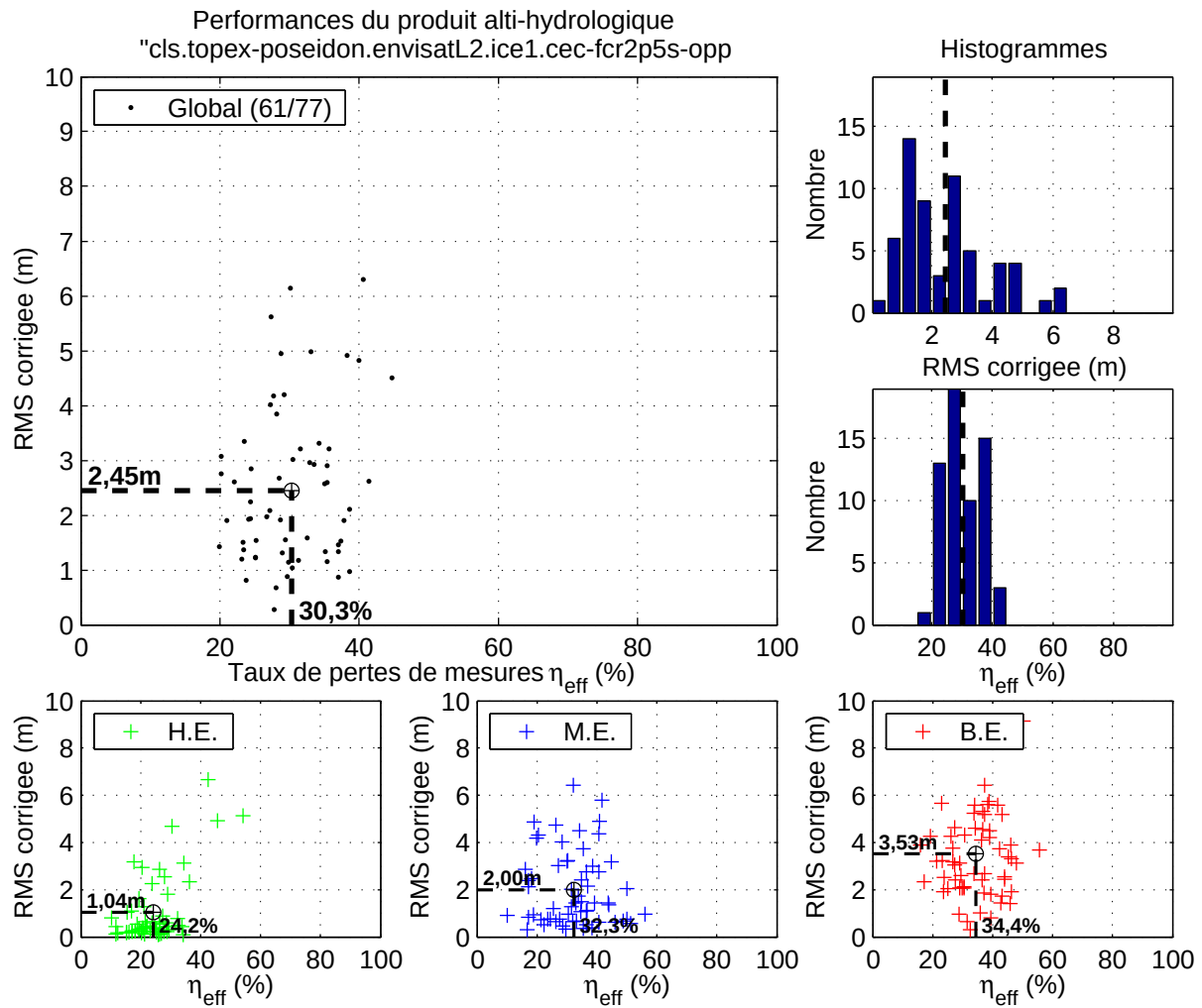
FIG. 7.14: Figure de synthèse pour le meilleur produit alti-hydrologique issu du groupe CLS ENVISAT-L2, retracker Ice1 (Topex/Poseidon).
