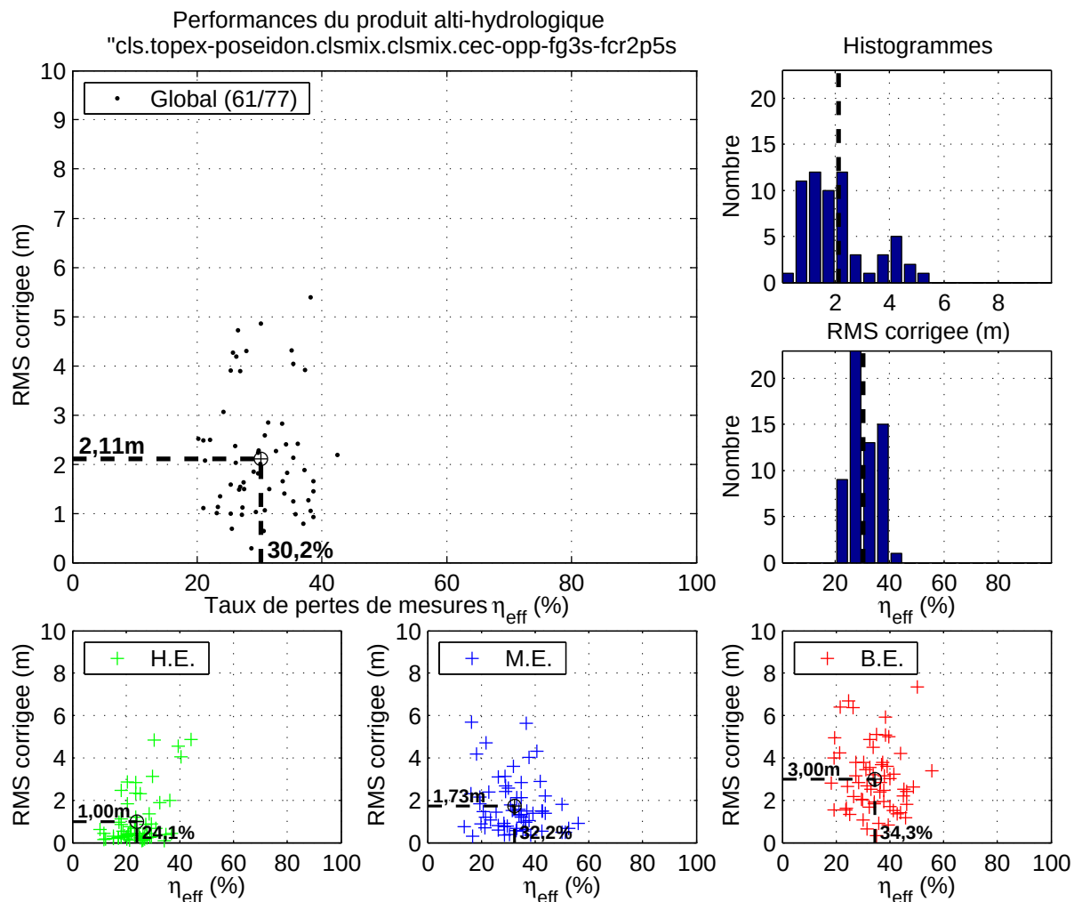
FIG. B.14: Figure de synthèse pour le produit alti-hydrologique « cls.topex-poseidon.clsmix.clsmix.cec-opp-fg3s-fcr2p5s ».
