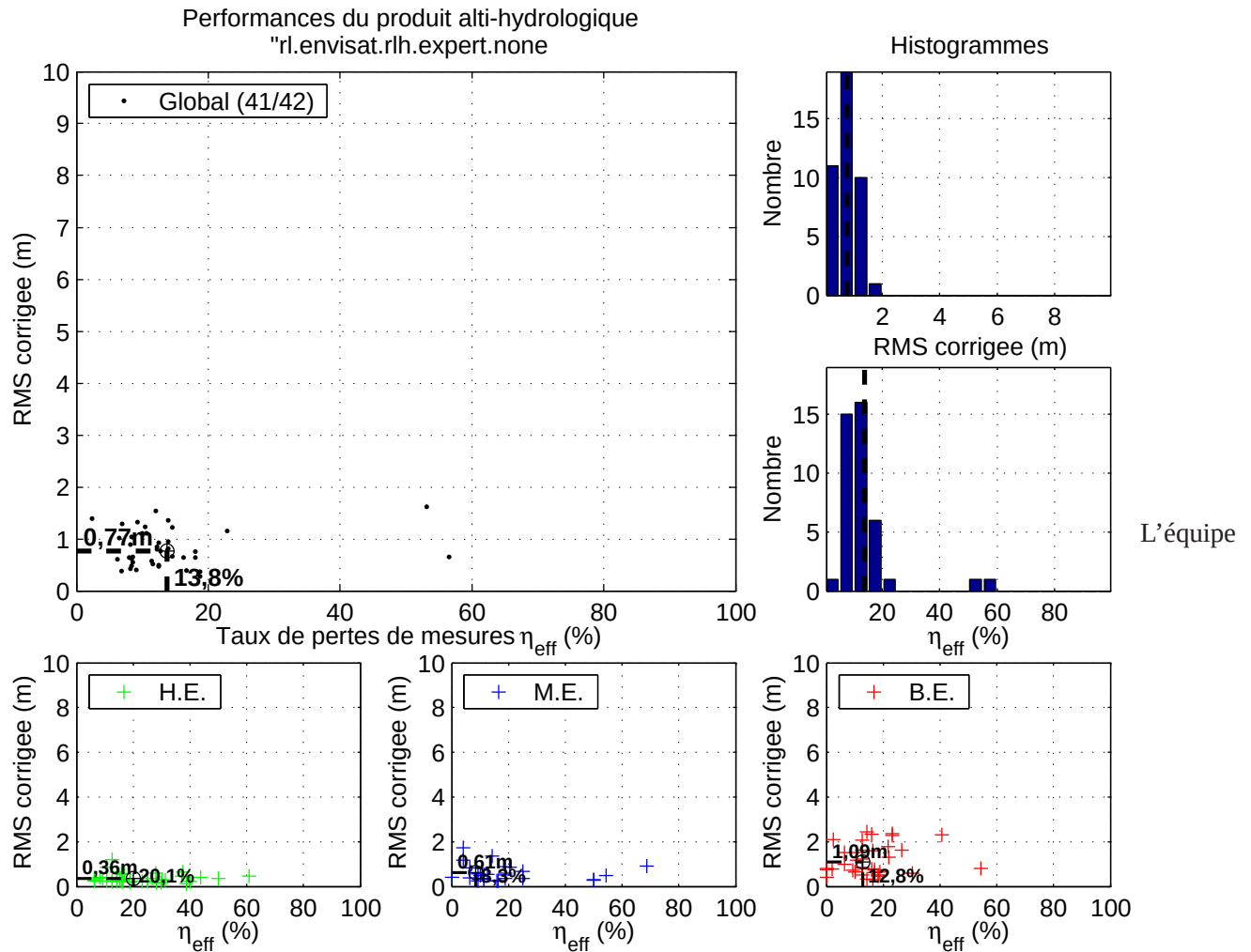
FIG. 7.10: Figure de synthèse pour le produit alti-hydrologique River &amp; Lake Hydrology/ENVISAT.
