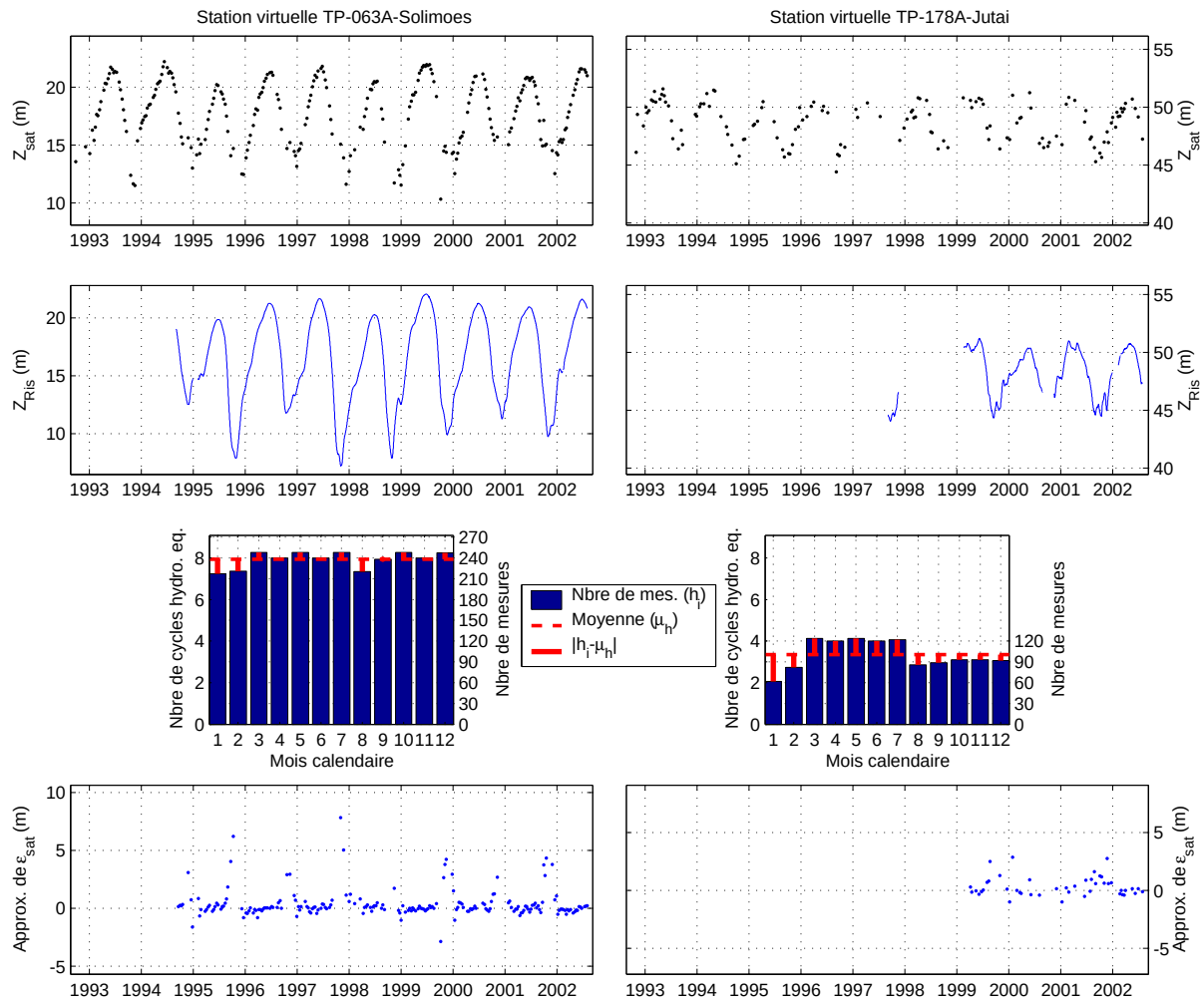
FIG. 5.8: Séries temporelles altimétriques, in-situ reconstituée et de l'erreur pour les stations virtuelles TP-063A-Solimoes (à gauche) et TP-178A-Jutai (à droite). Rangée du haut : séries temporelles altimétriques issues des stations virtuelles. Deuxième rangée : séries temporelles in-situ reconstituées. Troisième rangée : histogrammes de répartition des mesures in-situ reconstituées dans l'année calendaire (le minimum d'un histogramme correspond au nombre équivalent de cycles hydrologiques \tilde{N}_{CA} ). Dernière rangée : séries temporelles de l'erreur approximée des mesures altimétriques.
