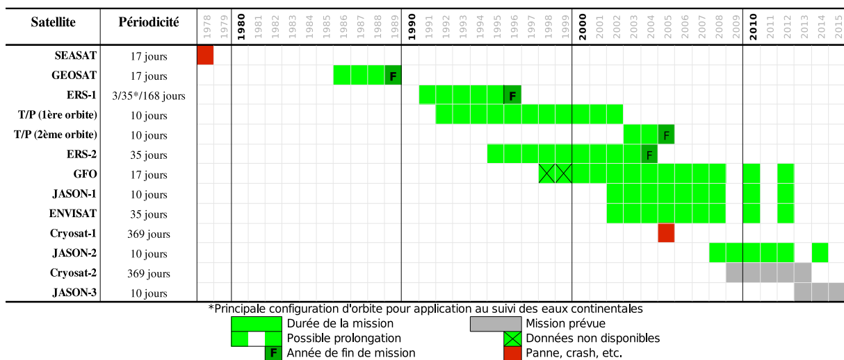
FIG. 1.1: Chronologie des principales missions altimétriques de 1978 à nos jours et à venir.
