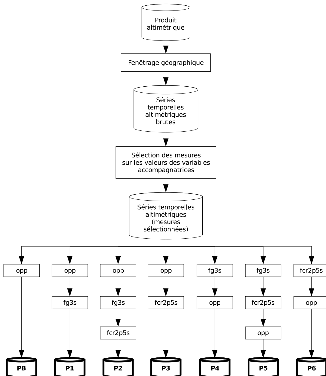
FIG. 7.1: Schéma des différentes chaînes de génération des produits alti-hydrologiques mises en œuvre sur les produits altimétriques AVISO et CLS.
