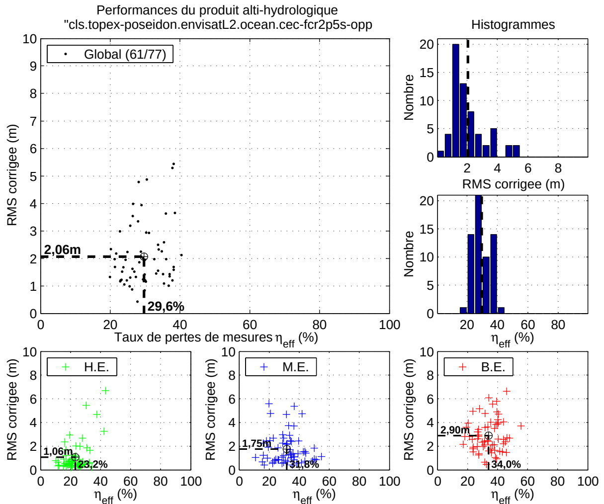
FIG. 7.16: Figure de synthèse pour le meilleur produit alti-hydrologique issu du groupe CLS ENVISAT-L2, retracker Ocean (Topex/Poseidon).
