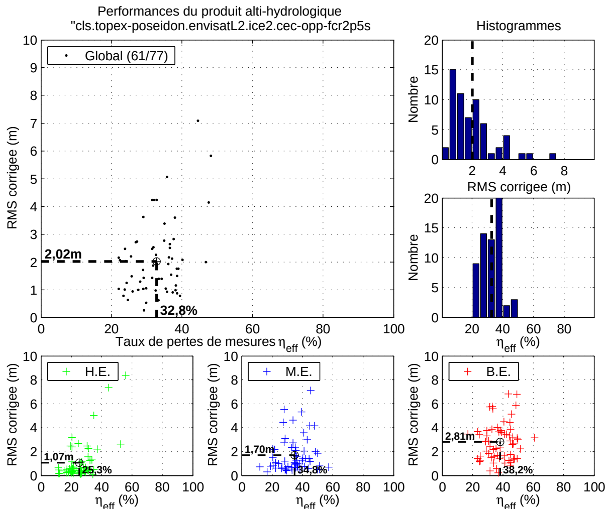
FIG. B.36: Figure de synthèse pour le produit alti-hydrologique « cls.topex-poseidon.envisatL2.ice2.cec-opp-fcr2p5s ».
