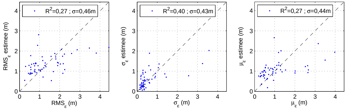
FIG. 8.2: Modèles globaux : Illustration de la sortie des modèles multivariables d'estimation des indicateurs de précision pour le produit alti-hydrologique AVISO/TP/M-GDR en fonction de leurs valeurs réelles. La ligne en pointillé illustre la droite de corrélation idéale. Les valeurs de \sigma présentées dans les graphiques sont les écart-types de l'erreur résiduelle des modèles.
