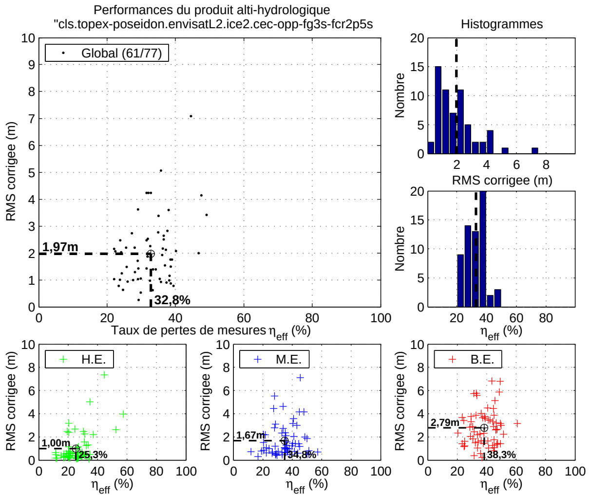
FIG. B.35: Figure de synthèse pour le produit alti-hydrologique « cls.topex-poseidon.envisatL2.ice2.cec-opp-fg3s-fcr2p5s ».
