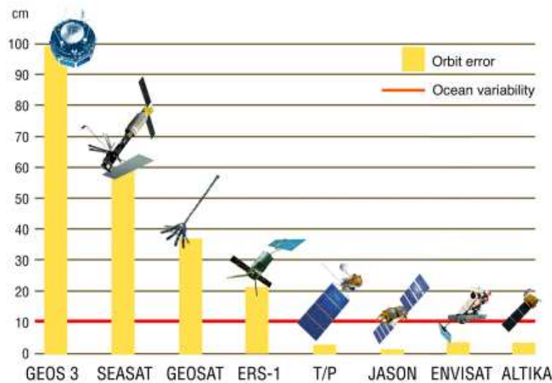
FIG. 1.3: Précision des orbites des principales missions satellitaires d'altimétrie radar nadir.
