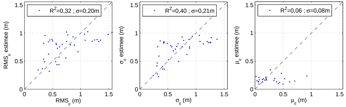
FIG. 8.6: Modèles globaux : Illustration de la sortie des modèles multivariables d'estimation des indicateurs de précision pour le produit alti-hydrologique RLH/ENVISAT en fonction de leurs valeurs réelles. La ligne en pointillé illustre la droite de corrélation idéale. Les valeurs de \sigma présentées dans les graphiques sont les écart-types de l'erreur résiduelle des modèles.
