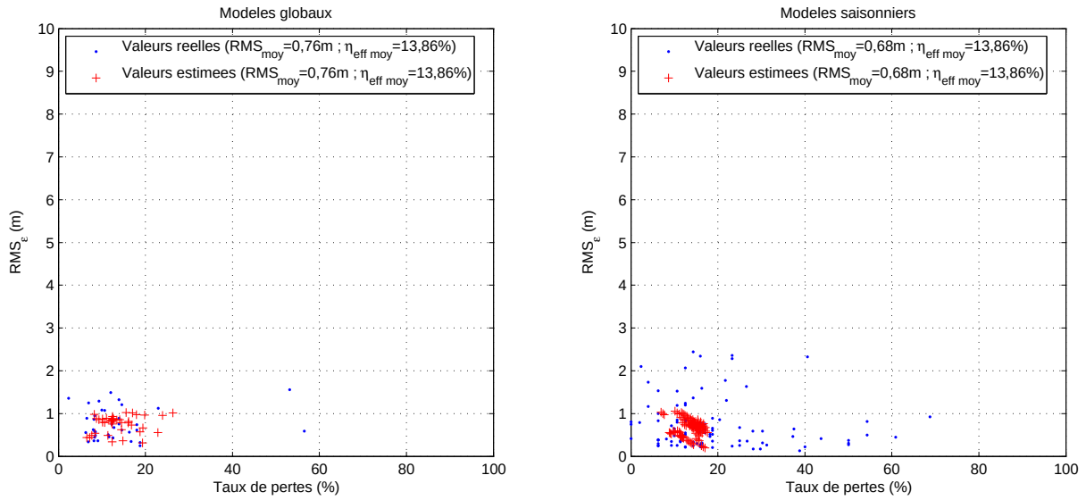
FIG. 8.8: Comparaison entre les valeurs réelles des indicateurs de qualité RMS et \eta_{eff} du produit alti-hydrologique RLH/ENVISAT aux valeurs issues des modèles globaux et saisonniers.
