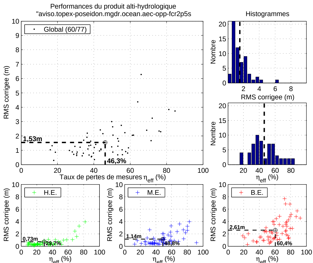
FIG. B.8: Figure de synthèse pour le produit alti-hydrologique « aviso.topex-poseidon.mgdr.ocean.aec-opp-fcr2p5s ».
