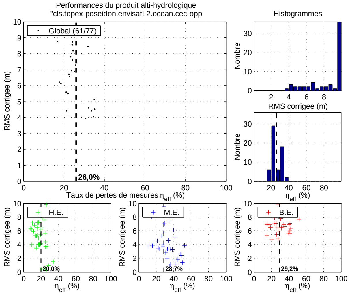
FIG. B.19: Figure de synthèse pour le produit alti-hydrologique « cls.topex-poseidon.envisatL2.ocean.cec-opp ».
