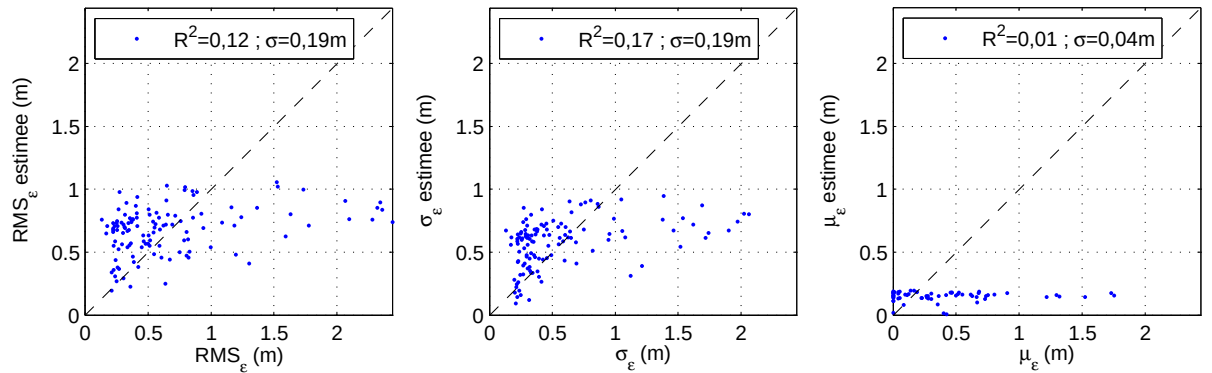
FIG. 8.7: Modèles saisonniers : Illustration de la sortie des modèles multivariables d'estimation des indicateurs de précision pour le produit alti-hydrologique RLH/ENVISAT en fonction de leurs valeurs réelles. La ligne en pointillé illustre la droite de corrélation idéale. Les valeurs de \sigma présentées dans les graphiques sont les écart-types de l'erreur résiduelle des modèles.
