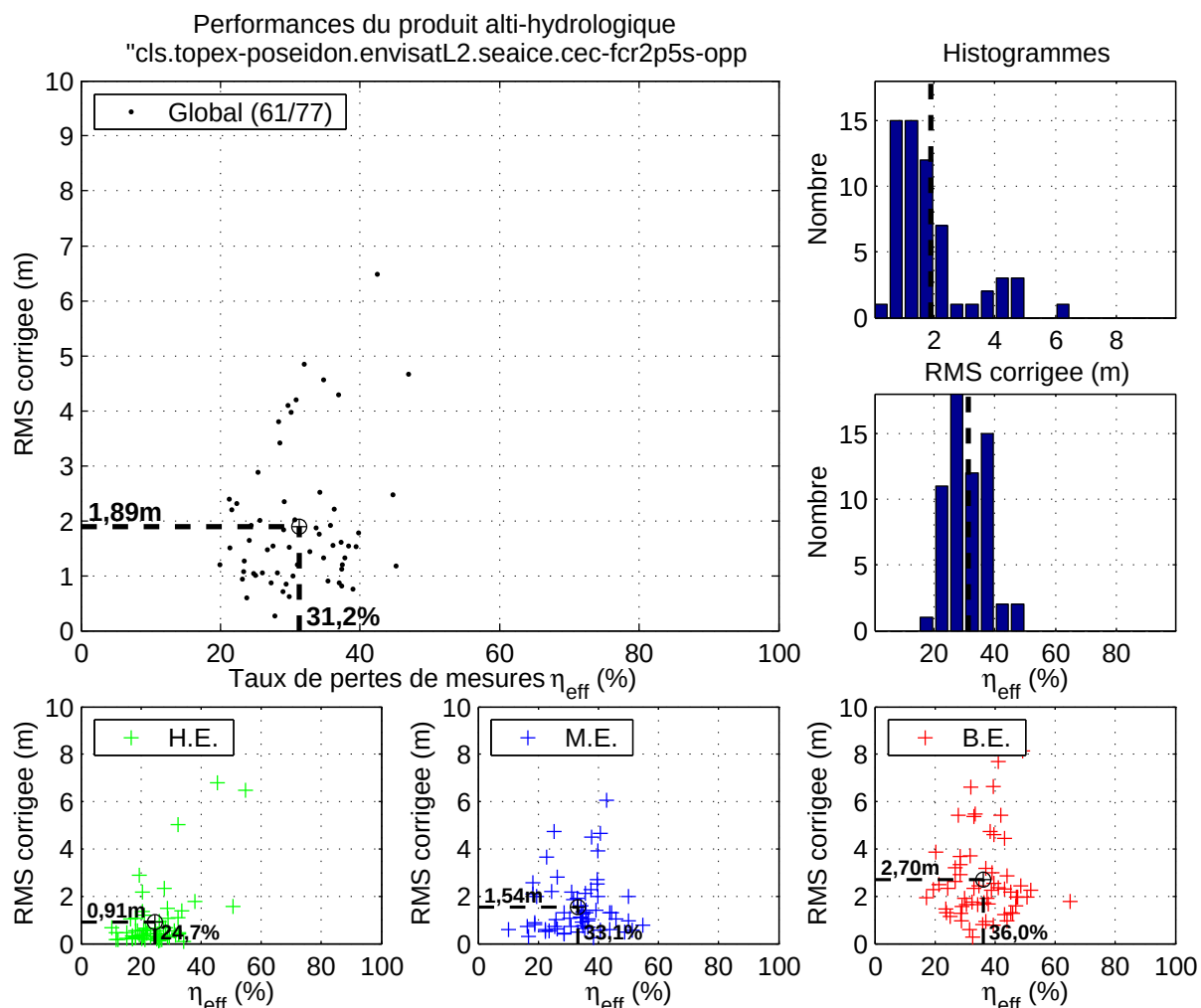
FIG. B.46: Figure de synthèse pour le produit alti-hydrologique « cls.topex-poseidon.envisatL2.seaice.cec-fcr2p5s-opp ».
