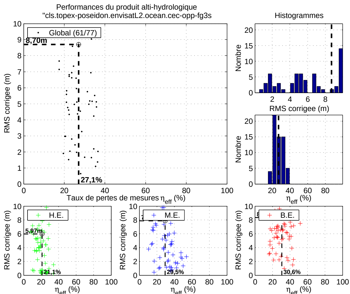
FIG. B.20: Figure de synthèse pour le produit alti-hydrologique « cls.topex-poseidon.envisatL2.ocean.cec-opp-fg3s ».
