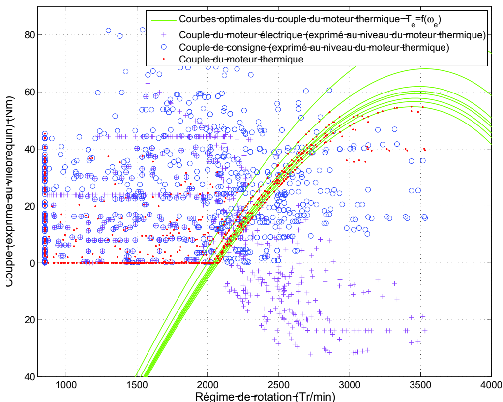
FIG. 3.8: Couple de consigne, couple du moteur électrique (ramené au niveau du moteur thermique) et couple du moteur thermique en fonction du régime. / Faisceaux de courbes représentant les points de fonctionnement optimaux du moteur thermique pour le véhicule de référence sur le cycle Artemis.
