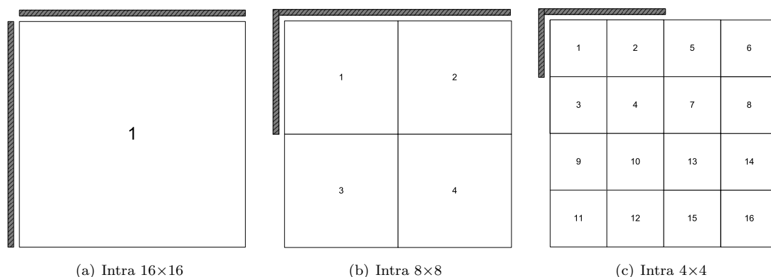
FIGURE 1.3 – Partitionnements de l’Intra de la norme H.264/AVC. Le signal de référence pour le premier bloc est représenté en gris. Les numéros à l’intérieur des blocs correspondent à l’ordre de parcours des partitionnements.
