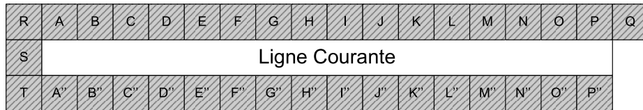
FIGURE 6.4 – Pixels du signal de référence utilisés pour le calcul des prédicteurs du partitionnement Ligne pour le parcours bidirectionnel dans le cas des partitions utilisant les partitions Par_i^B .
